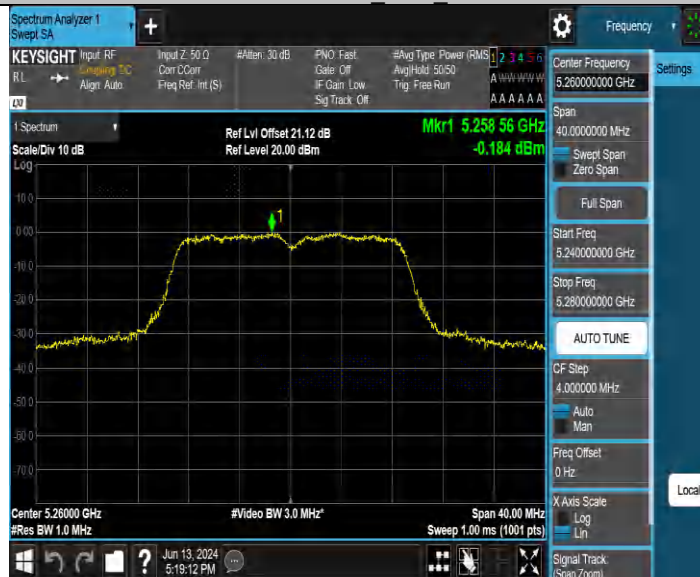
11AC20MIMO_Ant3 5260
