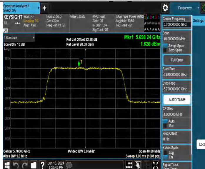
11AC20MIMO_Ant3 5700
