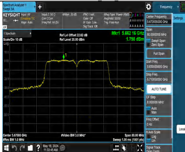
11AC40MIMO_Ant4 5670
