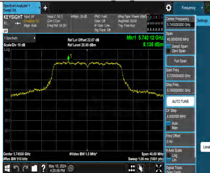
11AC20MIMO_Ant4 5745
