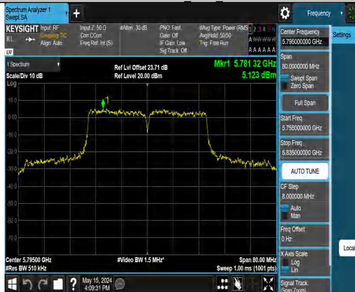
11N40MIMO Ant4 5795
