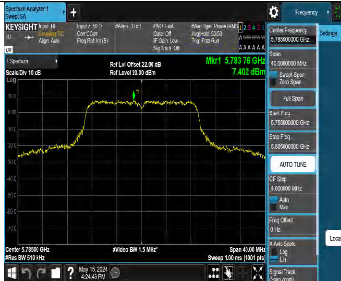
11AC20MIMO_Ant4_5785
