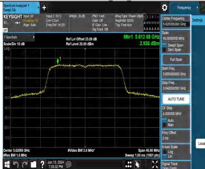
11AC20MIMO_Ant2_5620
