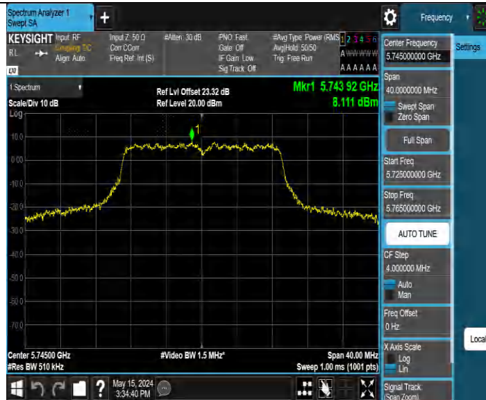
11N20MIMO Ant3 5745
