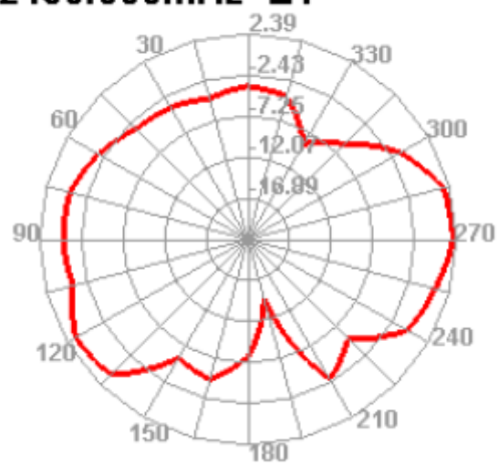
2450.000MHz E1
