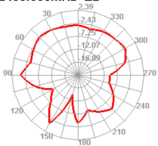
2450.000MHz E2
