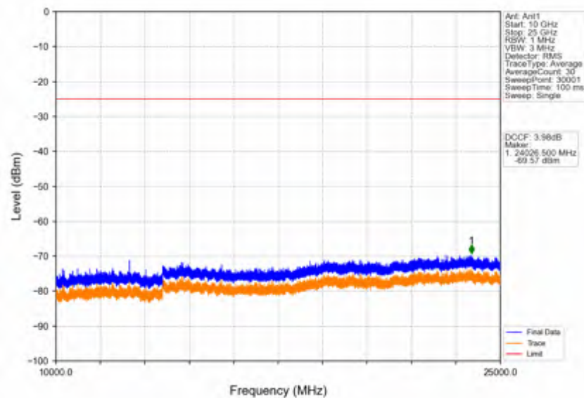
Band41 10MHz 64QAM LCH 2501MHz RB 1 0 NTNV
