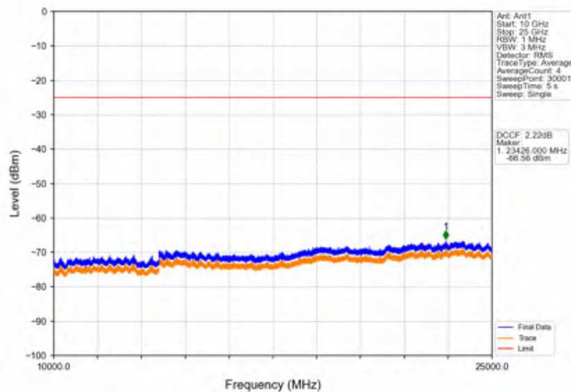
Band38 20MHz 16QAM LCH 2580MHz RB 1 0 NTNV
