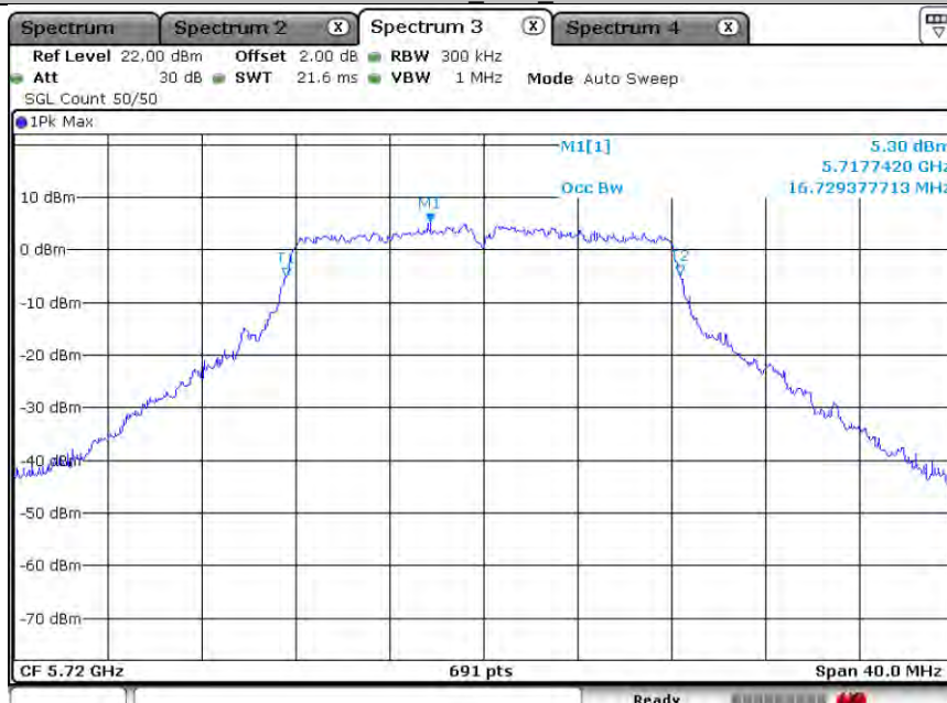
11A-CDD Ant1 5720
