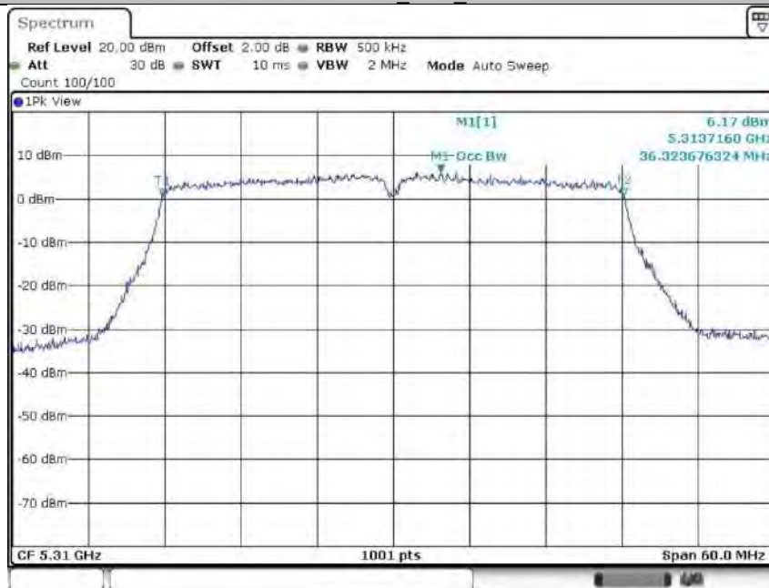
11N40MIMO_Ant2_5310
