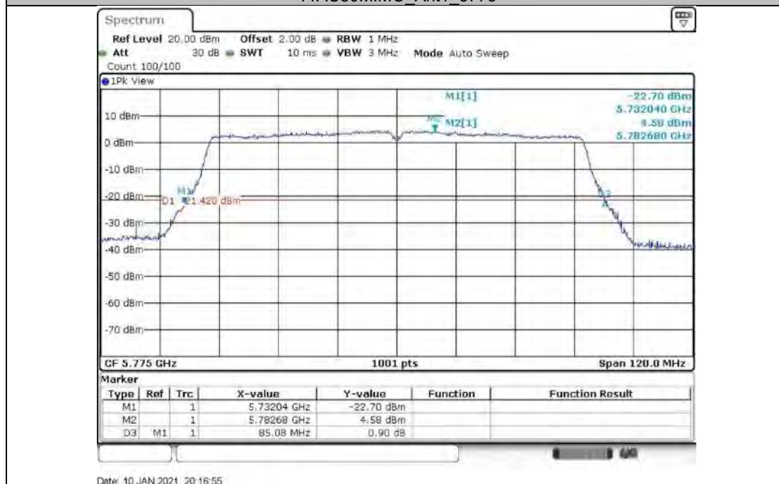
11AC80MIMO_Ant1_5775
