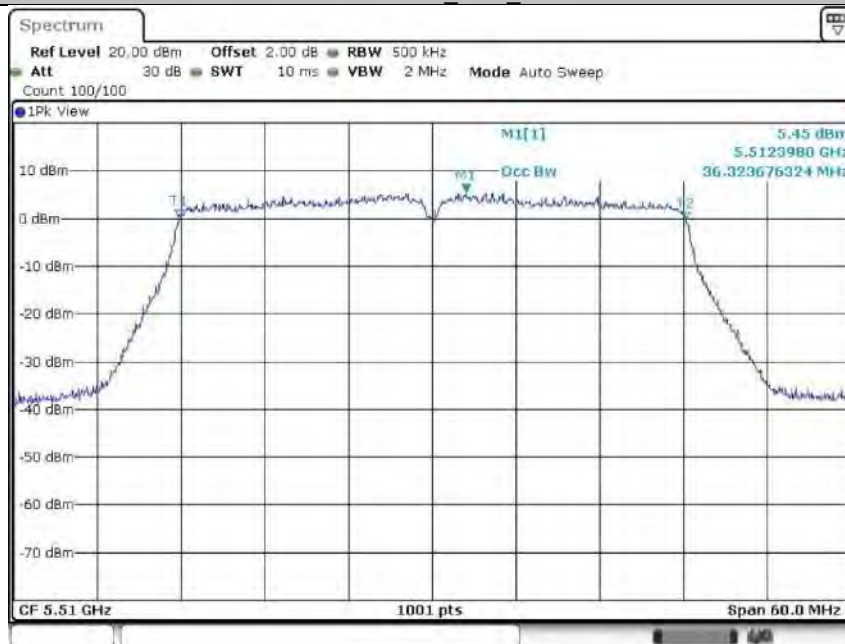
11AC40MIMO_Ant2_5510
