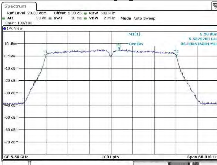
11AC40MIMO_Ant1_5550
