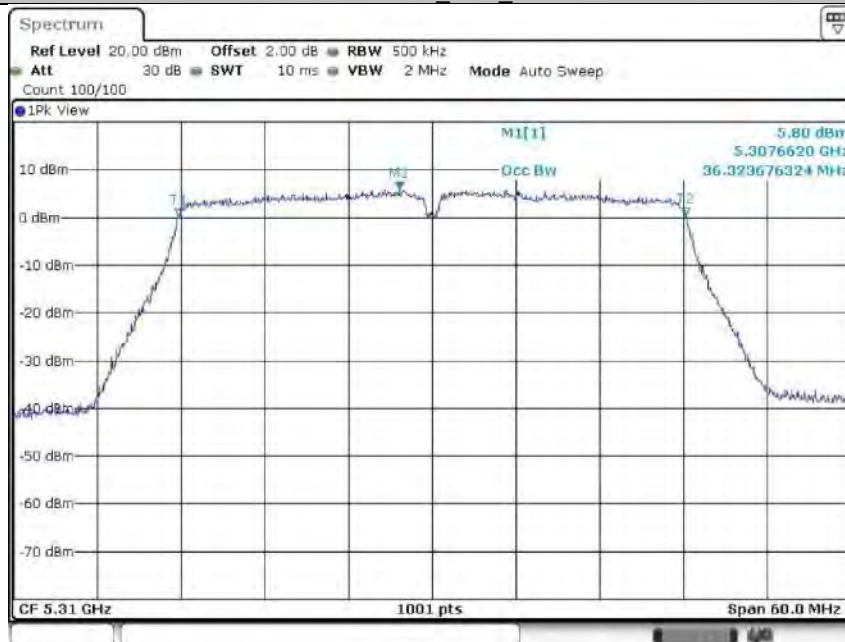
11N40MIMO_Ant1_5310
