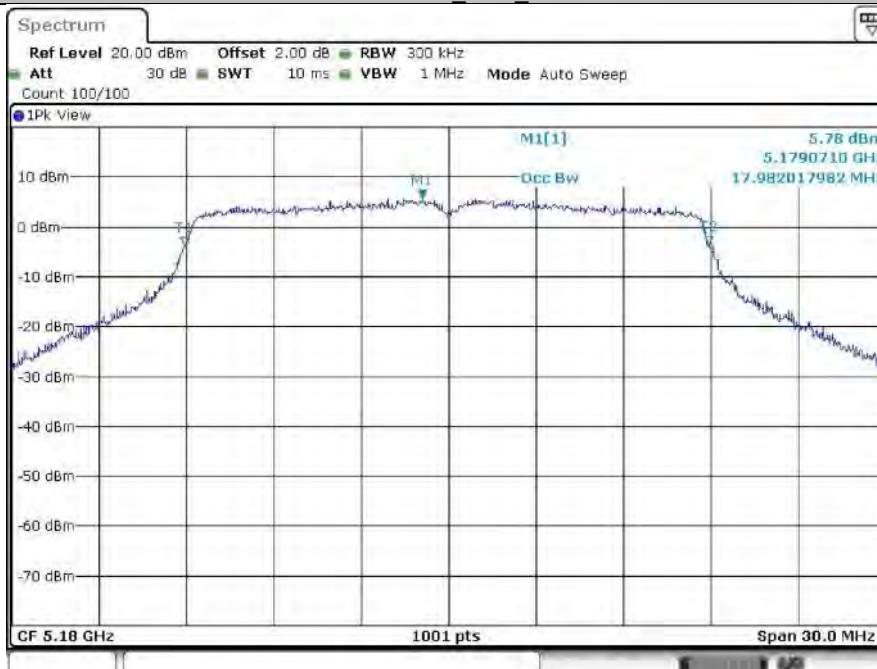
11N20MIMO Ant1 5180
