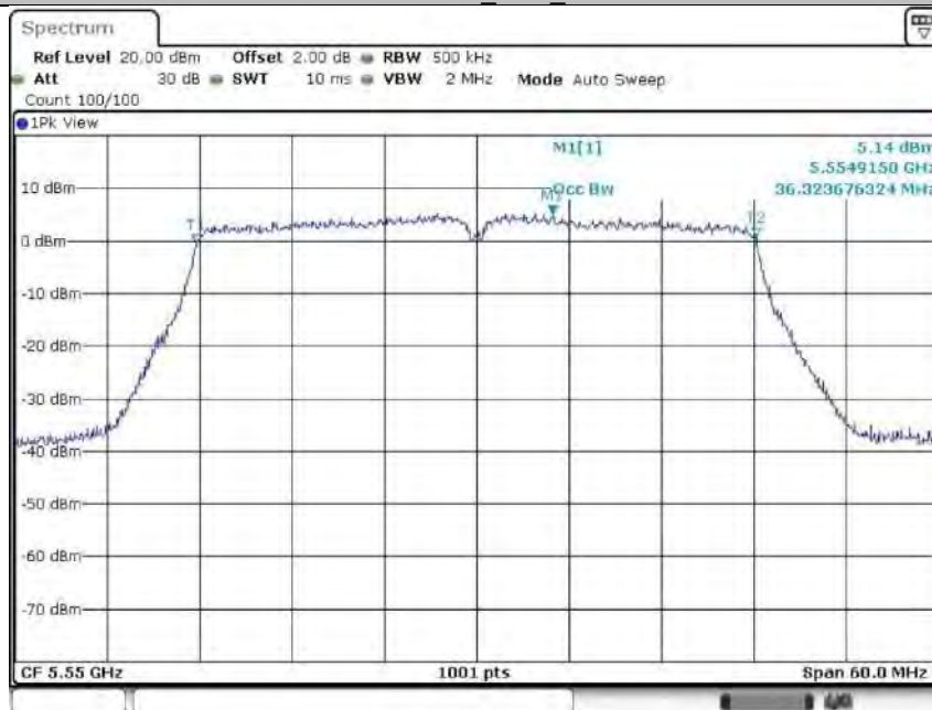
11N40MIMO_Ant2_5550
