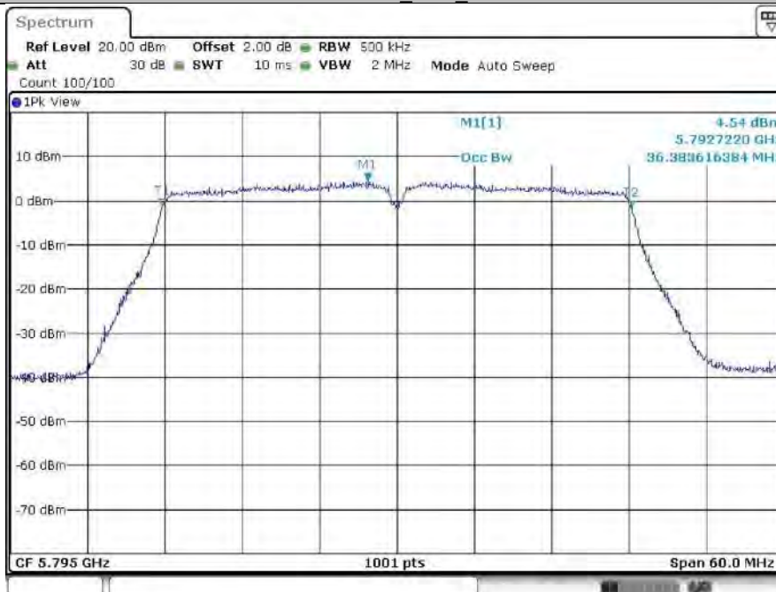
11N40MIMO Ant1 5795
