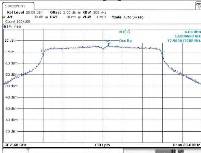
11N20SISO_Ant2_5580
