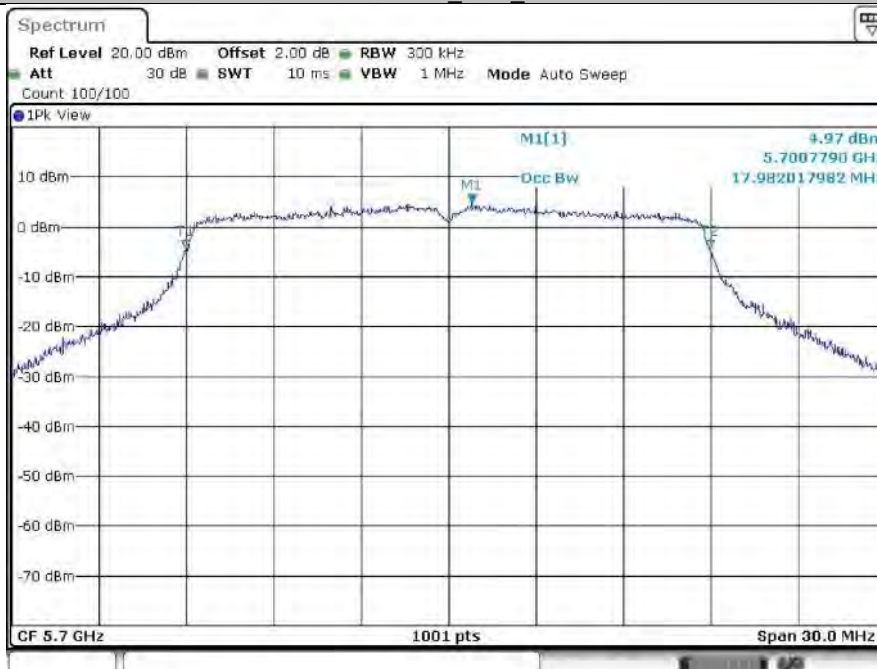
11N20SISO_Ant1_5700
