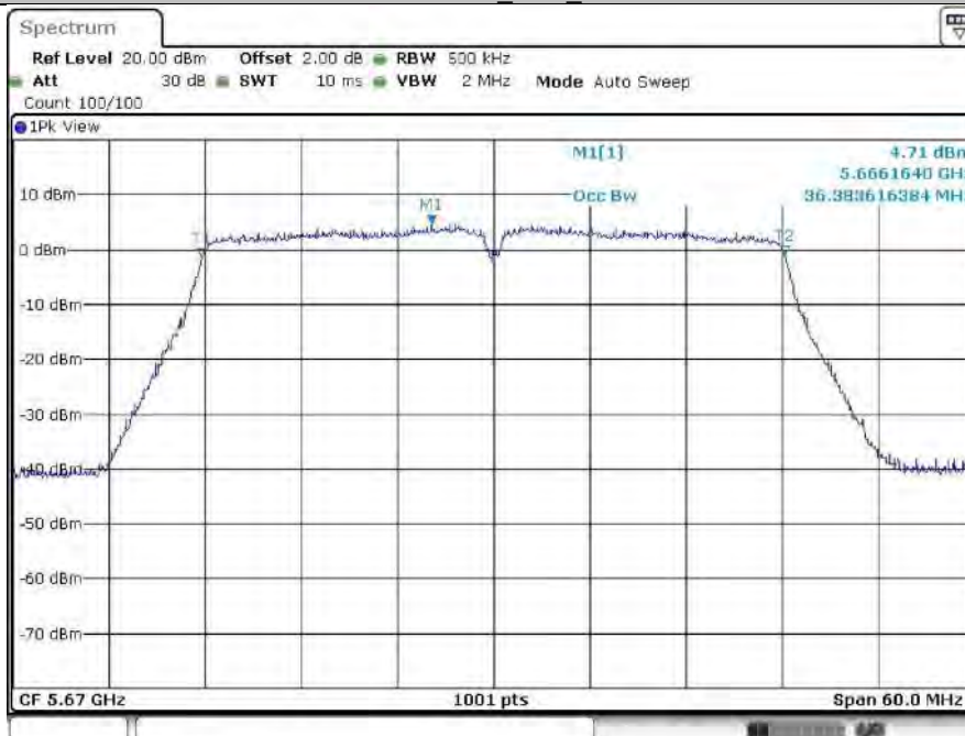
11N40MIMO_Ant1_5670
