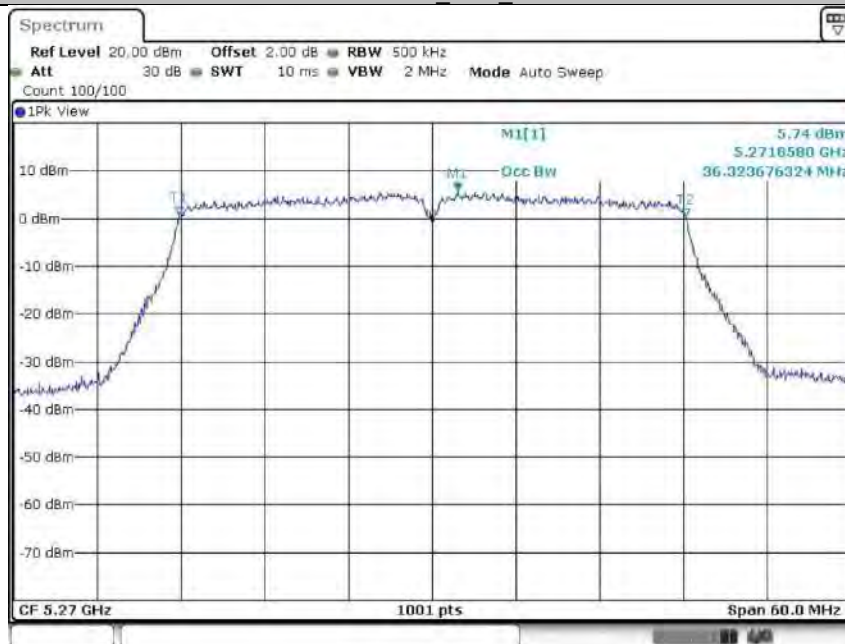
11N40MIMO_Ant2_5270
