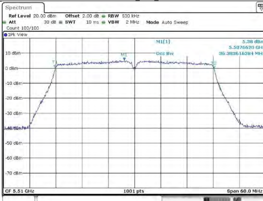
11N40MIMO_Ant1_5510
