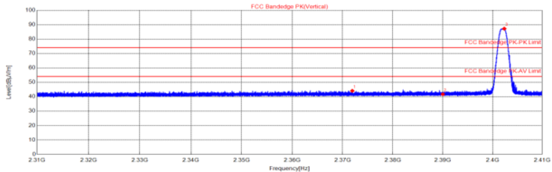
BLE_1M_2402_Ant1/ Vertical
