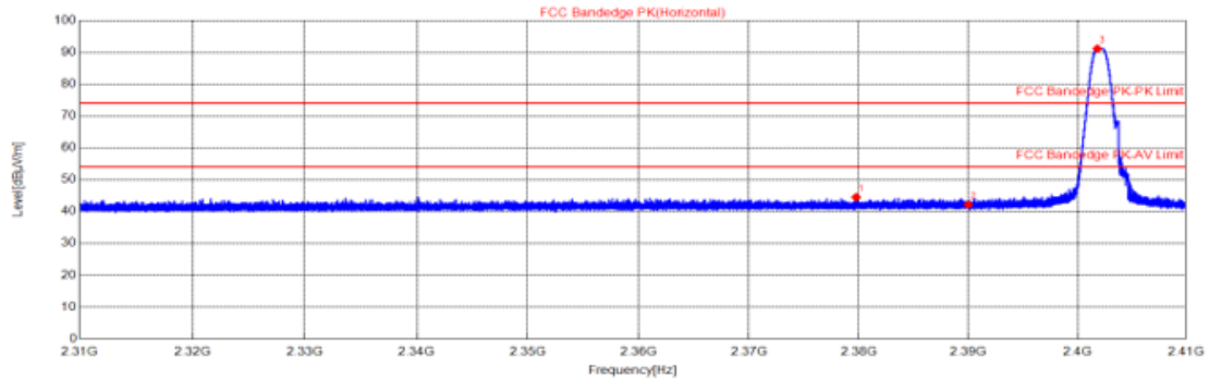
BLE_1M_2402_Ant1/ Horizontal
