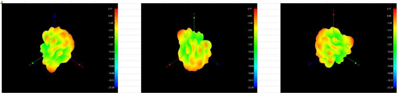
5150MHZ
