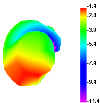
2480.000MHz
