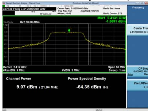
Antenna A
