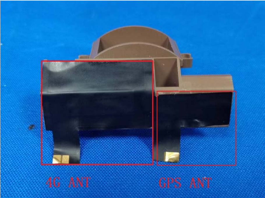
LTE/GPS Antenna
