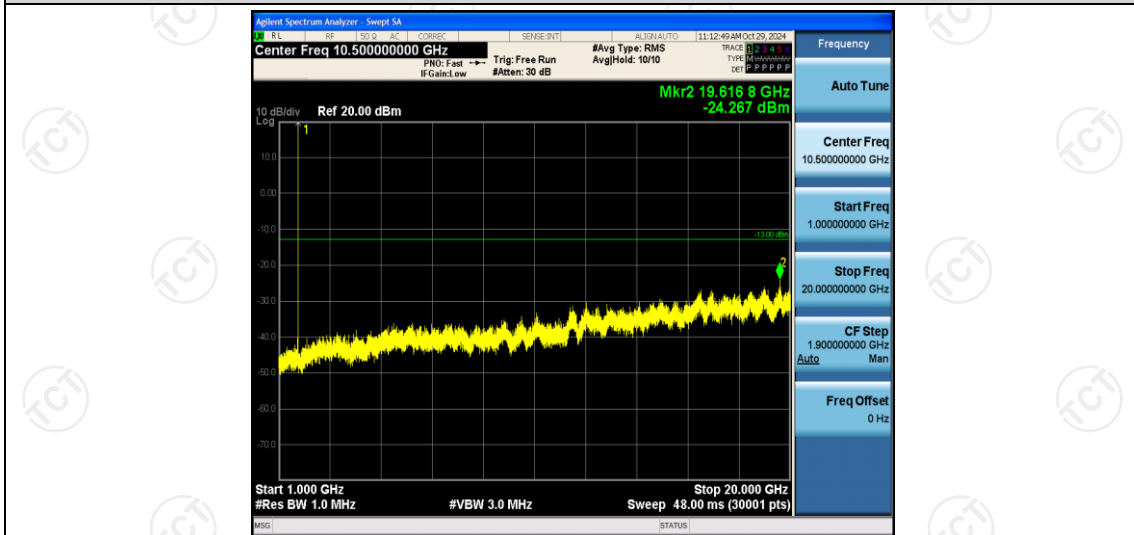
Band4-1.4MHz-QPSK-19957-1RB#0-Range2:1000~20000MHz
