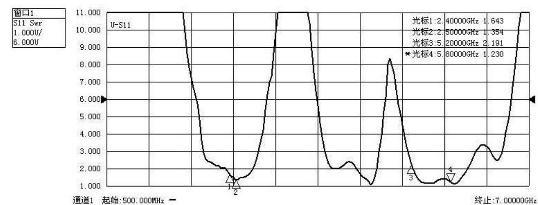
天线 VSWR 特性
