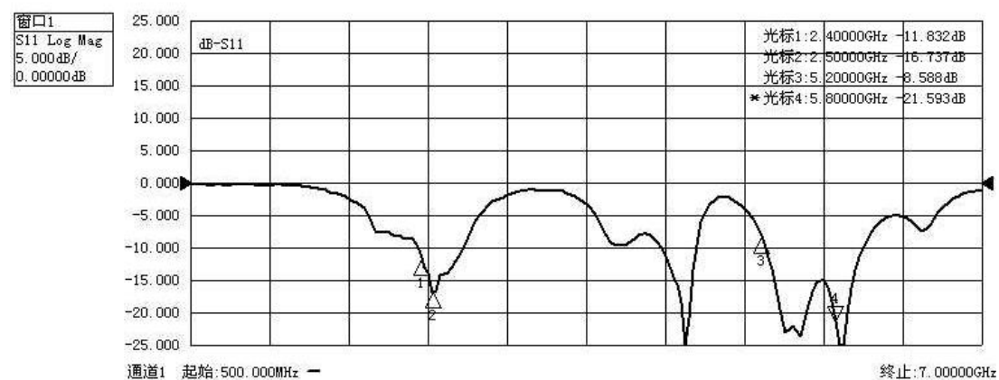
天线 S11 特性
