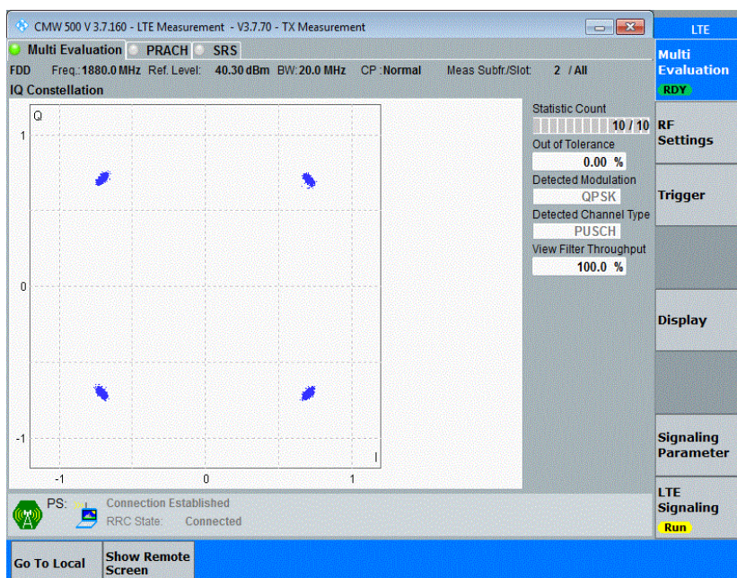
Band2-20MHz-QPSK-19100-100RB#0
