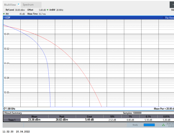
Band2-20MHz-QPSK-18900-100RB#0
