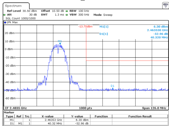
802.11b_2462MHz
