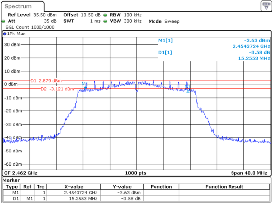
802.11n20_2462MHz
