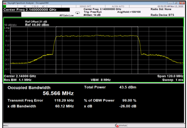
Figure 796: QPSK 60MHz B.W.; 2140.0MHz, 60kHz - Output
