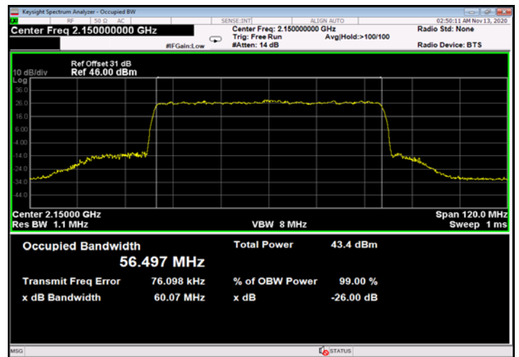
Figure 800: QPSK 60MHz B.W.; 2150.0MHz, 60kHz - Output
