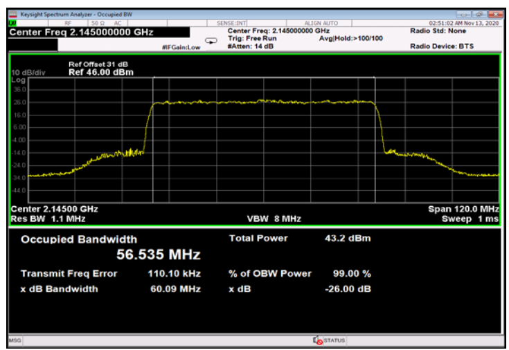
Figure 798: QPSK 60MHz B.W.; 2145.0MHz, 60kHz - Output
