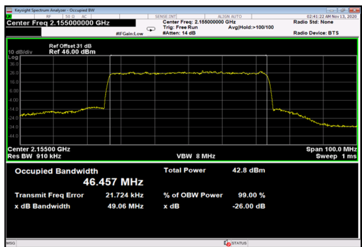
Figure 794: QPSK 50MHz B.W.; 2155.0MHz, 60kHz - Output
