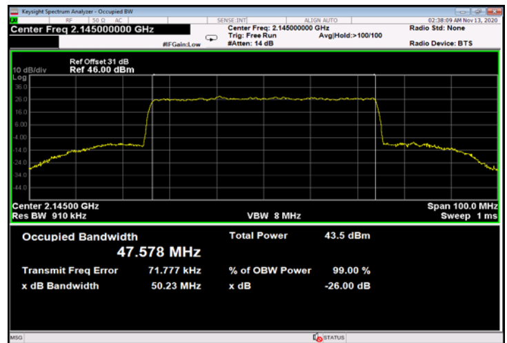
Figure 790: QPSK 50MHz B.W.; 2145.0MHz, 30kHz - Output
