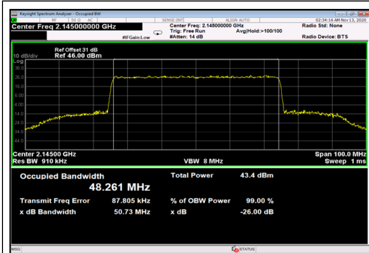
Figure 789: QPSK 50MHz B.W.; 2145.0MHz, 15kHz - Output
