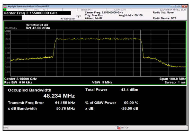
Figure 792: QPSK 50MHz B.W.; 2155.0MHz, 15kHz - Output
