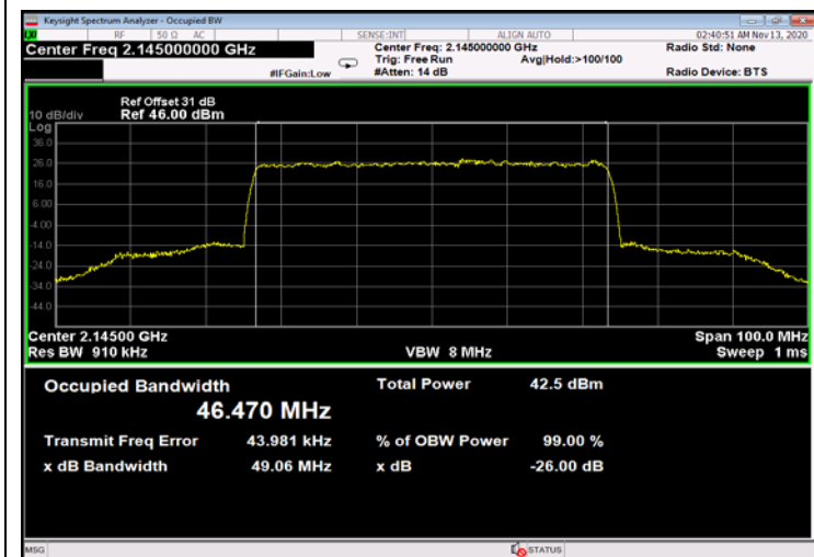
Figure 791: QPSK 50MHz B.W.; 2145.0MHz, 60kHz - Output
