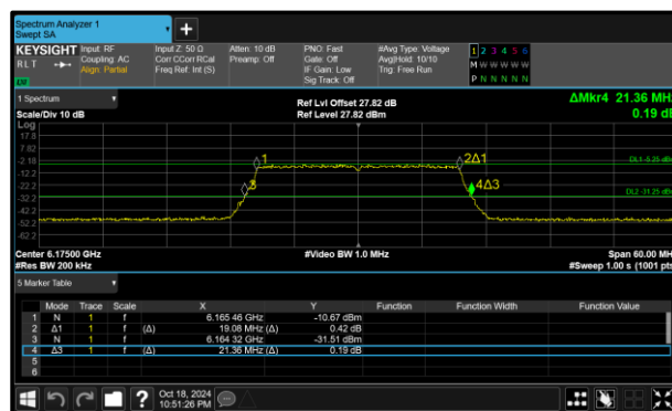
Figure 134 - 802.11ax HE20 SU LPI Maximum 99% OBW
