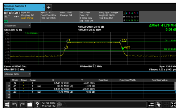
Figure 136 - 802.11ax HE40 SU LPI Maximum 99% OBW
