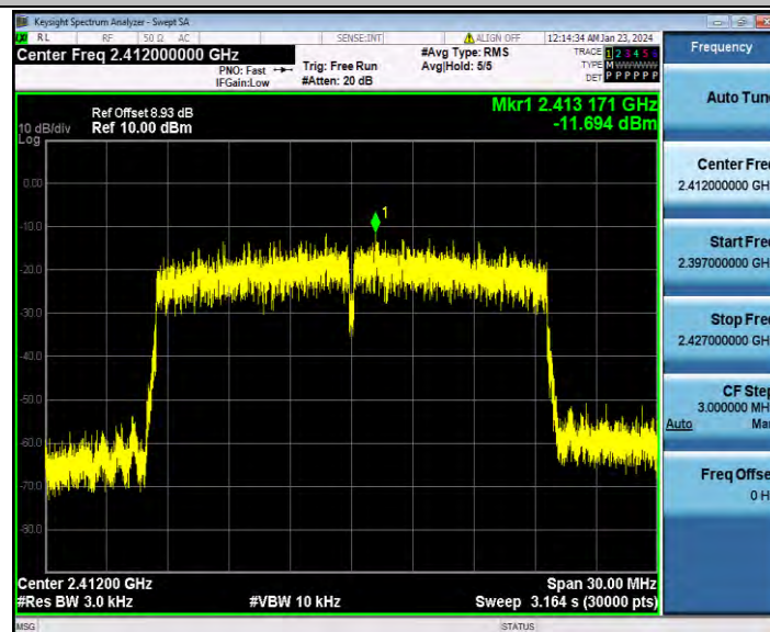
11AX20SISO_Ant0_2412
