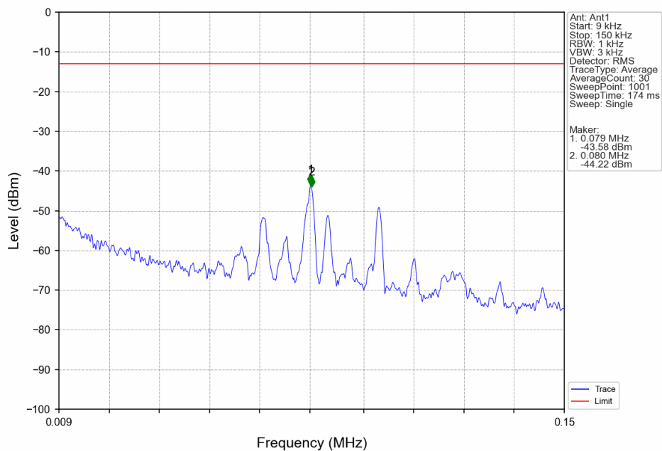
Band71 5MHz 16QAM MCH 680.5MHz RB 1 0 NTV
