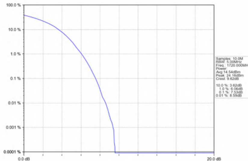
Band66_20MHz_256QAM_LCH_1720MHz_RB_100_0_NTNV
