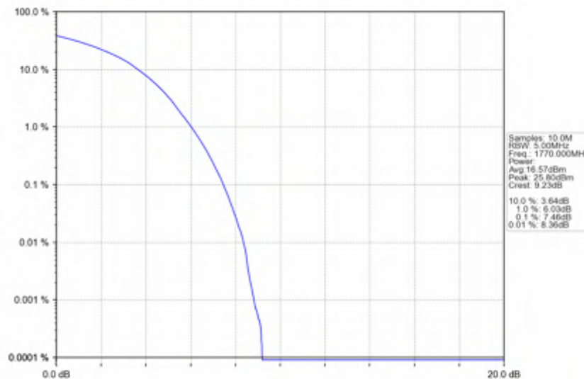
Band66_20MHz_QPSK_HCH_1770MHz_RB_100_0_NTNV
