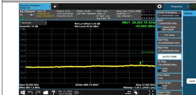
Band38-15MHz-QPSK-38175-1RB#0-20000~27000-PASS
