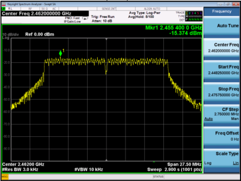
802.11n(HT20) 2462MHz
