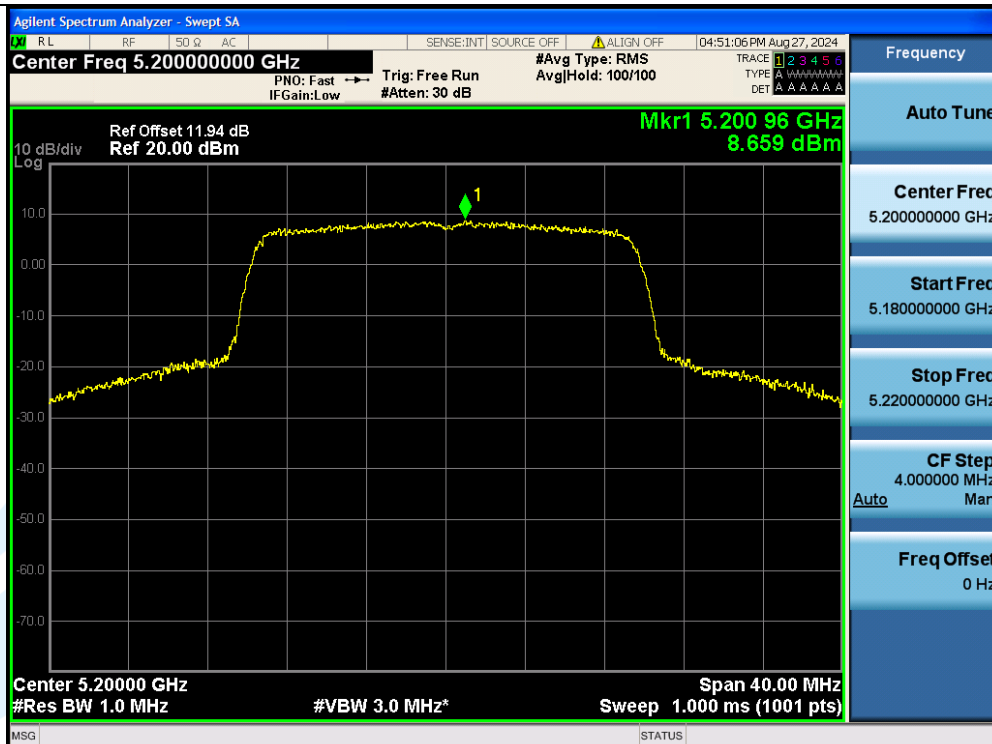
11AX20MIMO-Ant3-5200-PASS
