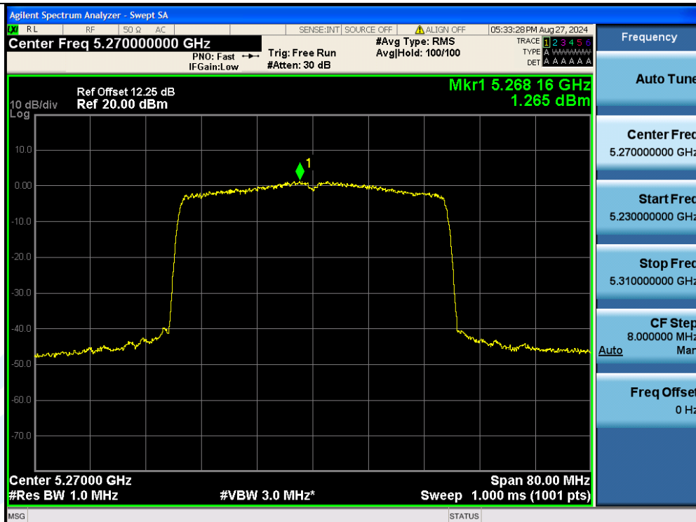
11AX40MIMO-Ant3-5270-PASS
