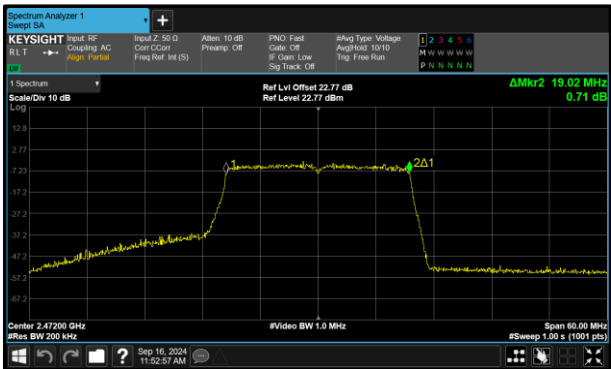
Figure 149 - 802.11ax HE20 SU Maximum 99% OBW
