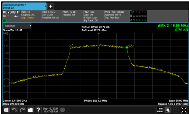
Figure 148 - 802.11ax HE20 SU Minimum 99% OBW
