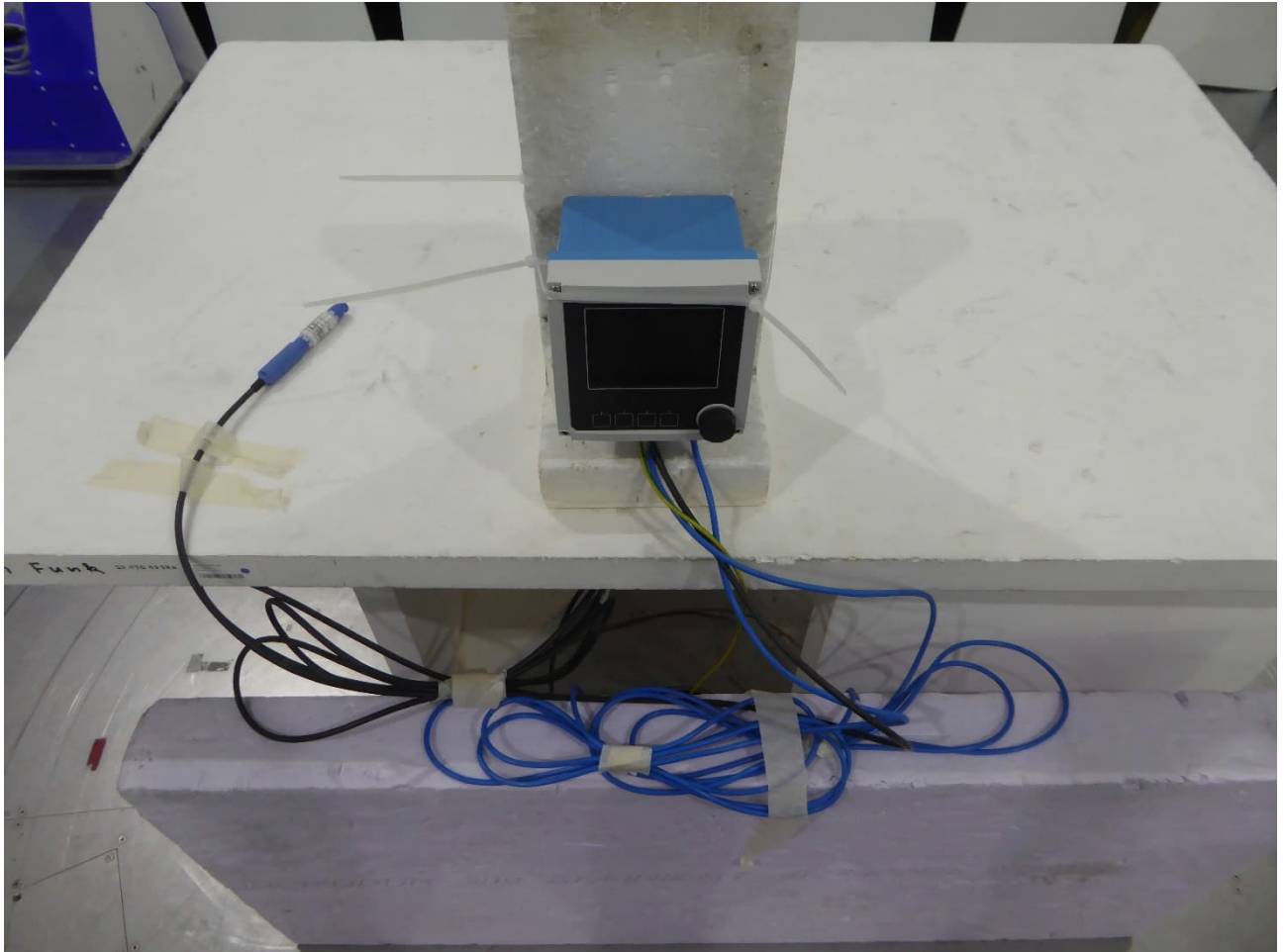
EUT setup
