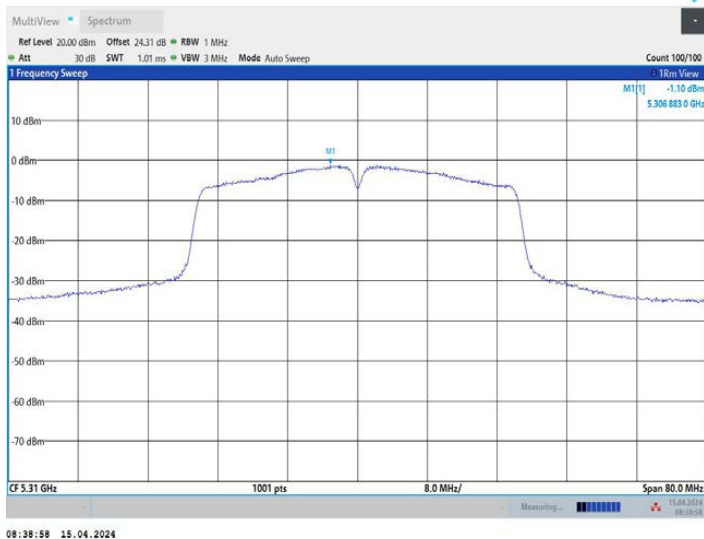
11AC40MIMO_Ant3_5310
