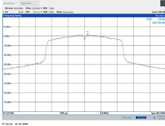
11N40MIMO_Ant3_5670
