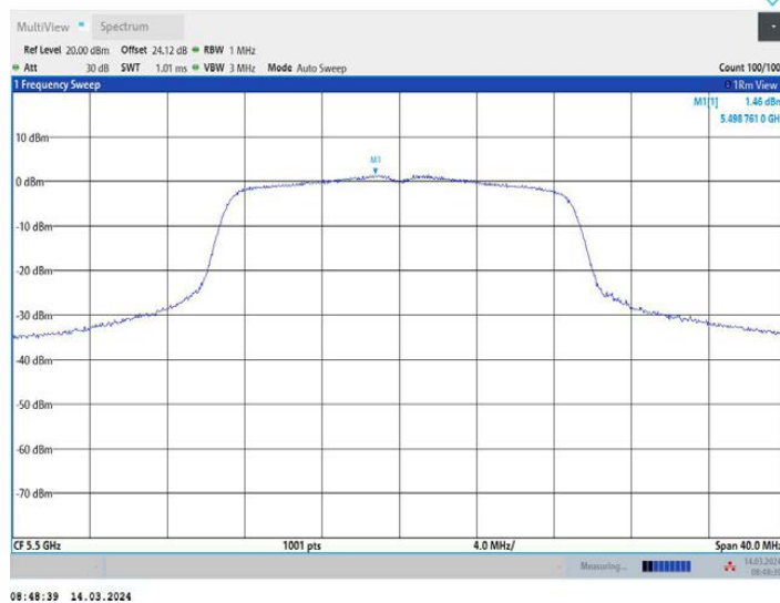
11AC20MIMO_Ant3_5500
