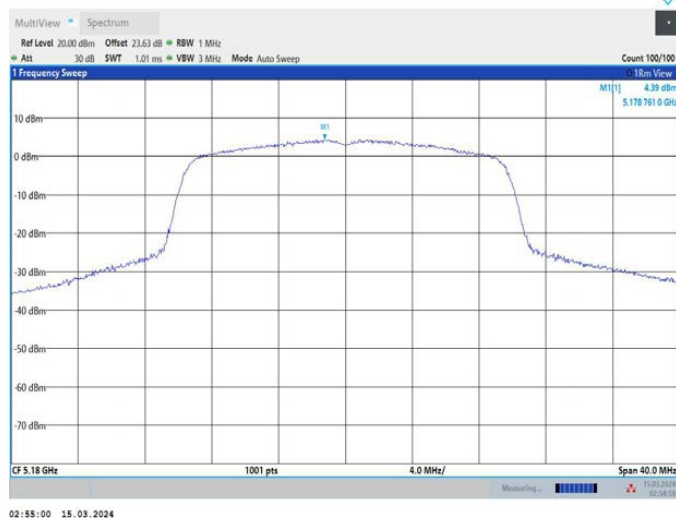
11AX20MIMO_Ant2_5180
