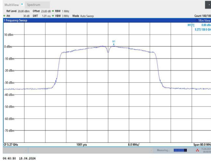
11N40MIMO_Ant3_5270
