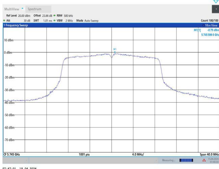
11AC20MIMO_Ant2_5745
