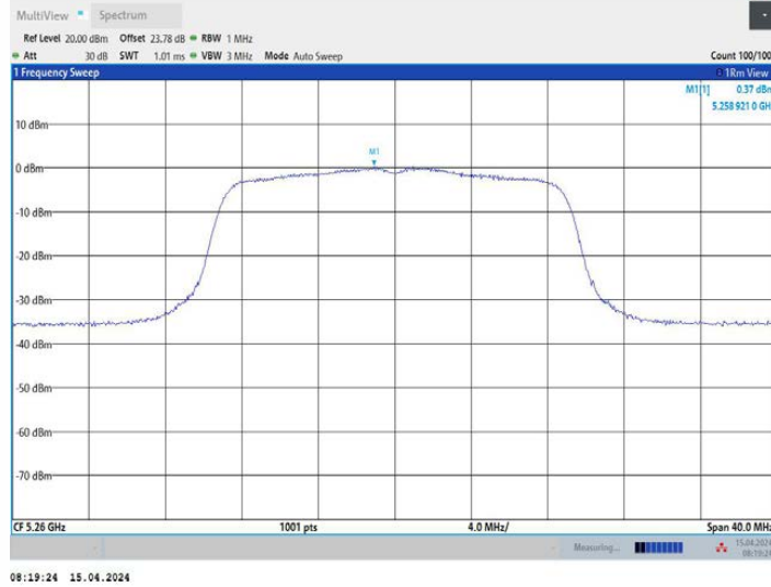
11AC20MIMO_Ant3_5260
