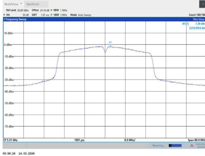
11N40MIMO_Ant3_5510
