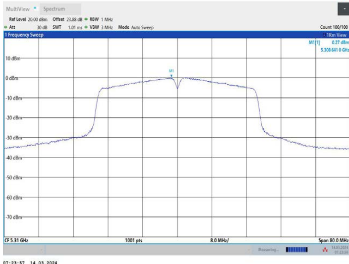
11N40MIMO_Ant2_5310
