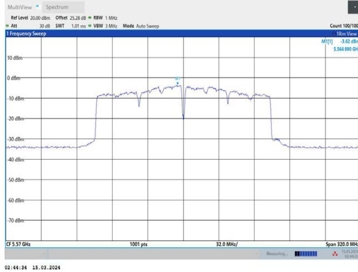
11AC160MIMO_Ant2_5570
