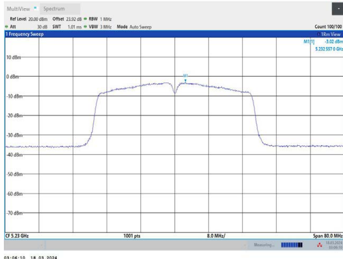
11AC40MIMO_Ant3_5230
