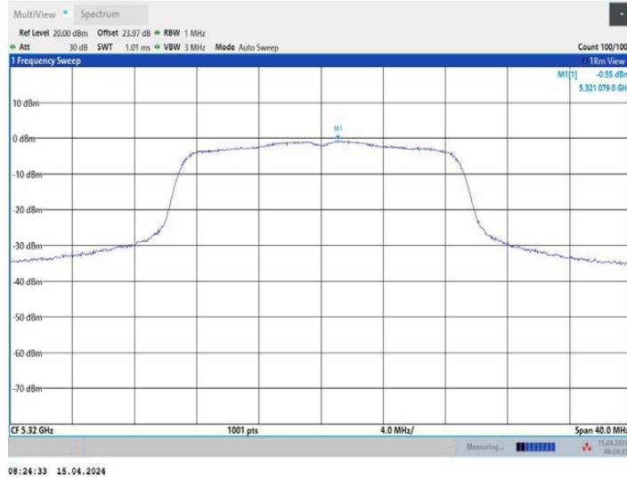
11AC20MIMO_Ant3_5320
