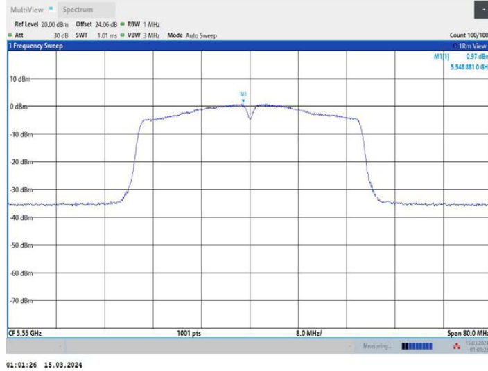
11AC40MIMO_Ant3_5550
