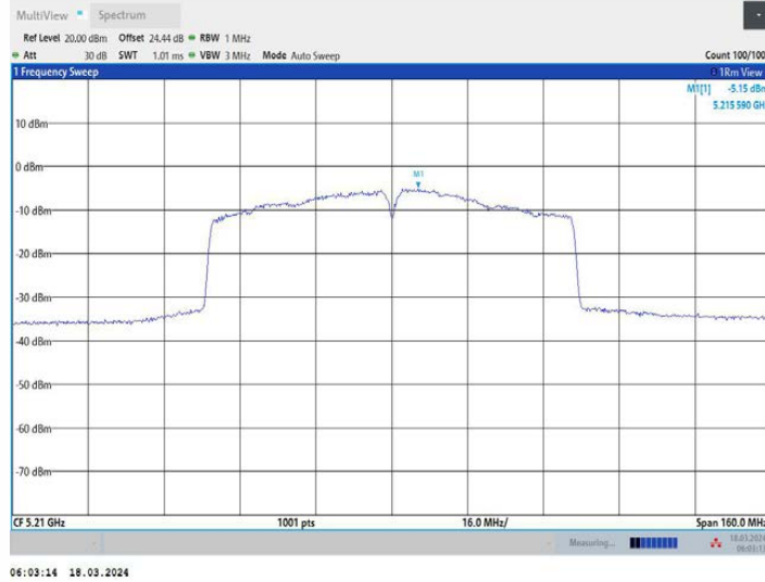
11AC80MIMO_Ant3_5210
