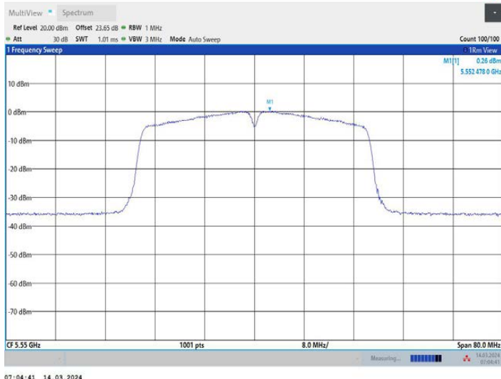
11N40MIMO_Ant2_5550
