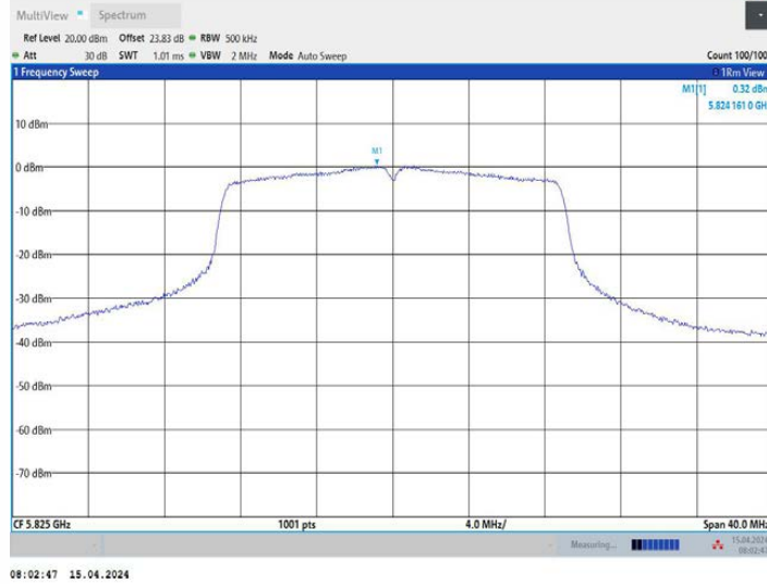
11AC20MIMO_Ant3_5825
