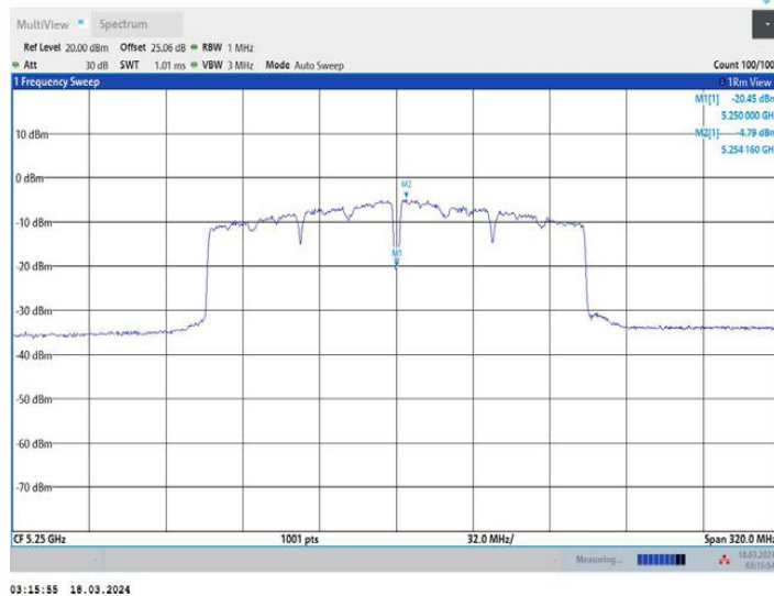
11AC160MIMO_Ant2_5250_UNII-2A
