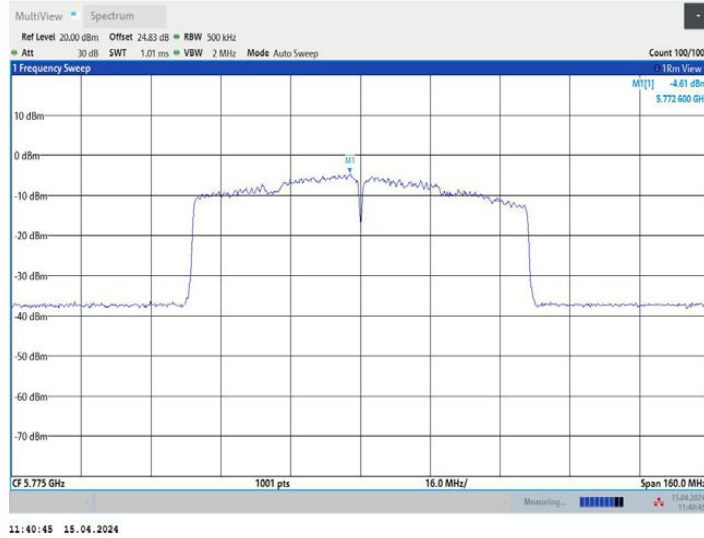
11AC80MIMO_Ant3_5775
