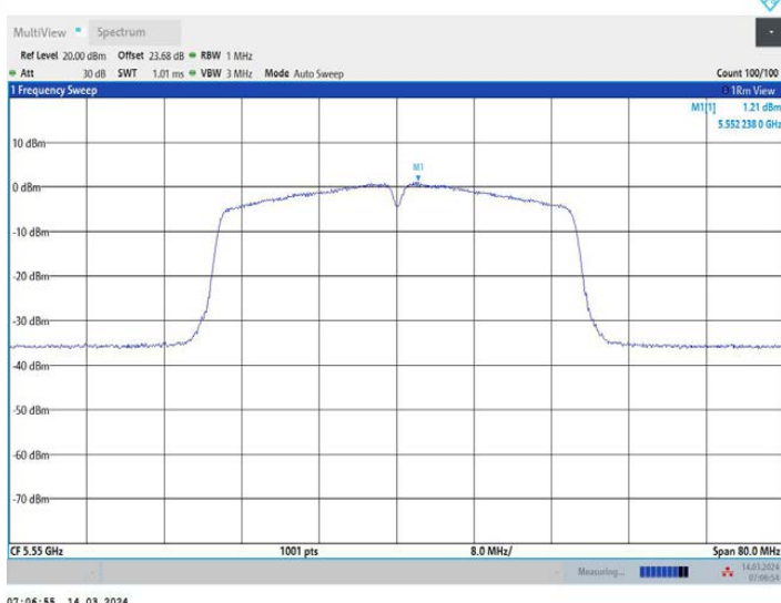
11N40MIMO_Ant3_5550
