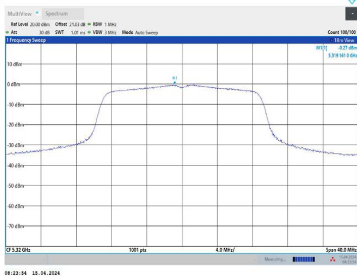
11AC20MIMO_Ant2_5320
