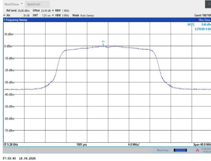
11N20MIMO_Ant3_5280
