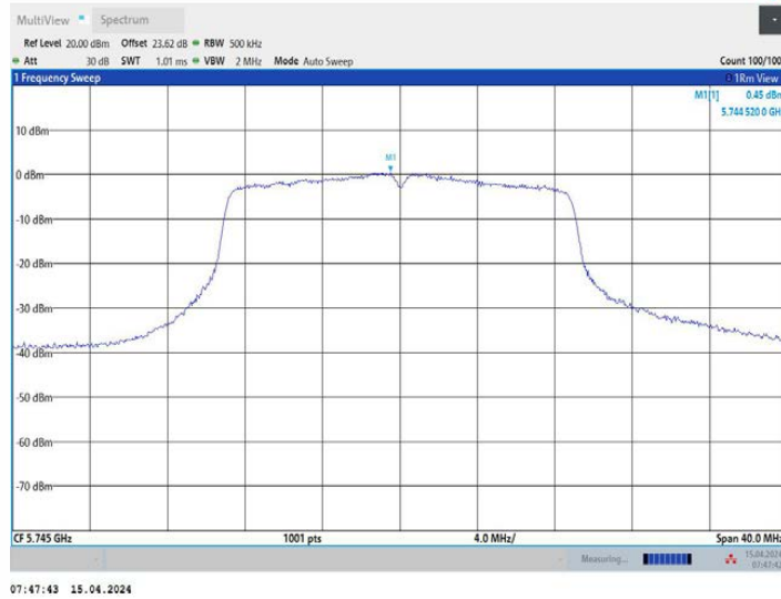
11AC20MIMO_Ant3_5745
