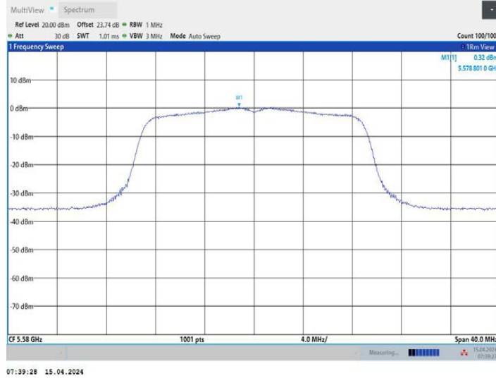
11AC20MIMO_Ant3_5580
