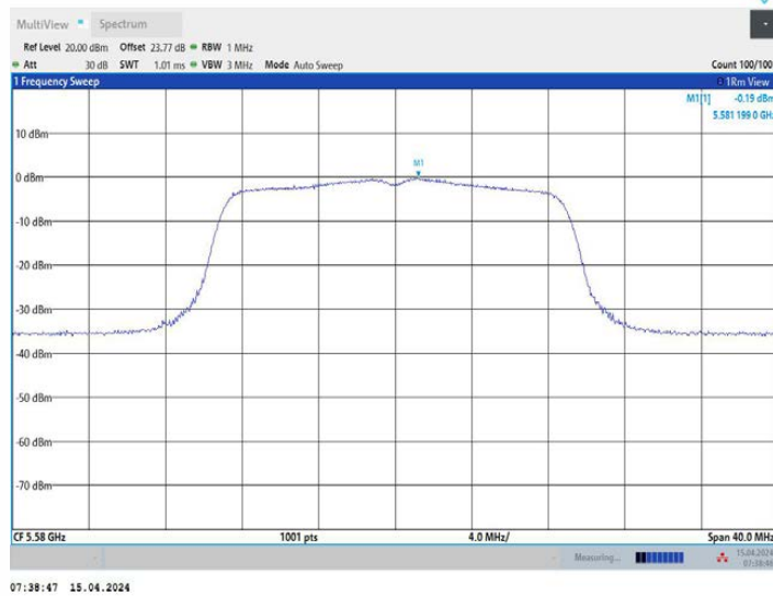
11AC20MIMO_Ant2_5580
