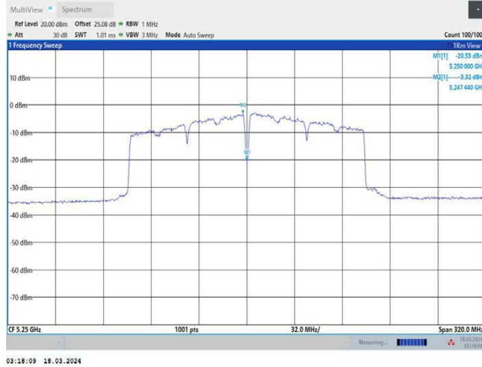
11AC160MIMO_Ant1_5250_UNII-2A
