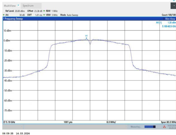
11N40MIMO_Ant2_5190
