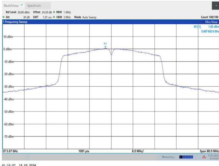
11AC40MIMO_Ant2_5670
