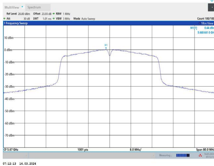
11N40MIMO_Ant2_5670
