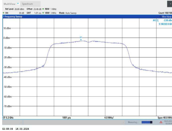
11AC20MIMO_Ant3_5200
