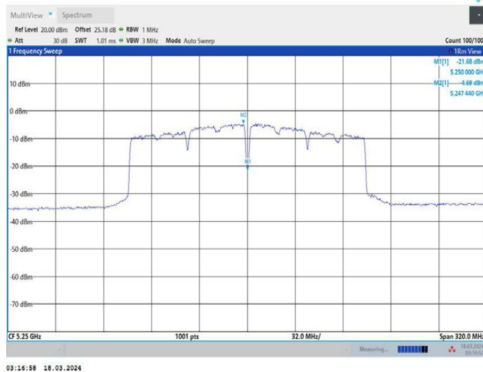
11AC160MIMO_Ant3_5250_UNII-1
