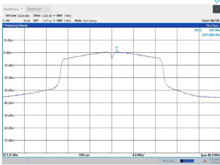
11N40MIMO_Ant3_5310
