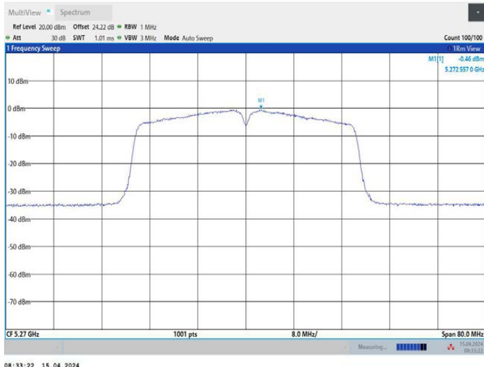
11AC40MIMO_Ant2_5270
