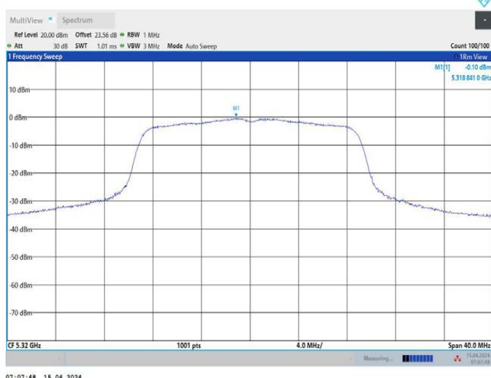
11N20MIMO_Ant3_5320
