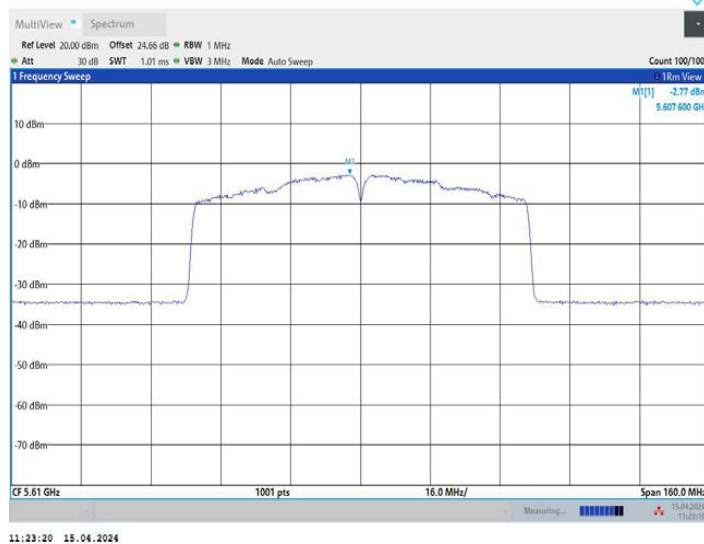
11AC80MIMO_Ant3_5610
