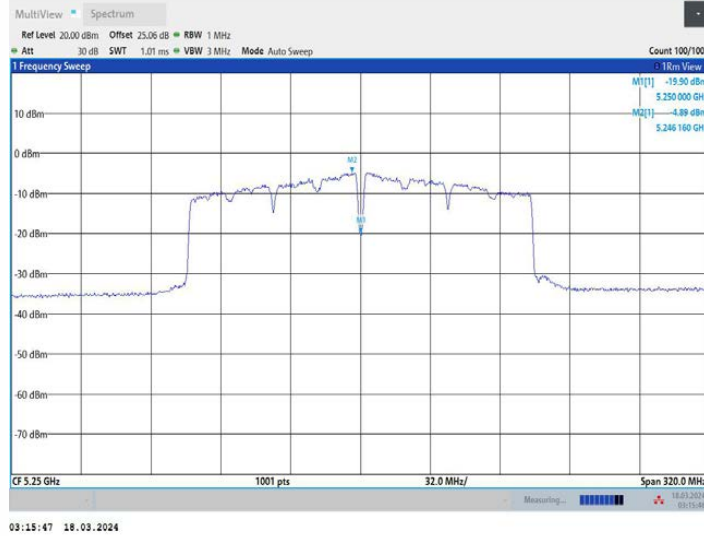
11AC160MIMO_Ant2_5250_UNII-1
