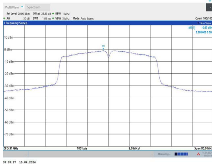
11AC40MIMO_Ant2_5310
