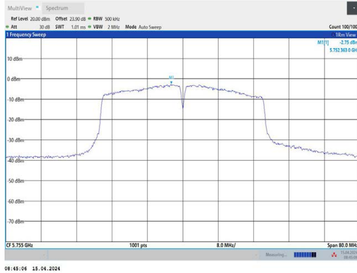
11AC40MIMO_Ant3_5755
