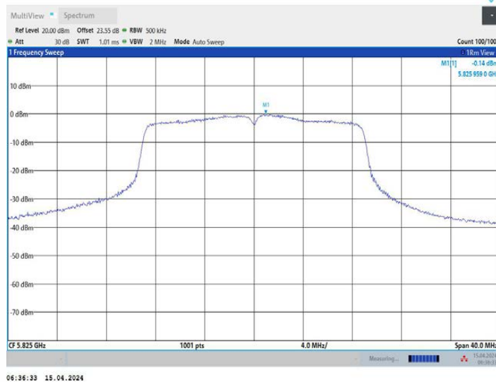
11N20MIMO_Ant3_5825
