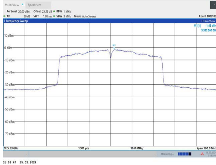
11AC80MIMO_Ant3_5530
