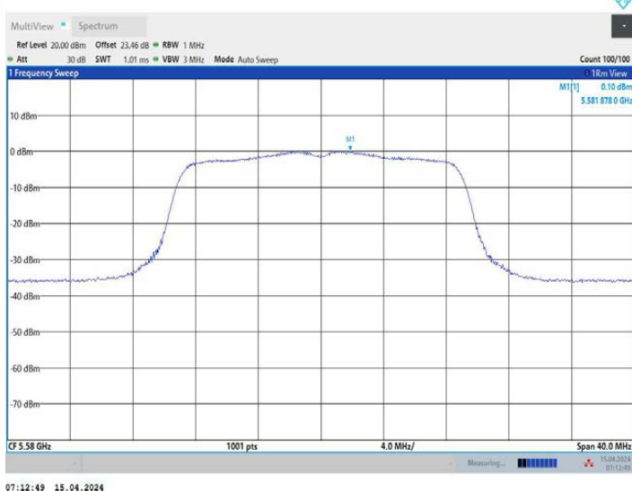
11N20MIMO_Ant3_5580
