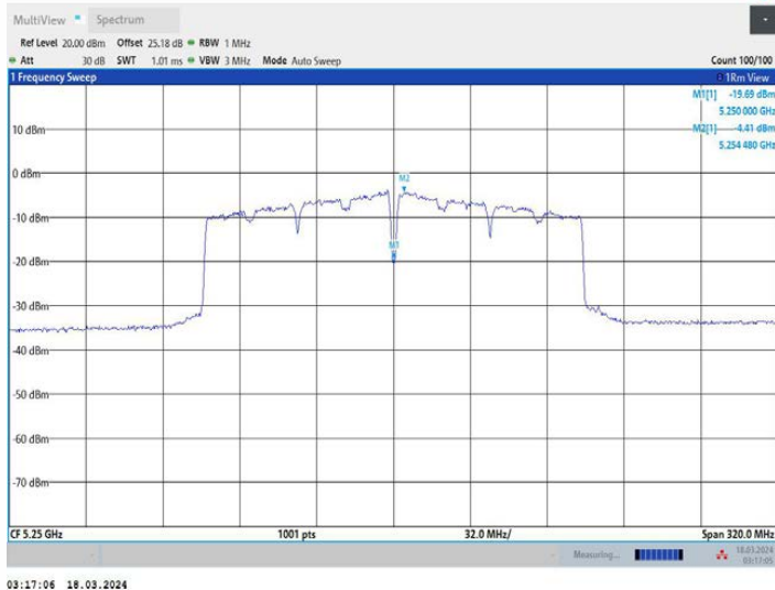
11AC160MIMO_Ant3_5250_UNII-2A
