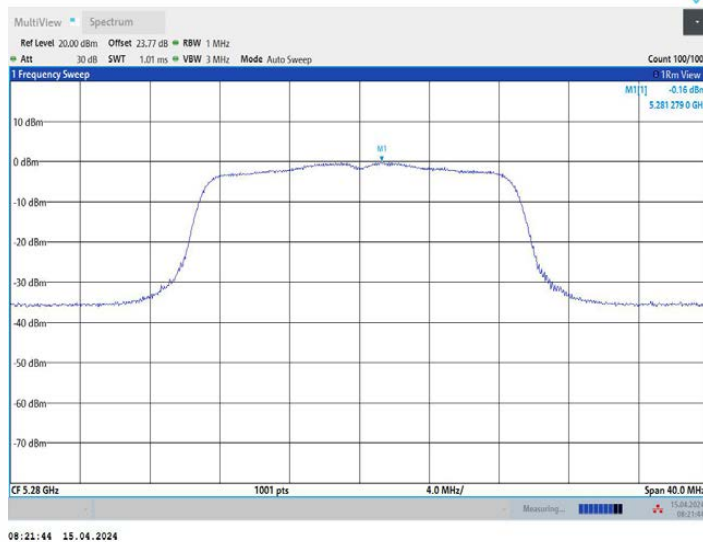
11AC20MIMO_Ant3_5280
