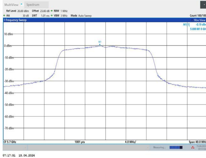
11N20MIMO_Ant3_5700
