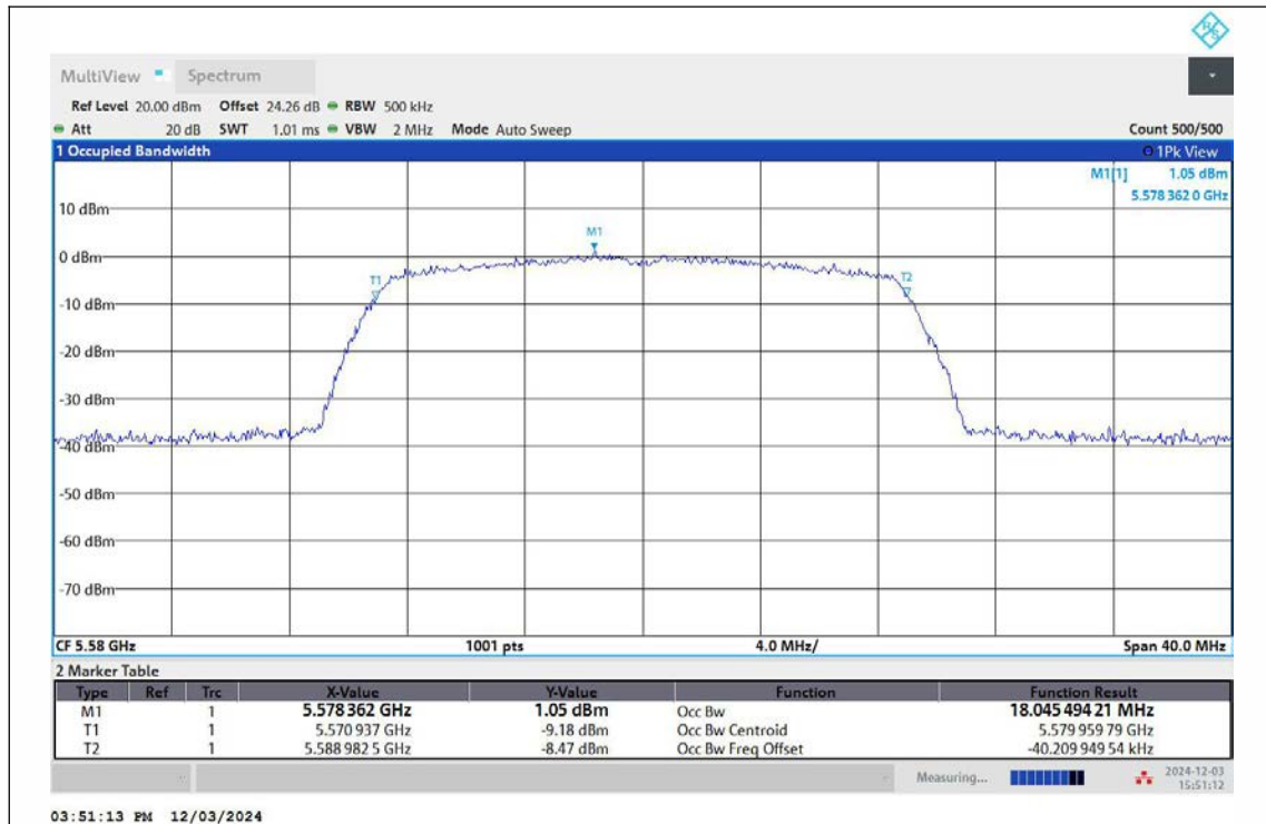
11N20MIMO-Ant1-5580
