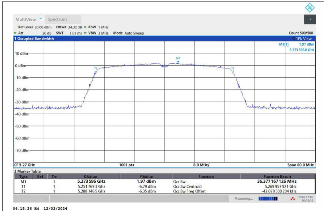
11N40MIMO-Ant1-5270
