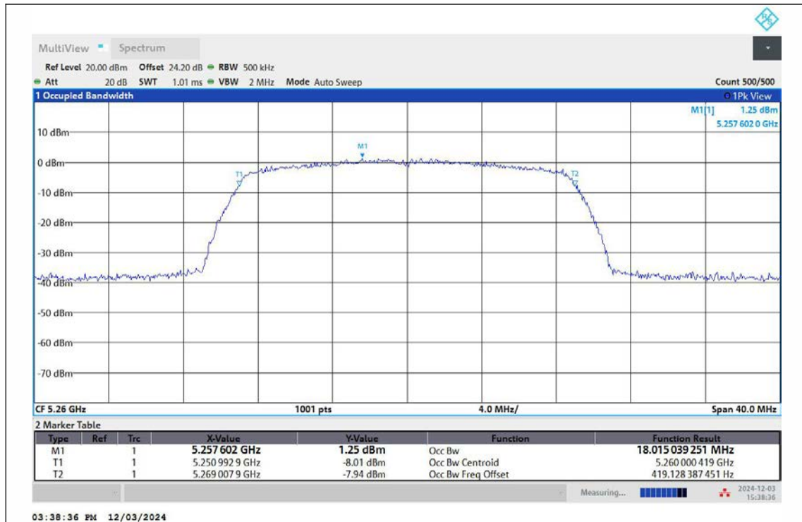
11N20MIMO-Ant1-5260
