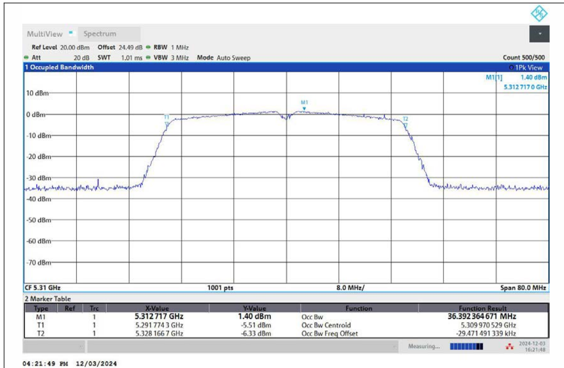
11N40MIMO-Ant1-5310
