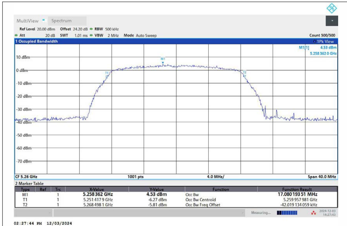
11A-Ant1-5260
