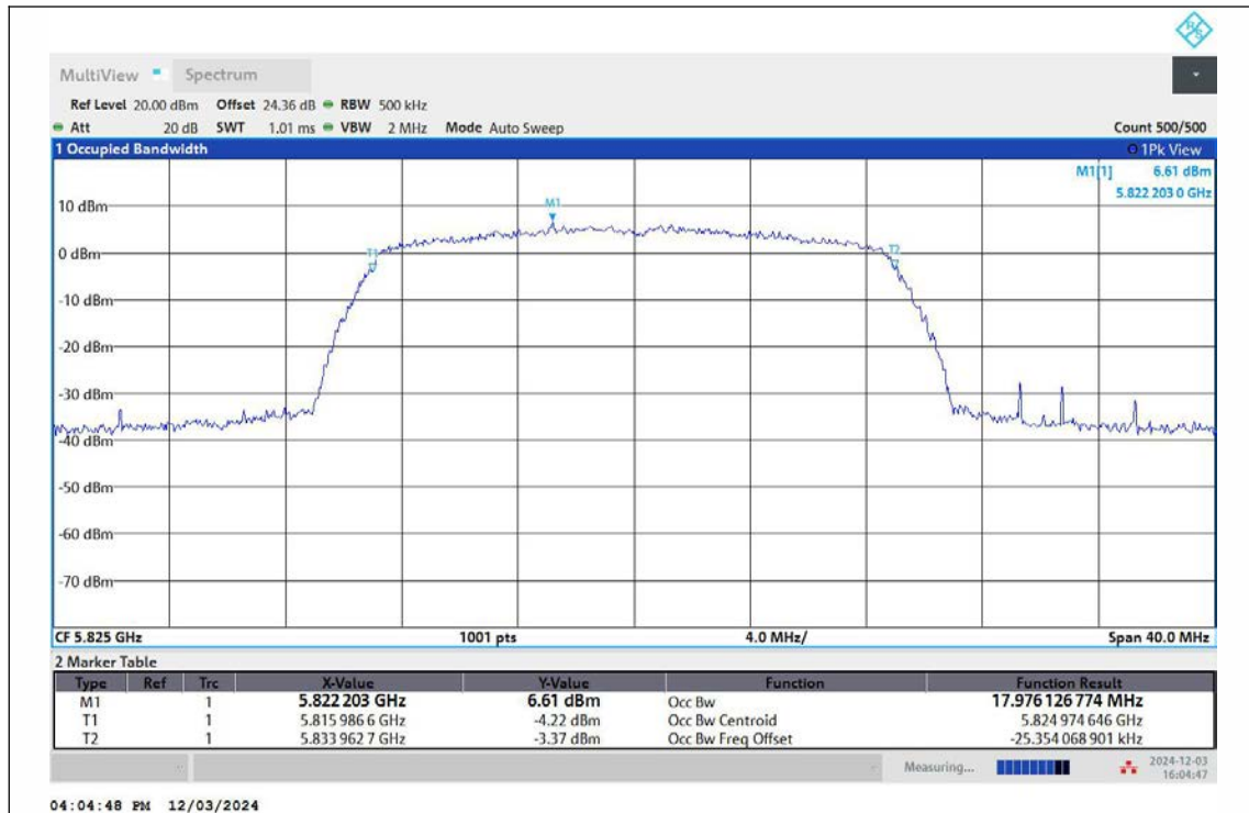
11N20MIMO-Ant1-5825
