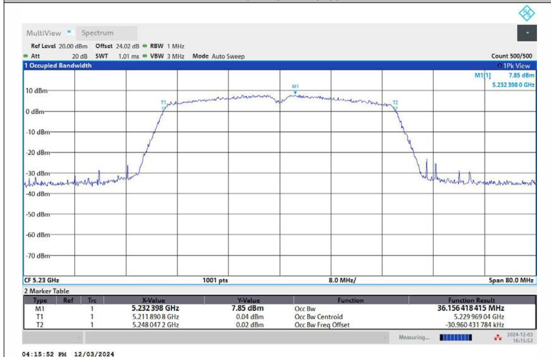
11N40MIMO-Ant2-5230
