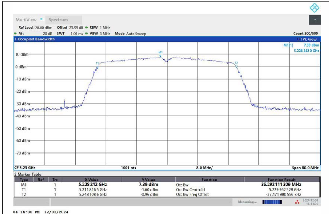
11N40MIMO-Ant1-5230
