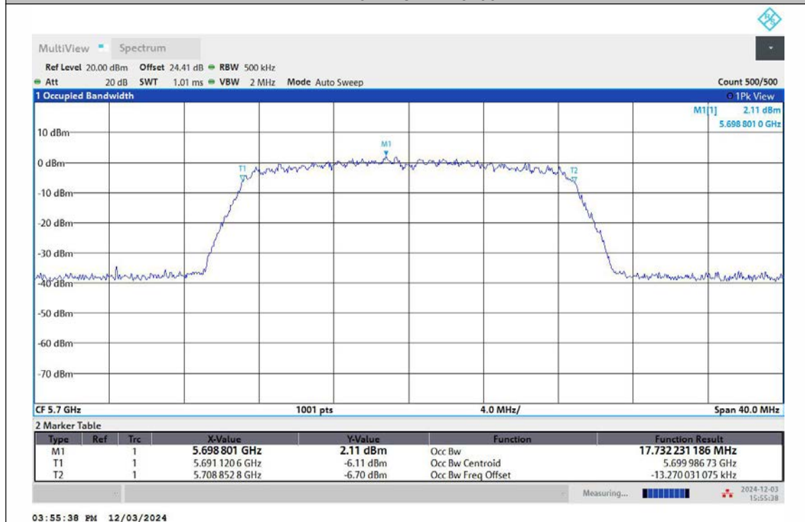
11N20MIMO-Ant2-5700
