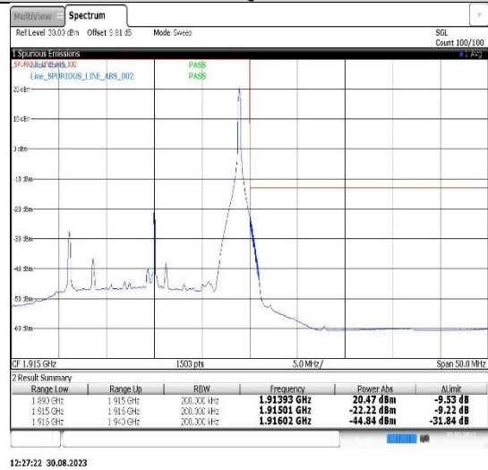
Band25-20MHz-16QAM-26590-1RB#99
