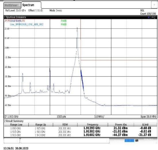
Band25-20MHz-QPSK-26590-1RB#99
