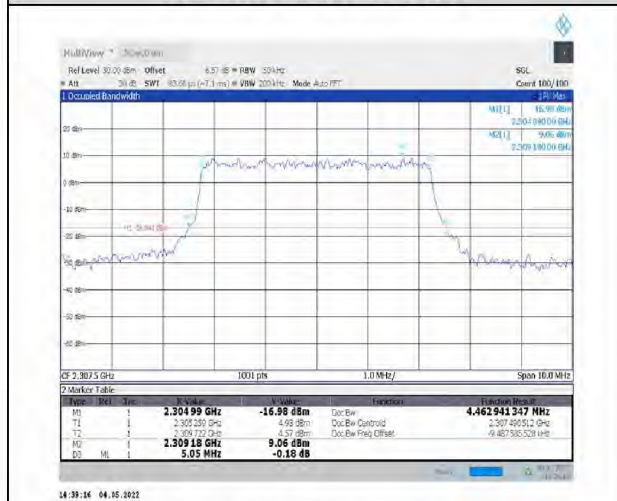
1-N30--15-5-L-7-CP-16QAM-Outer_Full-25@0-Ant1-4.463-5.050-≤5-PASS
