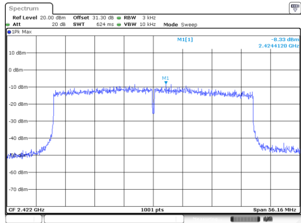
MIMO Ant. 8
