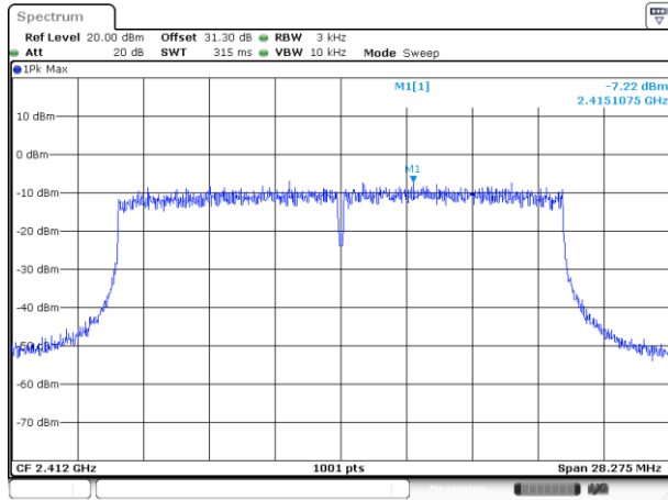
MIMO Ant. 7
