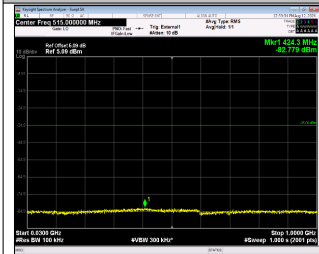
41-41-5MHz-20MHz-QPSK-QPSK-39683-39800-25RB#0-100RB#0-30~1000MHz-PASS
