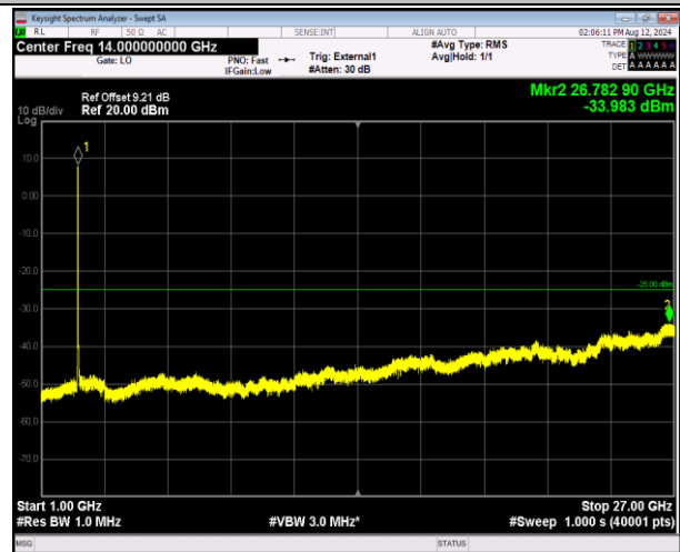
41-41-20MHz-5MHz-QPSK-QPSK-39750-39867-100RB#0-25RB#0-1000~27000MHz-PASS
