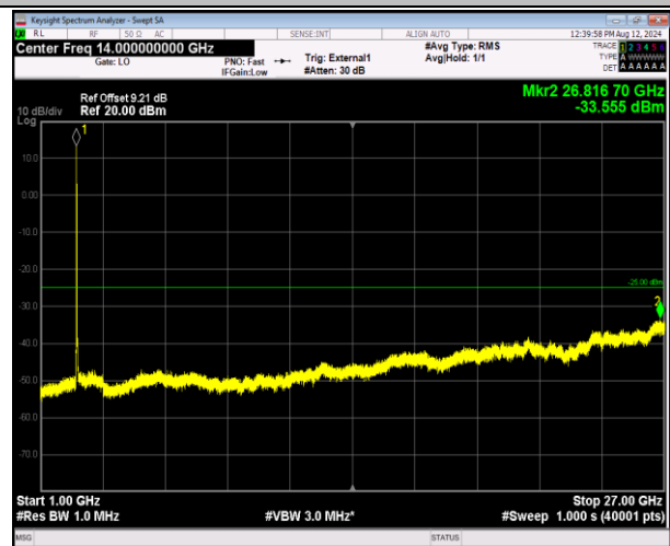
41-41-5MHz-20MHz-QPSK-QPSK-39683-39800-25RB#0-100RB#0-1000~27000MHz-PASS
