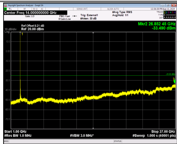
41-41-5MHz-20MHz-QPSK-QPSK-39683-39800-1RB#24-0RB#0-1000~27000MHz-PASS
