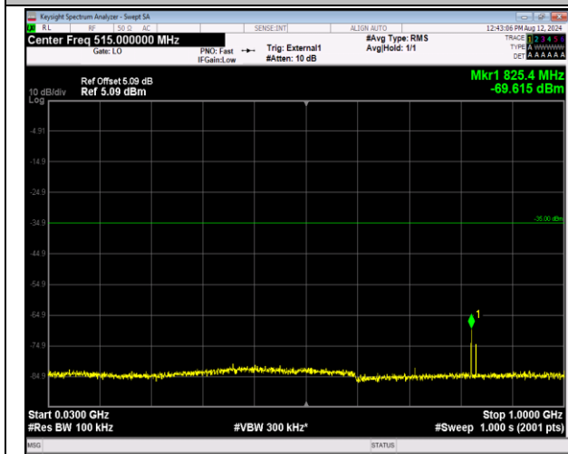
41-41-5MHz-20MHz-QPSK-QPSK-40528-40645-1RB#24-0-0RB#0-30~1000MHz-PASS
