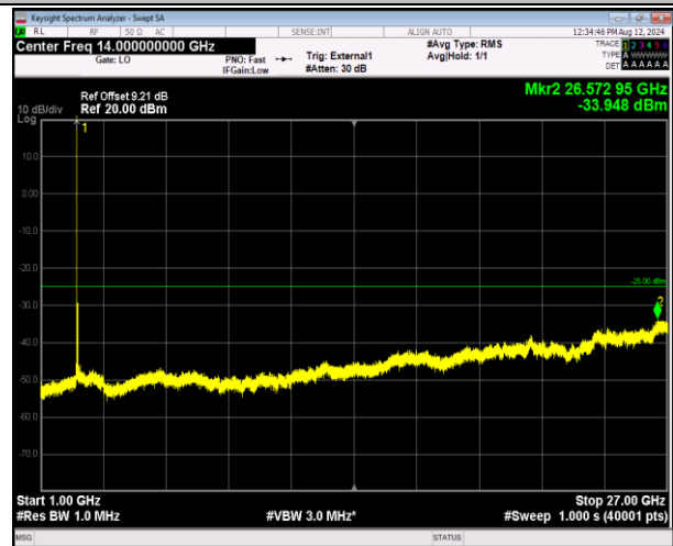
41-41-5MHz-20MHz-QPSK-QPSK-39683-39800-1RB#0-0R B#0-1000~27000MHz-PASS
