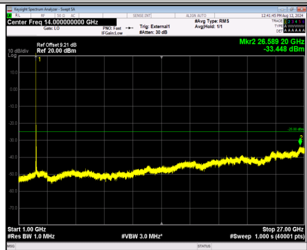
41-41-5MHz-20MHz-QPSK-QPSK-40528-40645-1RB#0-ORB#0-1000~27000MHz-PASS
