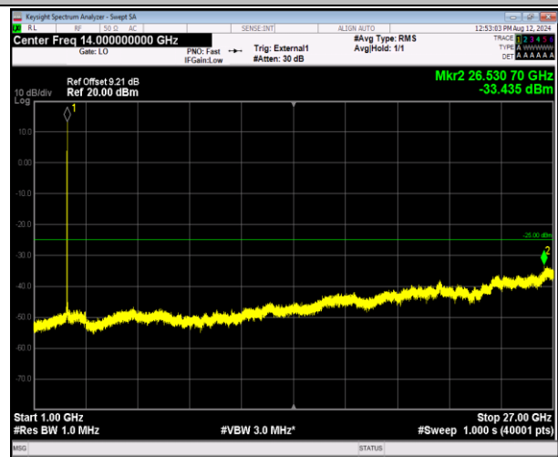
41-41-5MHz-20MHz-16QAM-16QAM-41373-41490-1RB#0- 1RB#99-1000~27000MHz-PASS
