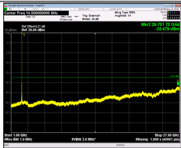
41-41-5MHz-20MHz-QPSK-QPSK-41373-41490-1RB#24-0-0RB#0-1000~27000MHz-PASS
