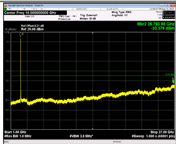
41-41-5MHz-20MHz-QPSK-QPSK-40528-40645-25RB#0-100RB#0-1000~27000MHz-PASS
