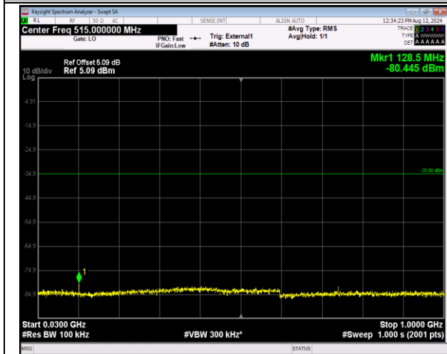
41-41-5MHz-20MHz-QPSK-QPSK-39683-39800-1RB#0-0- ORB#0-30~1000MHz-PASS
