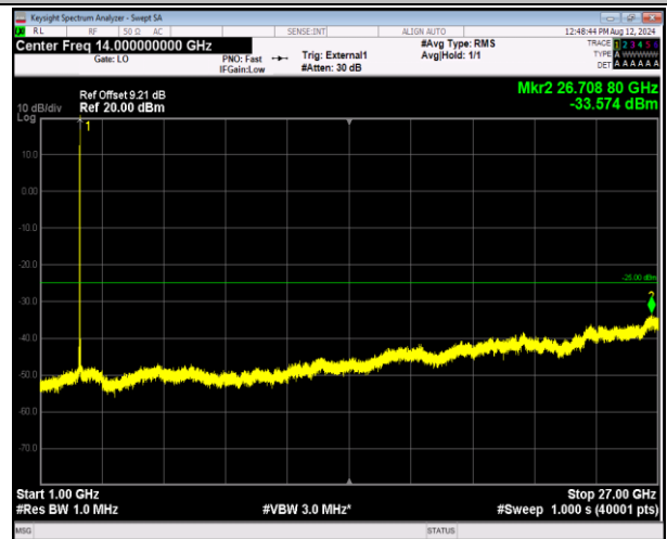
41-41-5MHz-20MHz-QPSK-QPSK-41373-41490-1RB#0-ORB#0-1000~27000MHz-PASS
