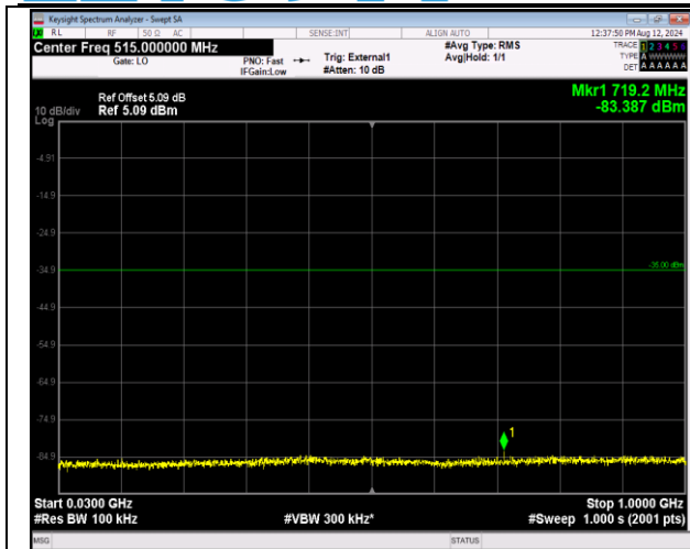
41-41-5MHz-20MHz-QPSK-QPSK-39683-39800-1RB#0-1RB#99-30~1000MHz-PASS
