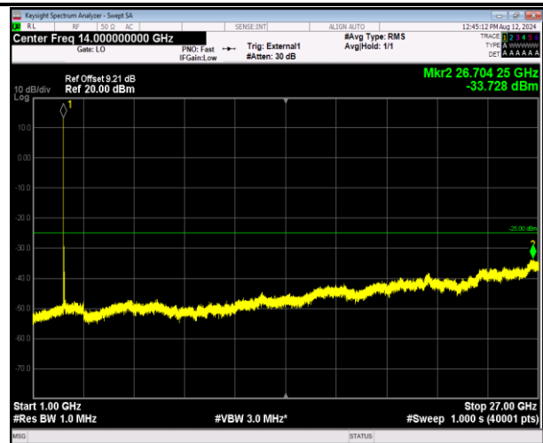
41-41-5MHz-20MHz-QPSK-QPSK-40528-40645-1RB#0-1RB#99-1000~27000MHz-PASS
