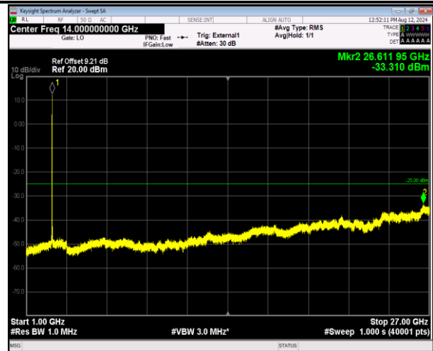
41-41-5MHz-20MHz-QPSK-QPSK-41373-41490-1RB#0-1RB#99-1000~27000MHz-PASS
