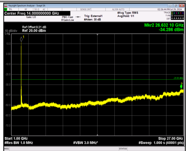
41-41-5MHz-20MHz-64QAM-64QAM-39683-39800-1RB#0- 1RB#99-1000~27000MHz-PASS
