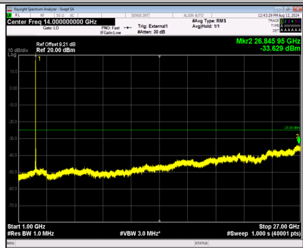
41-41-5MHz-20MHz-QPSK-QPSK-40528-40645-1RB#24-0-0RB#0-1000~27000MHz-PASS
