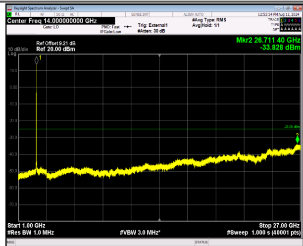
41-41-5MHz-20MHz-QPSK-QPSK-41373-41490-25RB#0-100RB#0-1000~27000MHz-PASS
