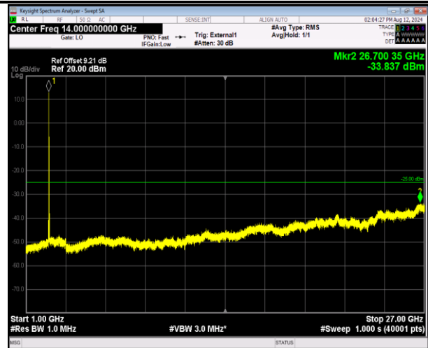
41-41-20MHz-5MHz-QPSK-QPSK-39750-39867-1RB#0-1RB#24-1000~27000MHz-PASS
