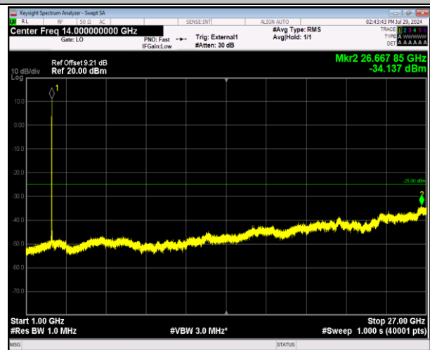
41-41-5MHz-20MHz-64QAM-64QAM-41373-41490-1RB#0- 1RB#99-1000~27000MHz-PASS
