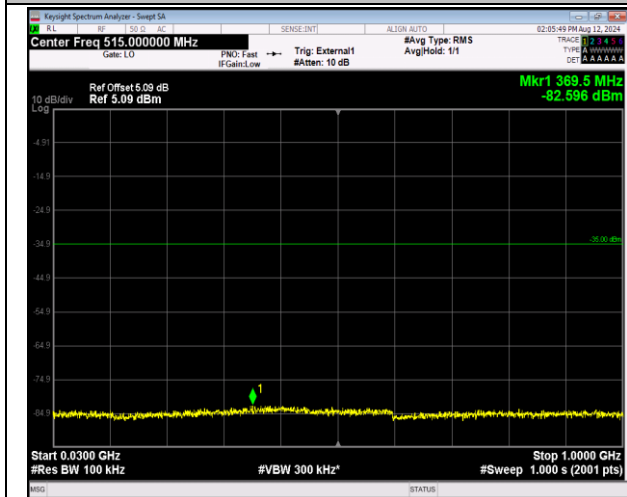
41-41-20MHz-5MHz-QPSK-QPSK-39750-39867-100RB#0-25RB#0-30~1000MHz-PASS
