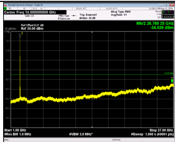
41-41-5MHz-20MHz-QPSK-QPSK-39683-39800-1RB#0-1RB#99-1000~27000MHz-PASS
