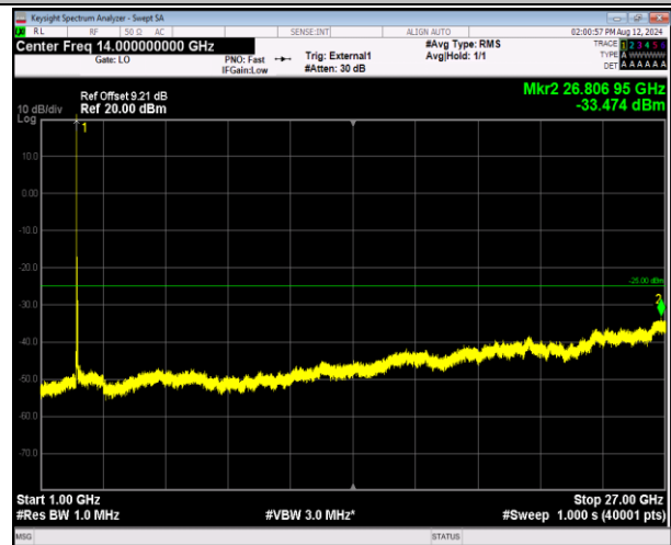
41-41-20MHz-5MHz-QPSK-QPSK-39750-39867-1RB#0-0R B#0-1000~27000MHz-PASS
