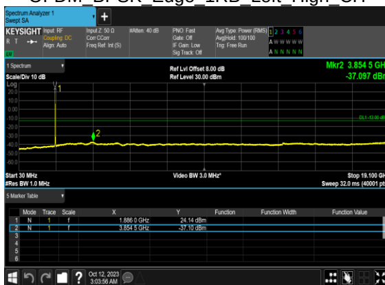
N2(25M)_DFT-s- OFDM BPSK Edge 1RB Left High CH
