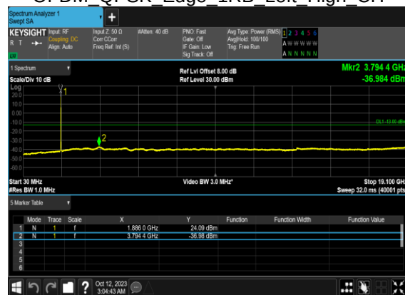
N2(25M)_DFT-s- OFDM QPSK Edge 1RB Left High CH
