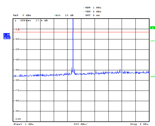
GSM 1900 CH-Middle 1GHz~3GHz
