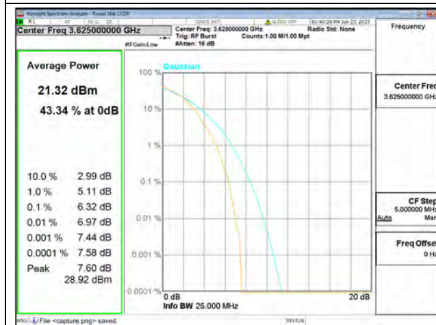
Band48 / 20MHz / Mid CH / 64QAM
