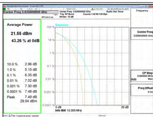
Band48 / 10MHz / Mid CH / 16QAM
