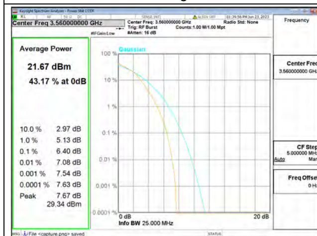
Band48 / 20MHz / Low CH / 16QAM
