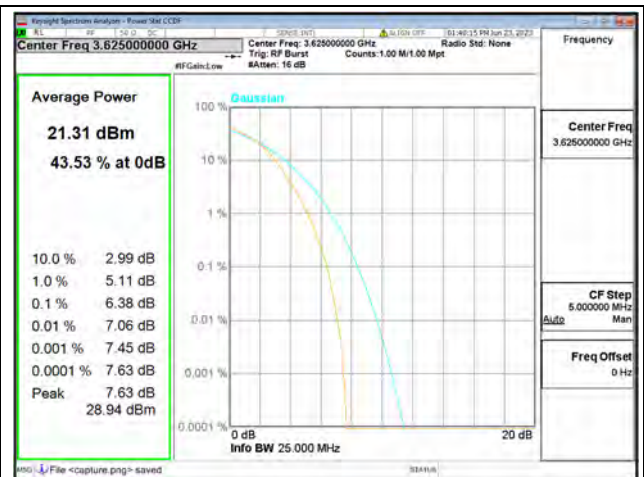
Band48 / 20MHz / Mid CH / 16QAM
