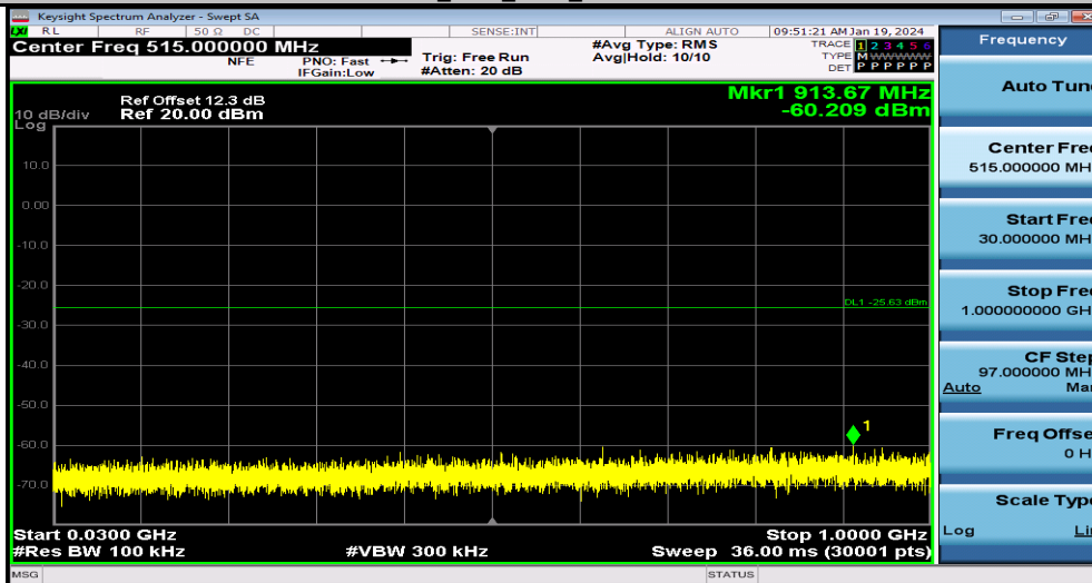
11B_Ant1_2462_30~1000
