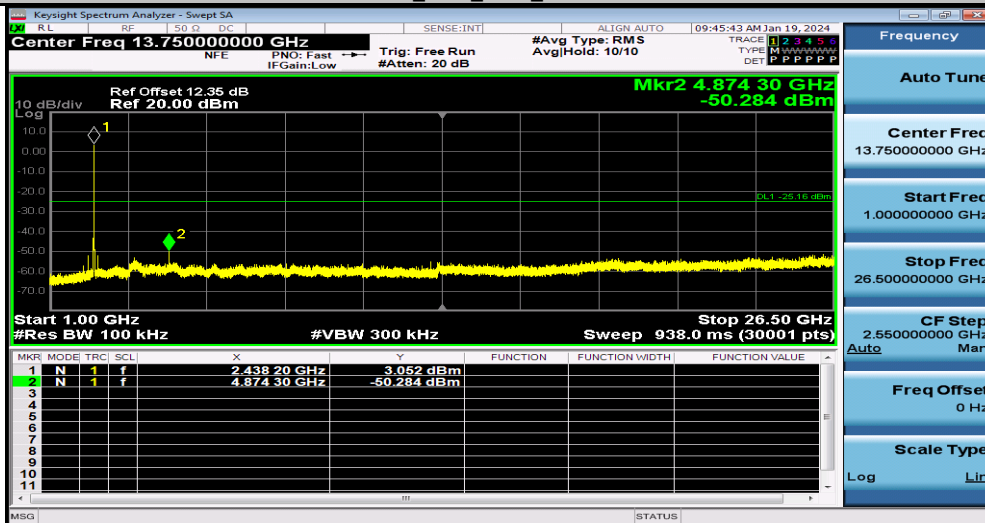
11B_Ant1_2437_1000~26500
