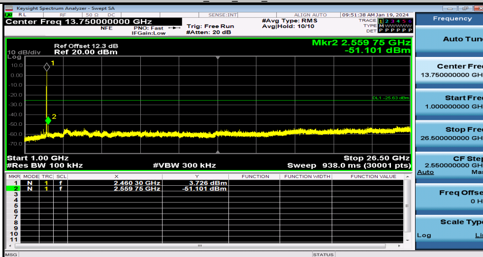
11B_Ant1_2462_1000~26500
