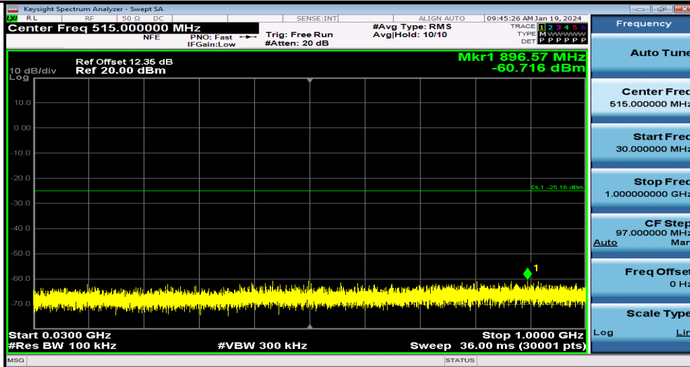
11B_Ant1_2437_30~1000
