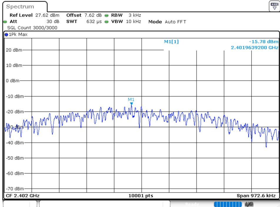
PSD NVNT GFSK 2402MHz Ant1
