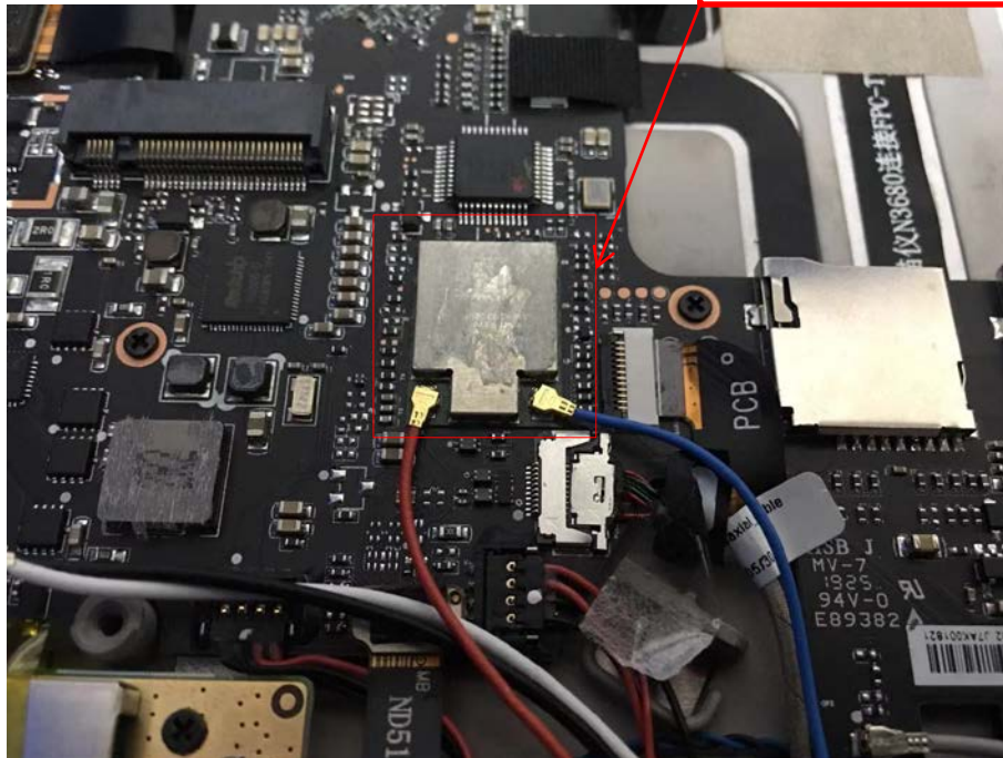
BT/WIFI Module
