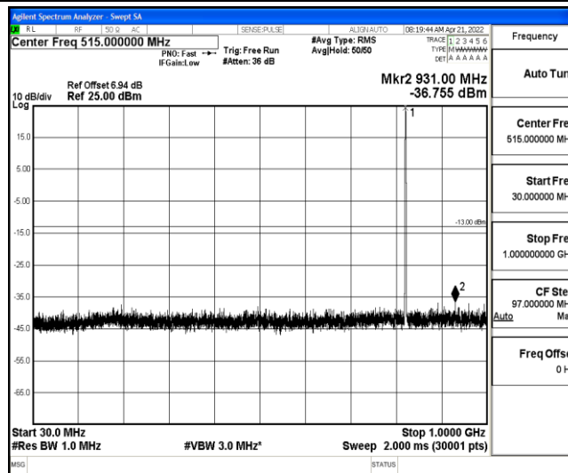
Band26-10MHz-QPSK-26840-1-0-Low-30-1000--36.76-PASS
