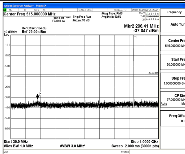
Band26-3MHz-QPSK-26915-1-0-Low-30-1000--37.05-PASS
