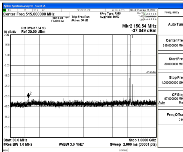
Band26-15MHz-QPSK-26865-1-0-Low-30-1000--37.05-PASS
