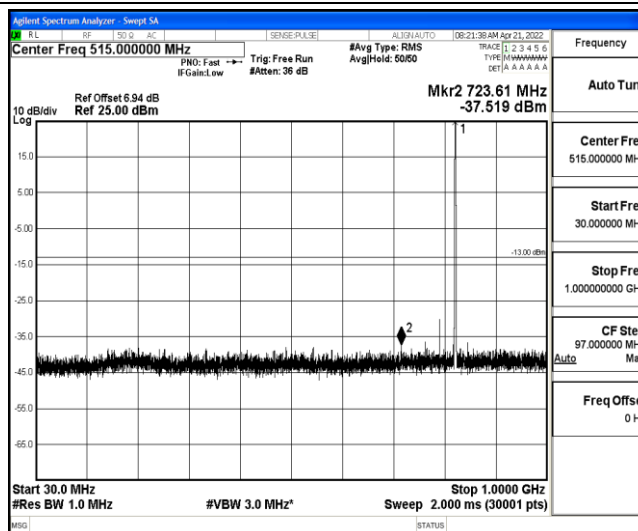
Band26-10MHz-16QAM-26840-1-0-Low-30-1000--37.52-PASS
