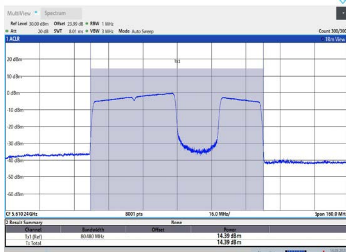
11BE80MIMO_Ant3_5610_484+242_OFDMA_4
