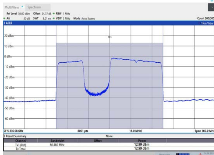
11BE80MIMO_Ant2_5530_484+242_OFDMA_3
