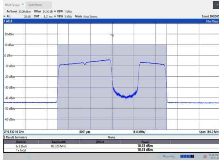
11BE80MIMO_Ant3_5530_484+242_OFDMA_3
