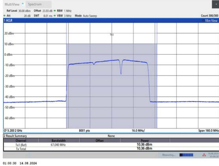
11BE80MIMO_Ant3_5290_484+242_OFDMA_4
