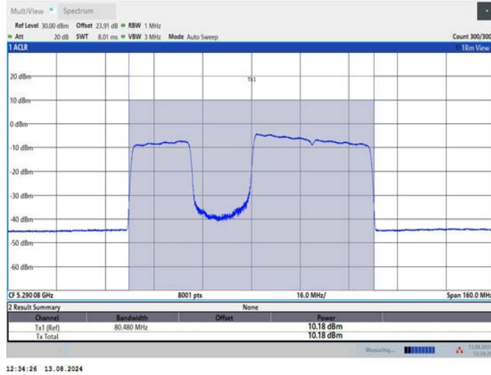
11BE80MIMO_Ant2_5290_484+242_OFDMA_2
