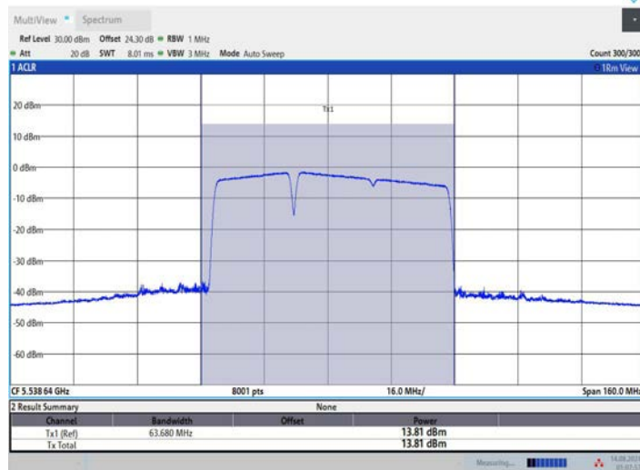
11BE80MIMO_Ant3_5530_484+242_OFDMA_2
