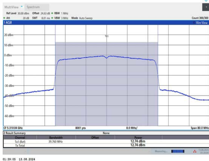
11BE40MIMO_Ant2_5310
