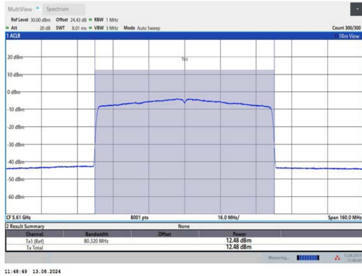
11BE80MIMO_Ant2_5610
