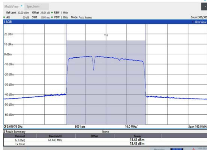
11BE80MIMO_Ant1_5610_484+242_OFDMA_2
