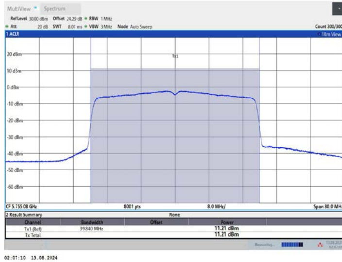
11BE40MIMO_Ant2_5755
