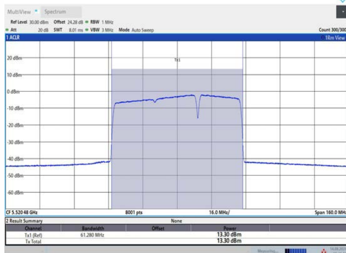
11BE80MIMO_Ant2_5530_484+242_OFDMA_1
