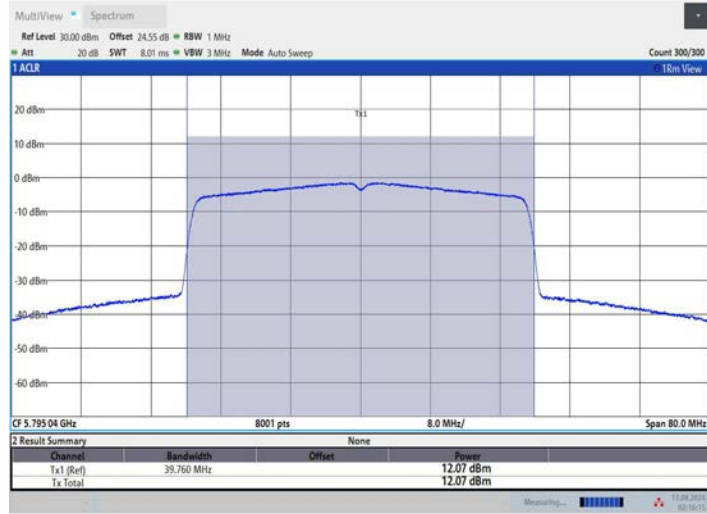
11BE40MIMO_Ant3_5795
