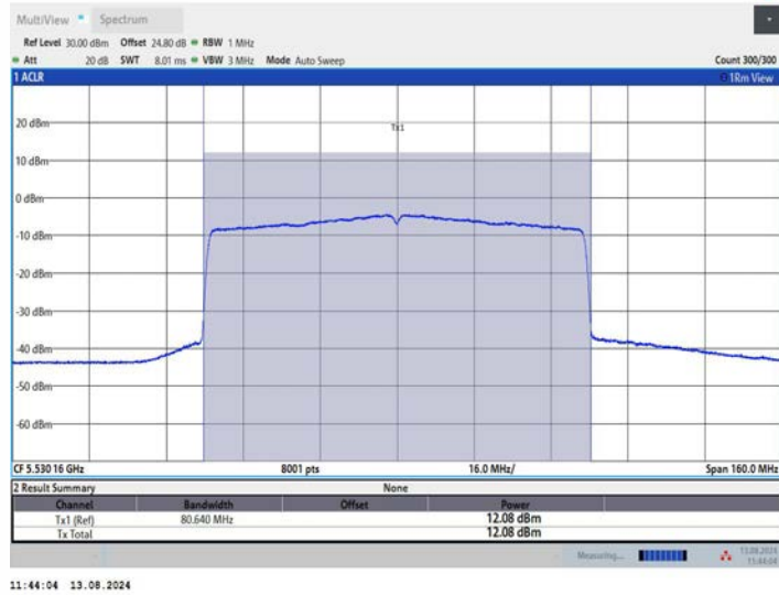
11BE80MIMO_Ant3_5530
