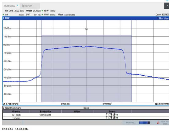
11BE40MIMO_Ant3_5755
