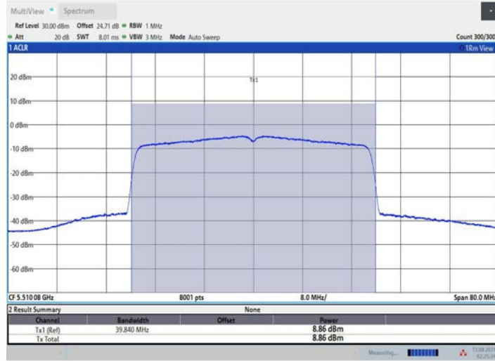
11BE40MIMO_Ant1_5510
