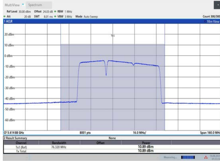
11BE80MIMO_Ant3_5610_484+242_OFDMA_1
