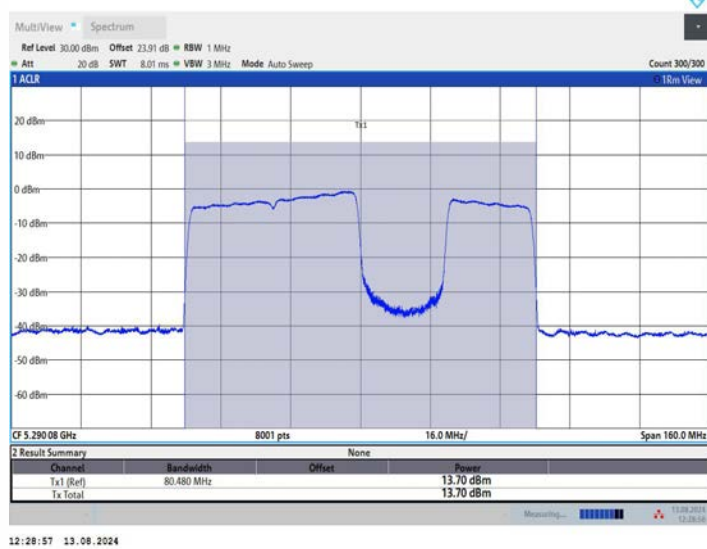
11BE80MIMO_Ant2_5290_484+242_OFDMA_4
