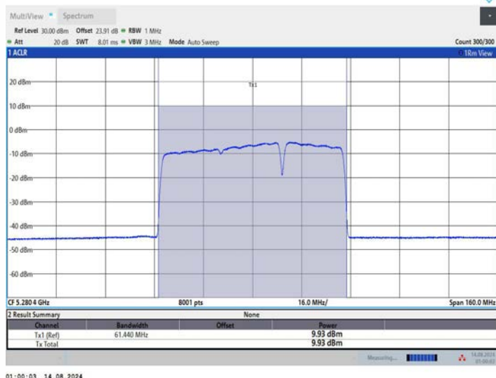
11BE80MIMO_Ant2_5290_484+242_OFDMA_4
