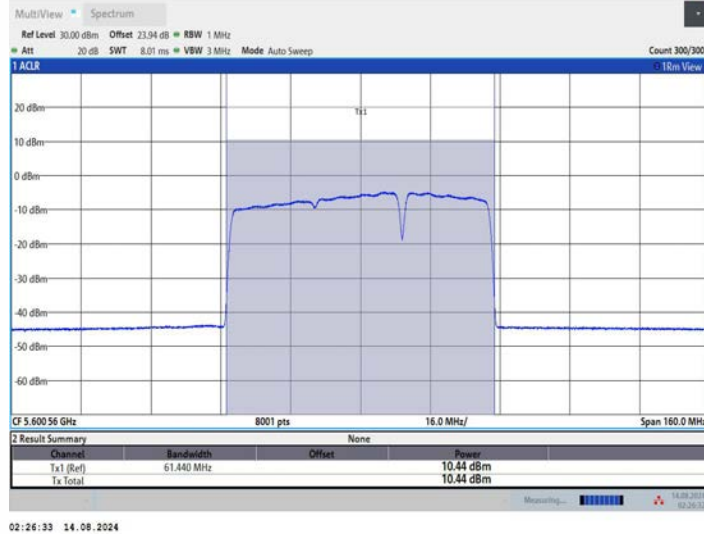
11BE80MIMO_Ant2_5610_484+242_OFDMA_4
