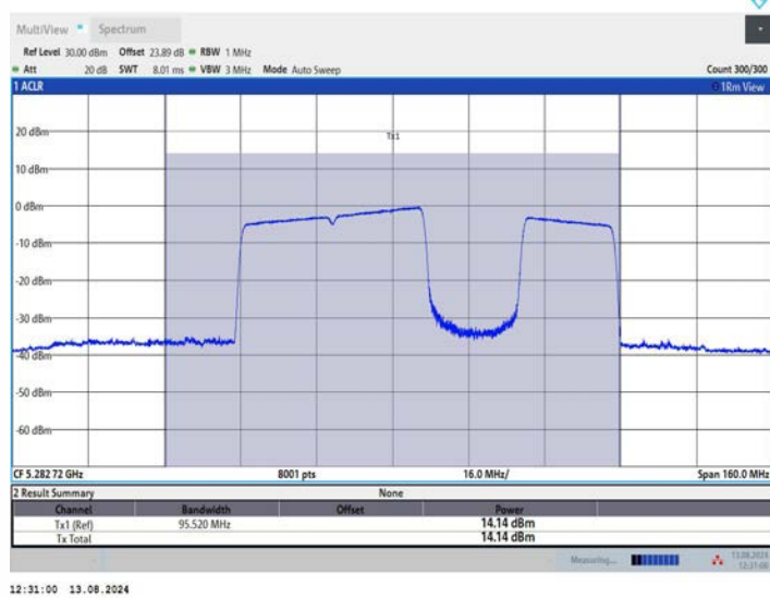
11BE80MIMO_Ant3_5290_484+242_OFDMA_4
