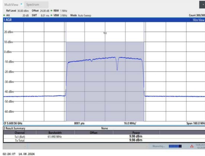
11BE80MIMO_Ant1_5610_484+242_OFDMA_4
