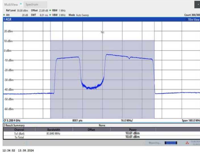
11BE80MIMO_Ant3_5290_484+242_OFDMA_2
