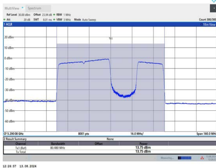
11BE80MIMO_Ant1_5290_484+242_OFDMA_4
