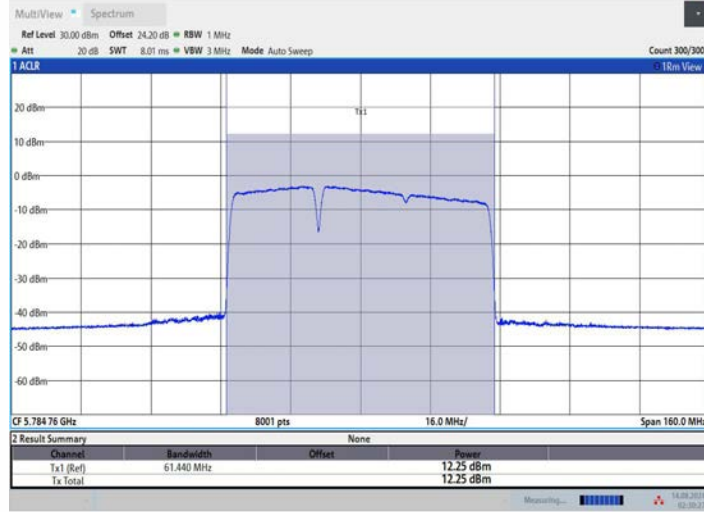
11BE80MIMO_Ant1_5775_484+242_OFDMA_2
