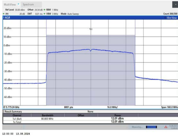
11BE80MIMO_Ant3_5775
