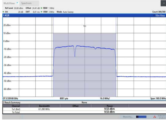
11BE80MIMO_Ant2_5530_484+242_OFDMA_1
