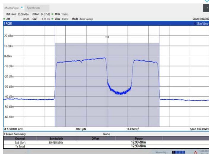
11BE80MIMO_Ant2_5530_484+242_OFDMA_4
