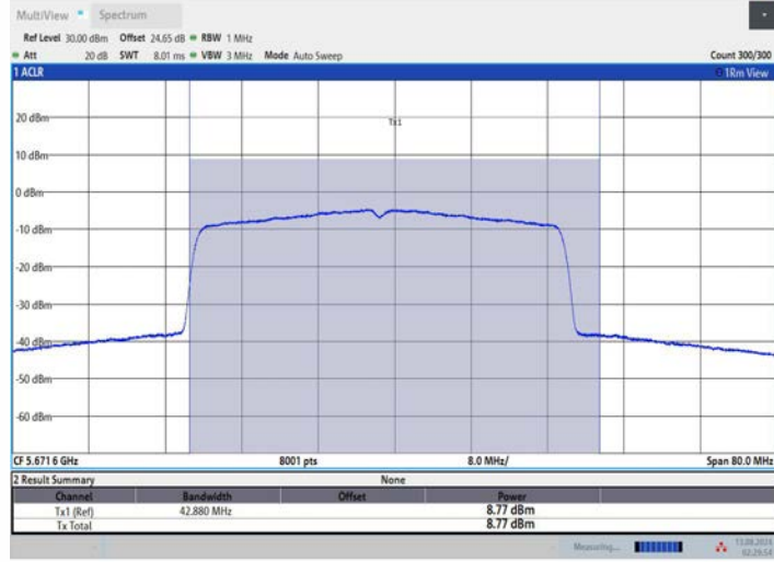
11BE40MIMO_Ant3_5670
