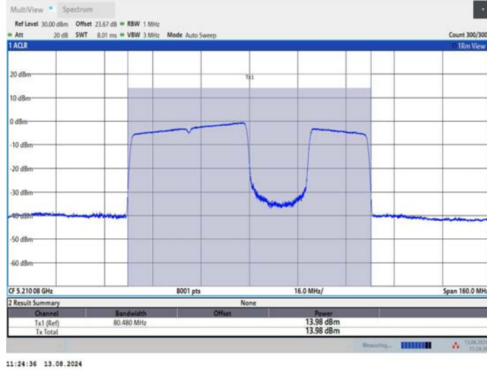
11BE80MIMO_Ant3_5210_484+242_OFDMA_4
