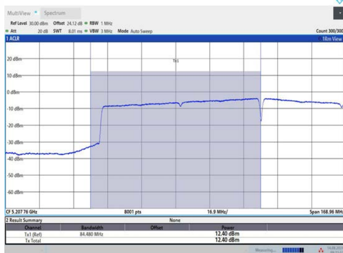
11BE160MIMO_Ant1_5250_UNII-2A
