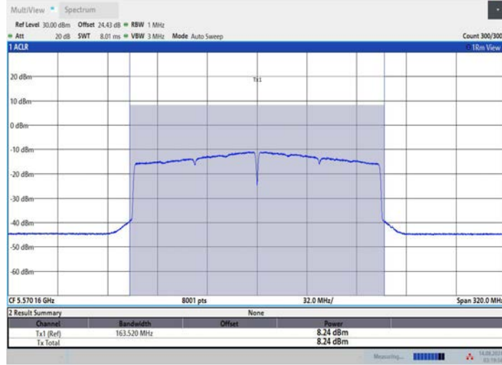
11BE160MIMO_Ant2_5570
