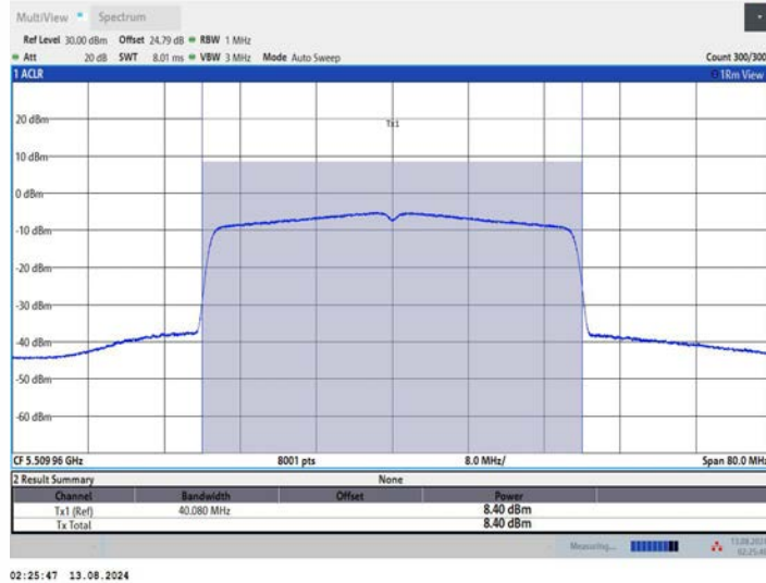
11BE40MIMO_Ant2_5510
