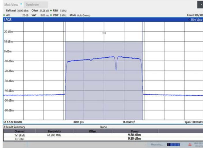
11BE80MIMO_Ant1_5530_484+242_OFDMA_4
