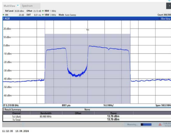
11BE80MIMO_Ant2_5210_484+242_OFDMA_3
