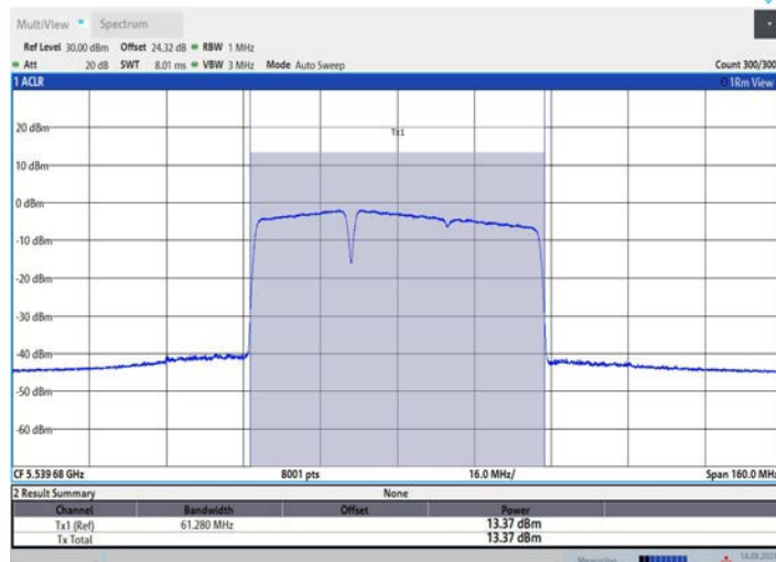
11BE80MIMO_Ant1_5530_484+242_OFDMA_2
