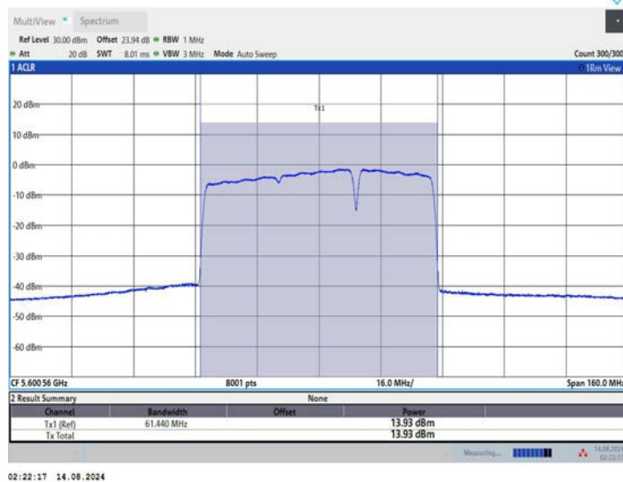
11BE80MIMO_Ant3_5610_484+242_OFDMA_1
