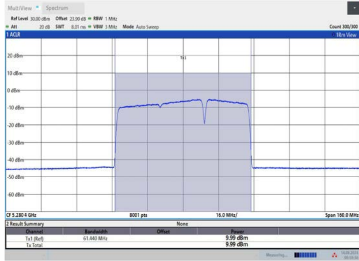
11BE80MIMO_Ant1_5290_484+242_OFDMA_4
