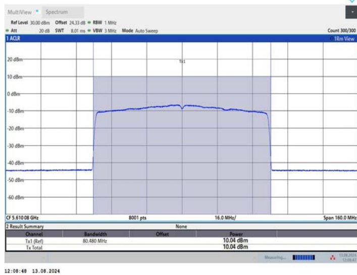
11BE80MIMO_Ant3_5610
