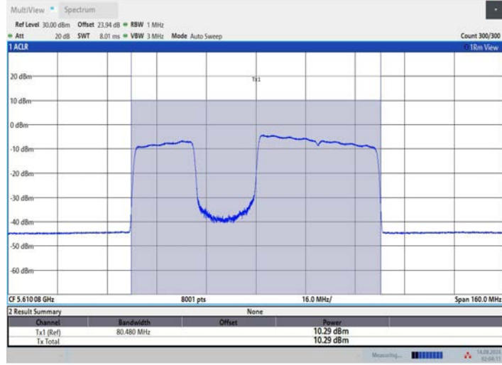
11BE80MIMO_Ant2_5610_484+242_OFDMA_2
