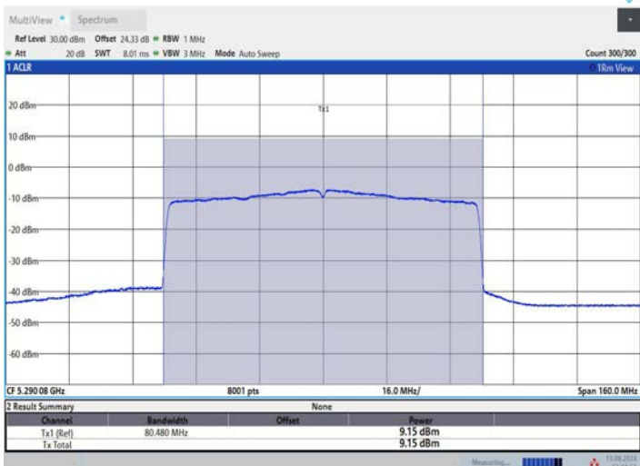
11BE80MIMO_Ant1_5290
