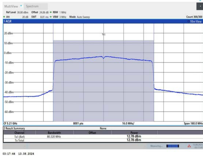
11BE80MIMO_Ant3_5210
