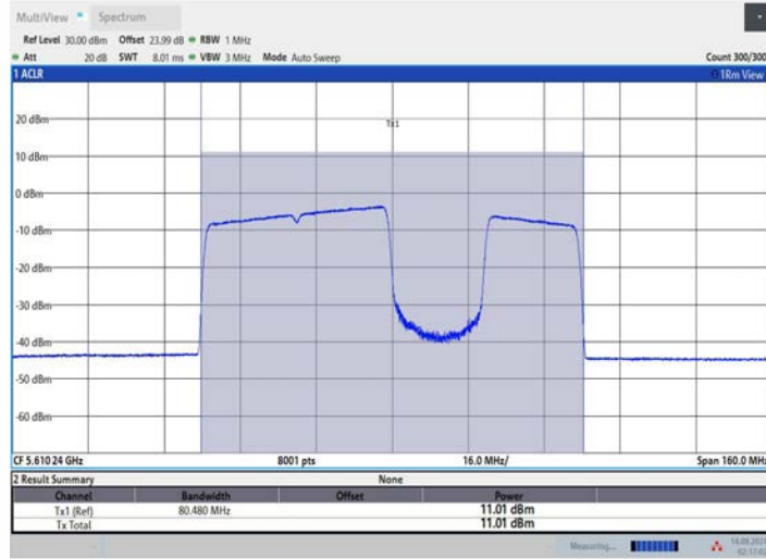
11BE80MIMO_Ant3_5610_484+242_OFDMA_3
