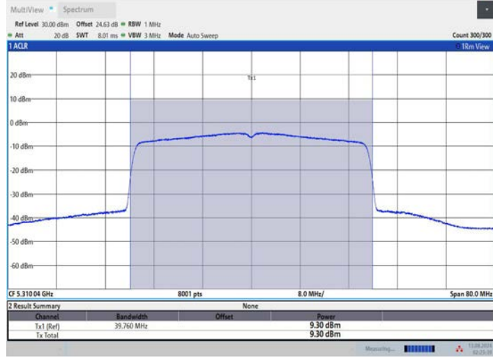
11BE40MIMO_Ant1_5310
