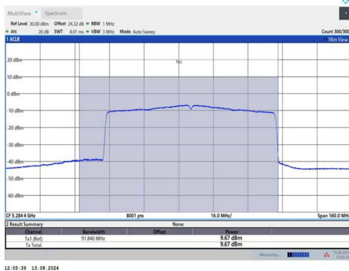
11BE80MIMO_Ant3_5290
