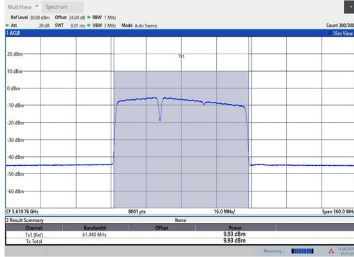
11BE80MIMO_Ant1_5610_484+242_OFDMA_1
