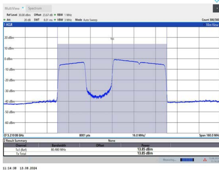
11BE80MIMO_Ant3_5210_484+242_OFDMA_3
