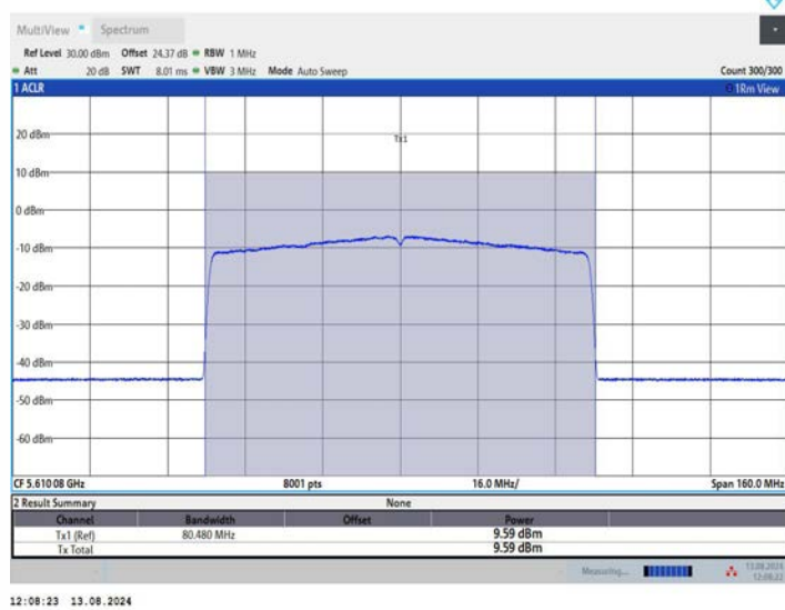
11BE80MIMO_Ant2_5610
