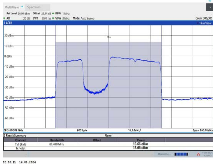
11BE80MIMO_Ant2_5610_484+242_OFDMA_3
