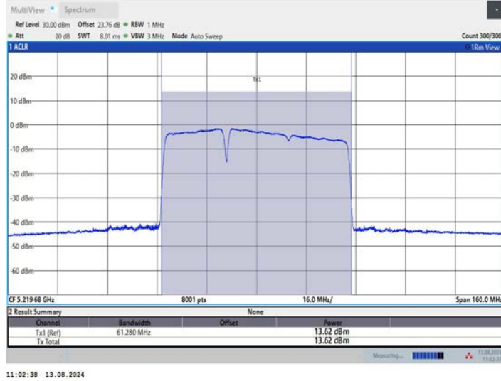
11BE80MIMO_Ant2_5210_484+242_OFDMA_2
