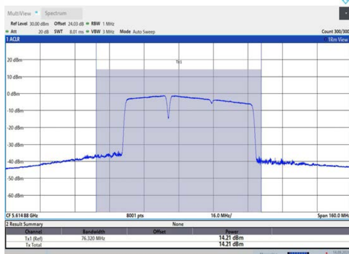
11BE80MIMO_Ant3_5610_484+242_OFDMA_2
