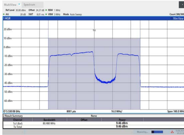
11BE80MIMO_Ant2_5530_484+242_OFDMA_3
