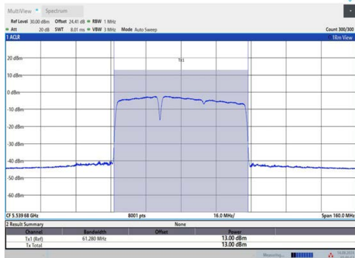
11BE80MIMO_Ant2_5530_484+242_OFDMA_2
