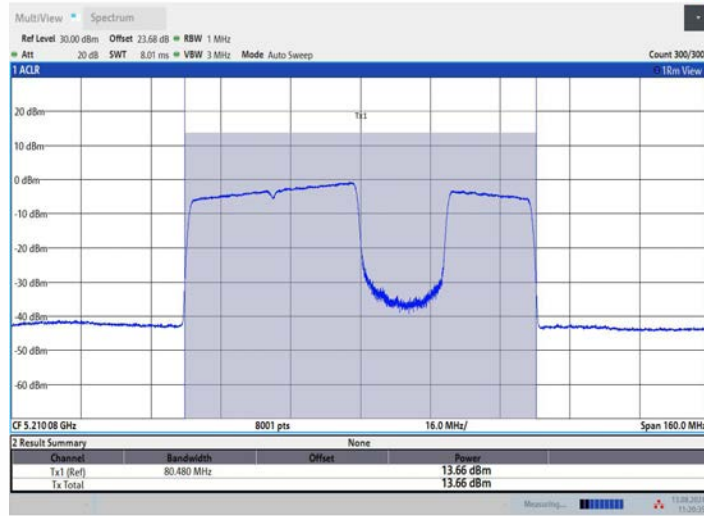
11BE80MIMO_Ant1_5210_484+242_OFDMA_4
