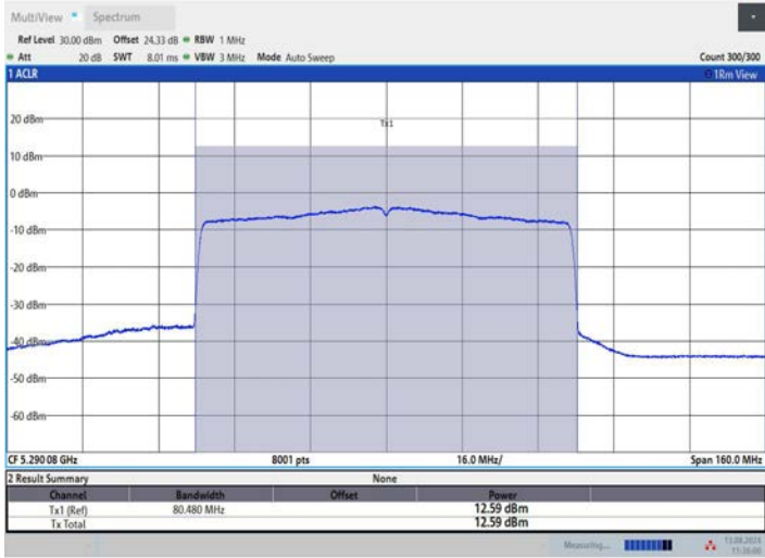
11BE80MIMO_Ant2_5290
