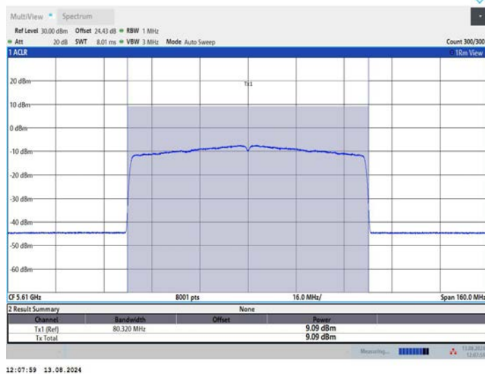
11BE80MIMO_Ant1_5610
