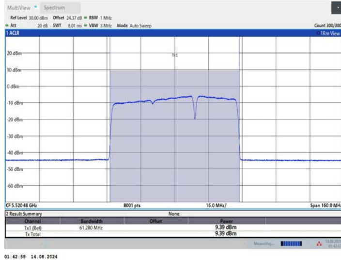
11BE80MIMO_Ant2_5530_484+242_OFDMA_4
