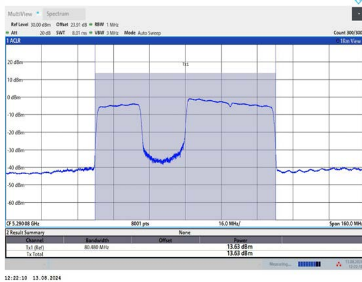
11BE80MIMO_Ant2_5290_484+242_OFDMA_3
