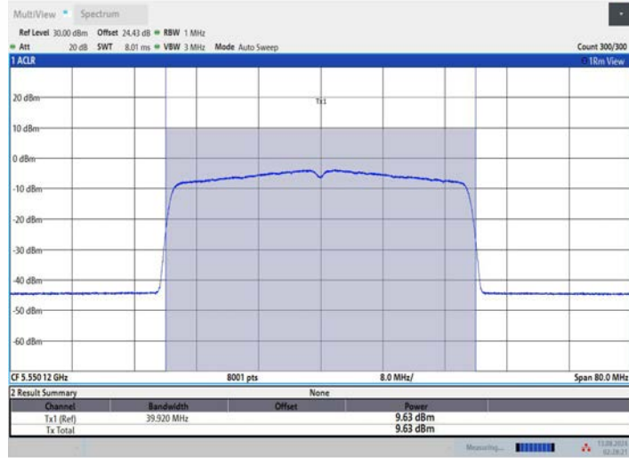
11BE40MIMO_Ant3_5550
