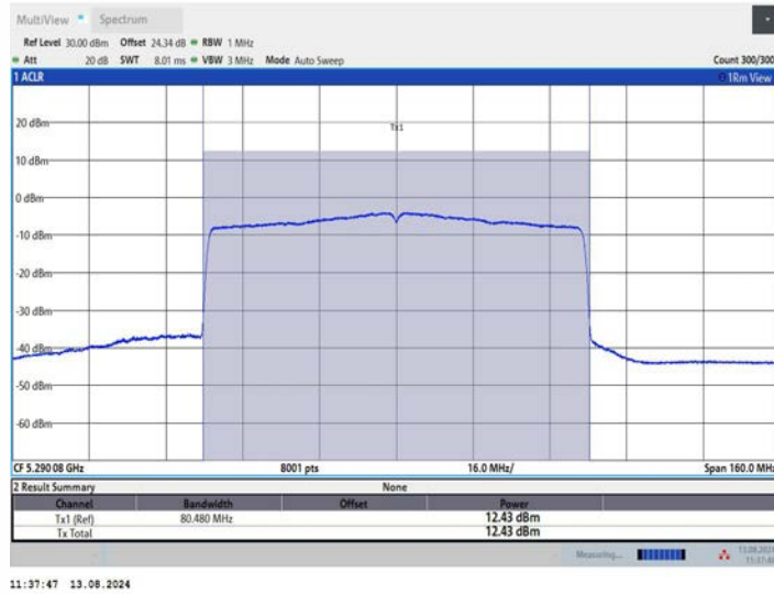
11BE80MIMO_Ant3_5290
