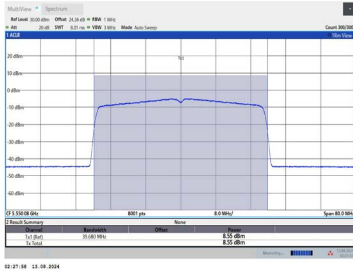
11BE40MIMO_Ant2_5550
