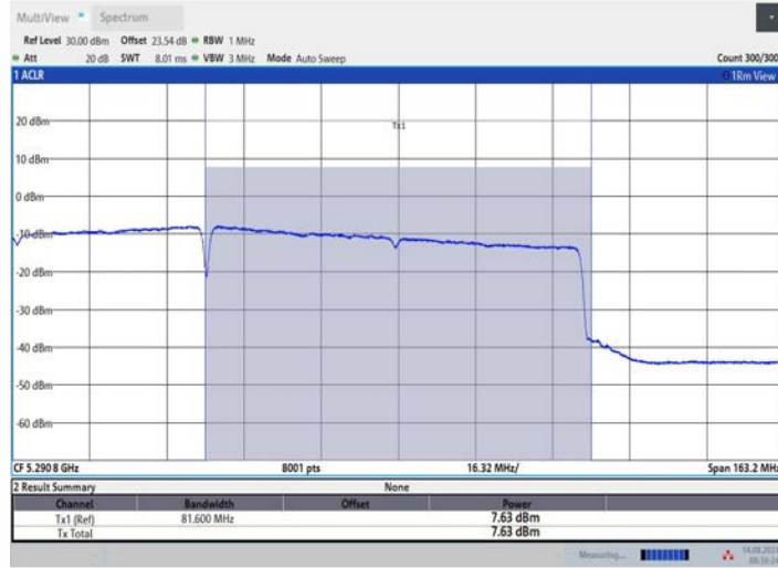
11BE160MIMO_Ant3_5250_UNII-2A
