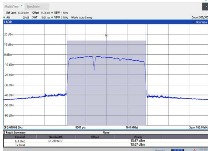
11BE80MIMO_Ant2_5610_484+242_OFDMA_2
