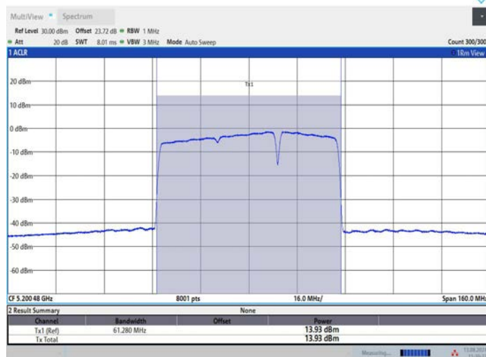
11BE80MIMO_Ant3_5210_484+242_OFDMA_1
