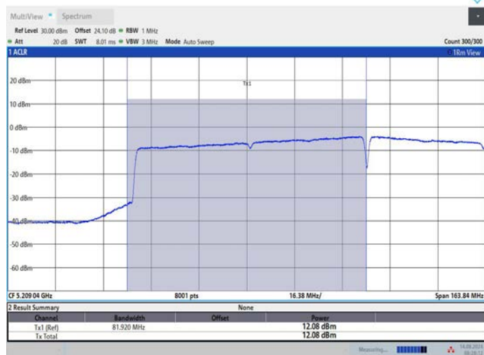
11BE160MIMO_Ant2_5250_UNII-1
