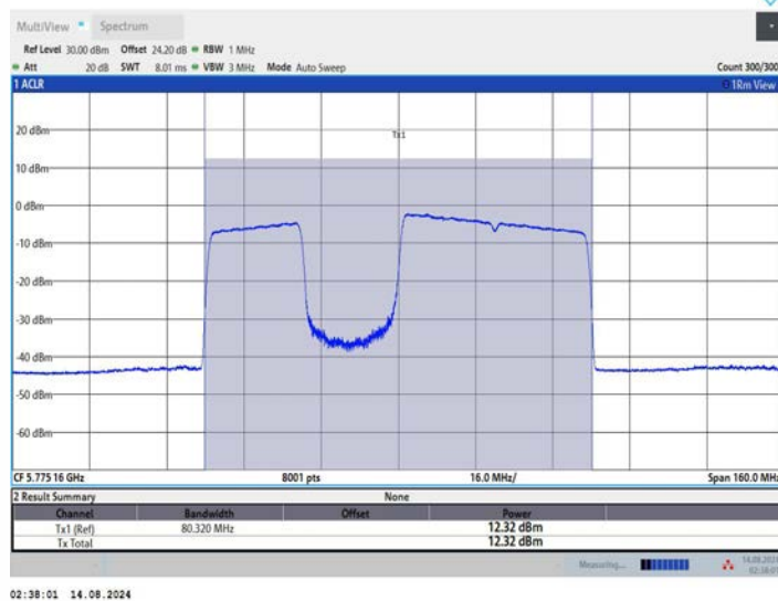
11BE80MIMO_Ant1_5775_484+242_OFDMA_3
