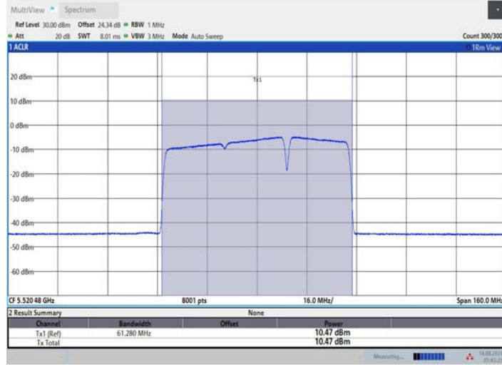
11BE80MIMO_Ant3_5530_484+242_OFDMA_4
