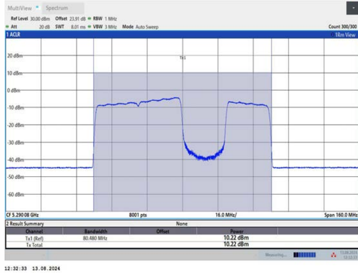
11BE80MIMO_Ant2_5290_484+242_OFDMA_3
