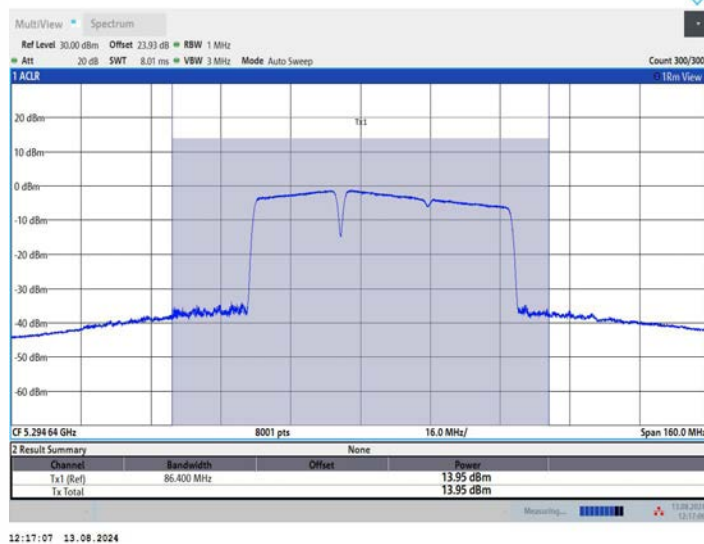
11BE80MIMO_Ant3_5290_484+242_OFDMA_2
