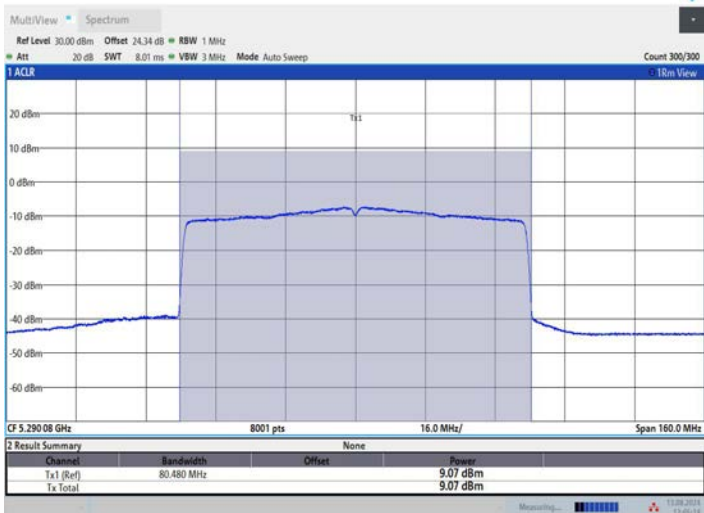
11BE80MIMO_Ant2_5290
