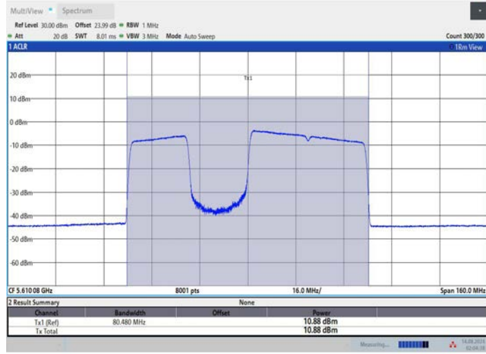
11BE80MIMO_Ant3_5610_484+242_OFDMA_2
