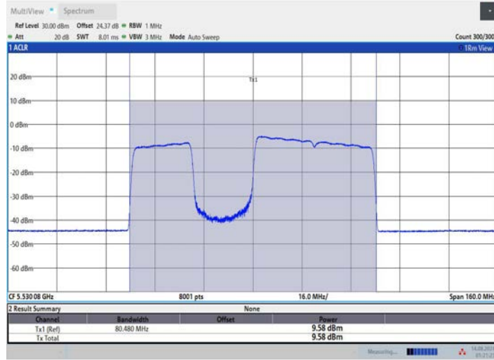
11BE80MIMO_Ant2_5530_484+242_OFDMA_2
