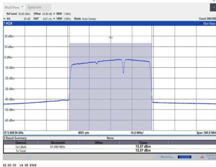
11BE80MIMO_Ant2_5610_484+242_OFDMA_1
