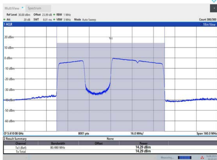
11BE80MIMO_Ant3_5610_484+242_OFDMA_3
