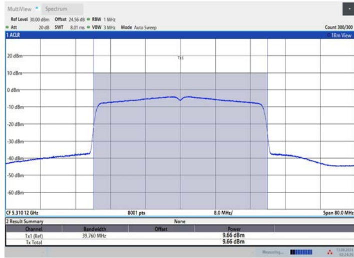
11BE40MIMO_Ant3_5310
