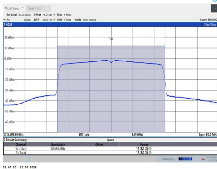
11BE40MIMO_Ant3_5510
