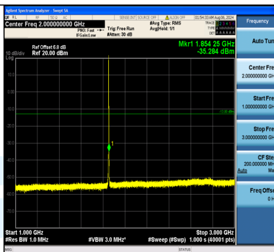
Band2 1.4MHz QPSK 18607 6RB#0 1000~3000 1000~3000
