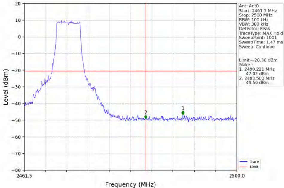
5M_HCH_2469.5MHz_Ant0_NTNV
