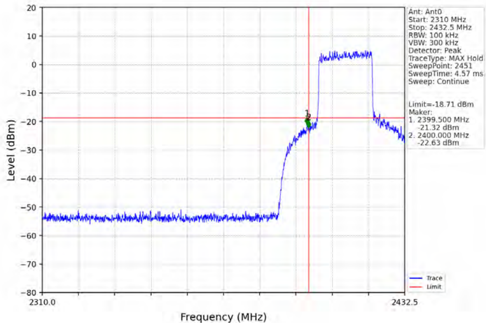
20M_LCH_2412.5MHz_Ant0_NTNV
