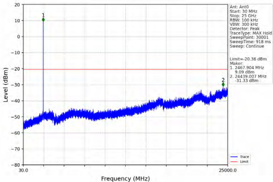
5M_HCH_2469.5MHz_Ant0_NTNV
