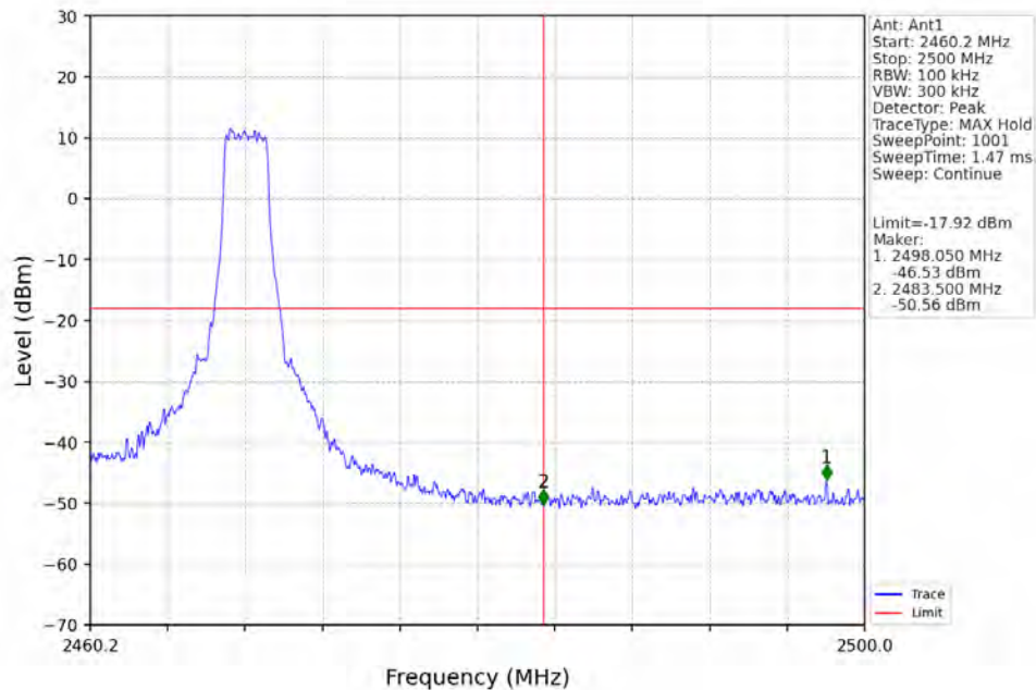
3M_HCH_2468.2MHz_Ant1_NTNV
