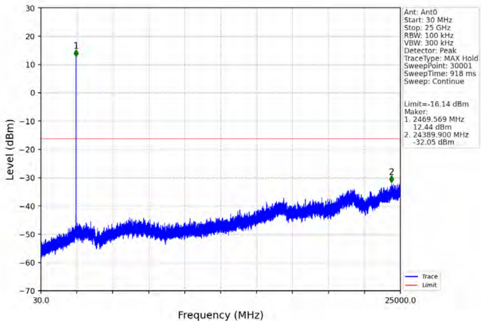
1.4M_HCH_2469.12MHz_Ant0_NTNV
