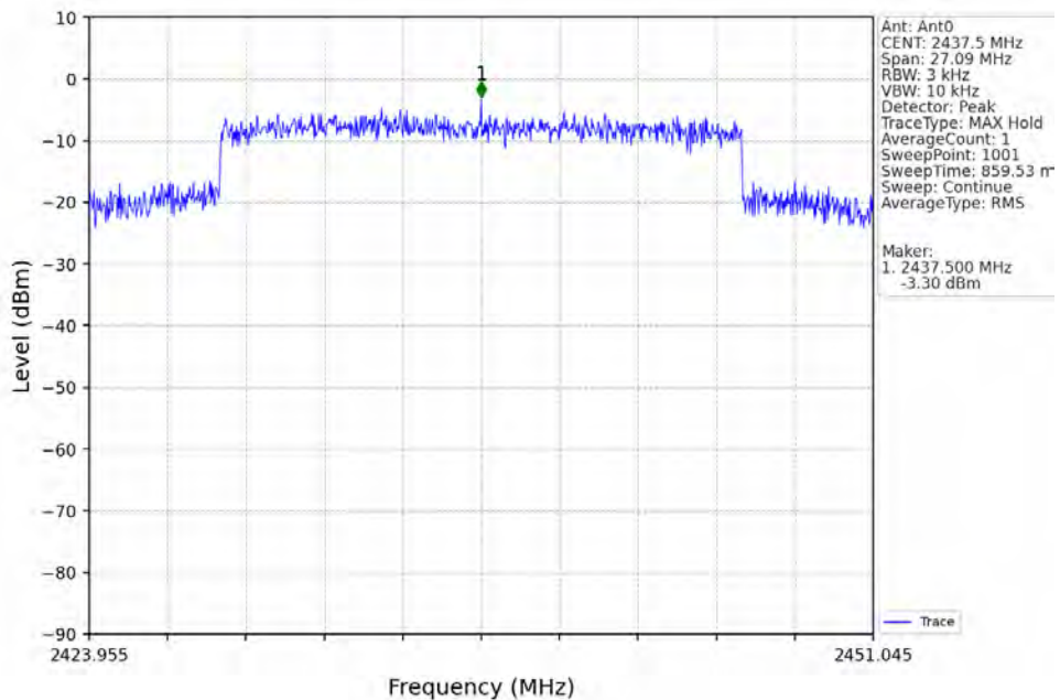
20M_MCH_2437.5MHz_Ant0_NTNV
