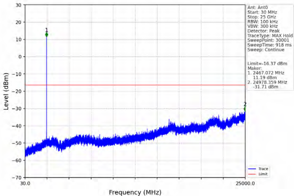
3M_HCH_2468.2MHz_Ant0_NTNV
