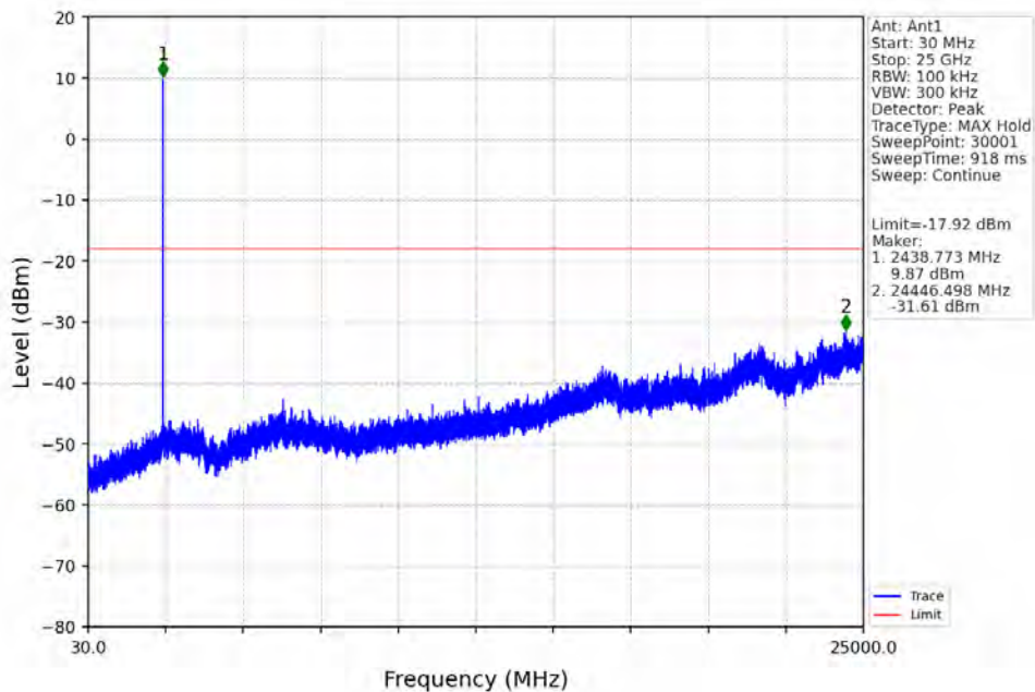
3M_MCH_2438.5MHz_Ant1_NTNV
