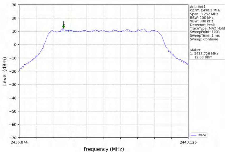
3M_MCH_2438.5MHz_Ant1_NTNV
