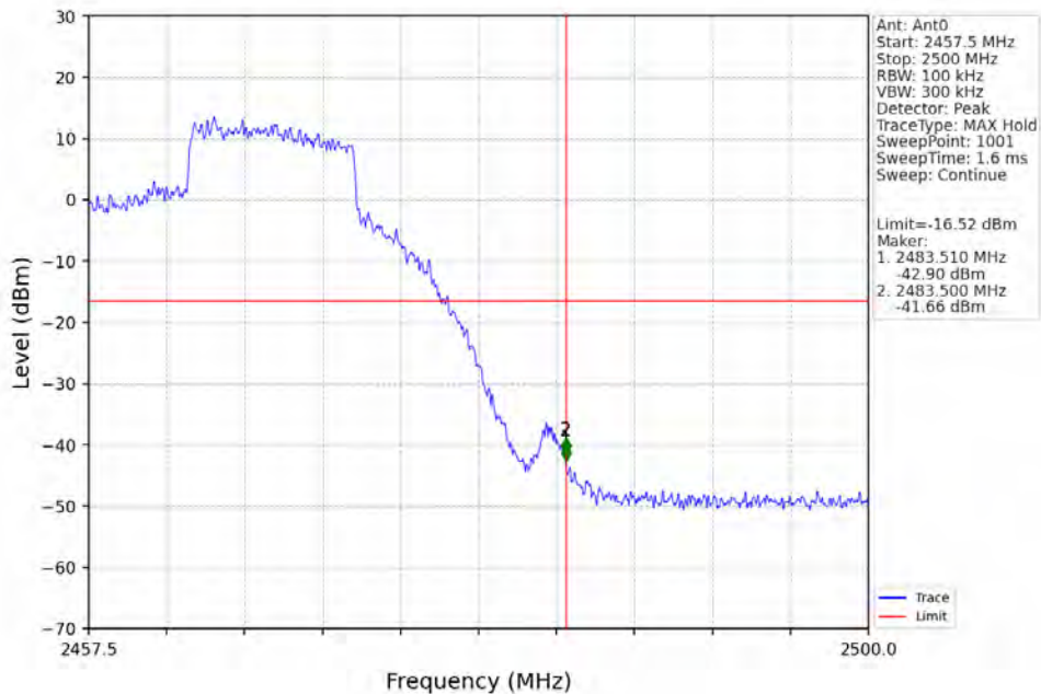
10M_HCH_2467.5MHz_Ant0_NTNV
