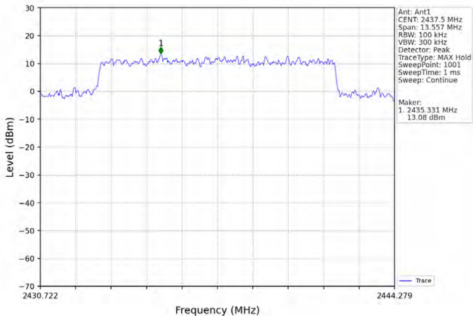
10M_MCH_2437.5MHz_Ant1_NTNV
