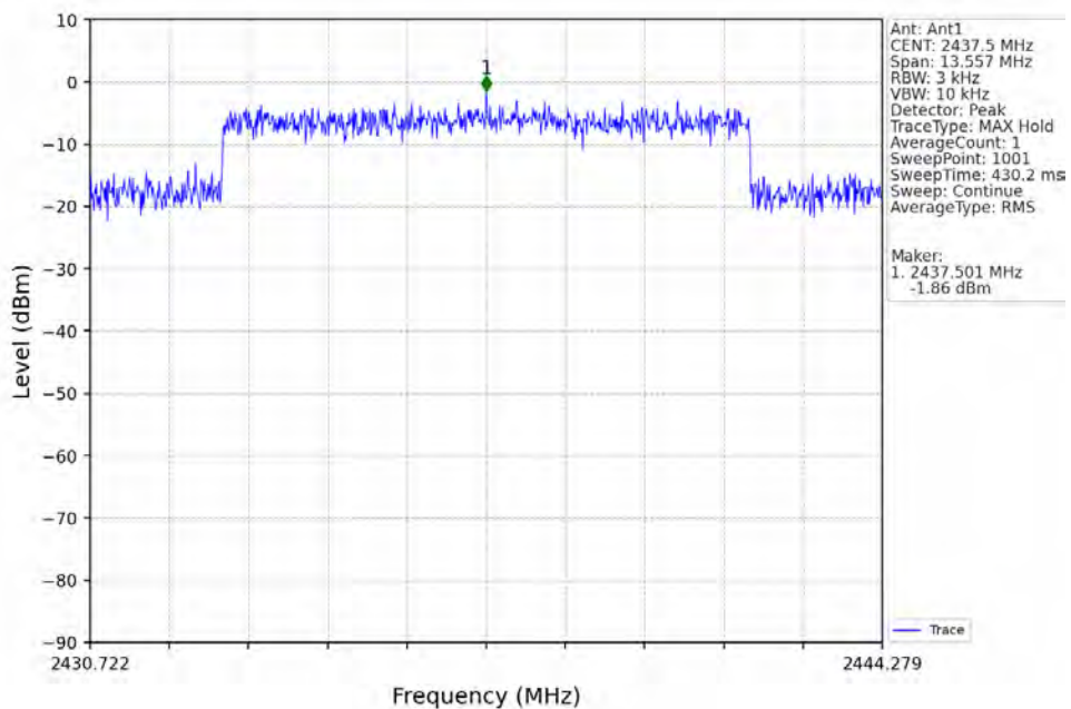
10M_MCH_2437.5MHz_Ant1_NTNV
