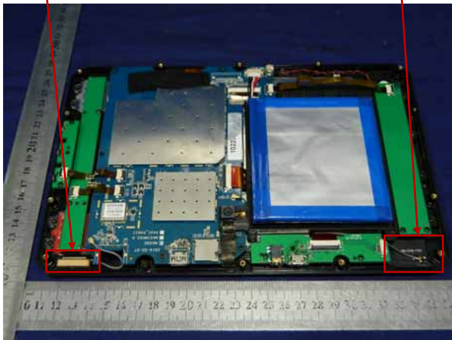
GPS Antenna
