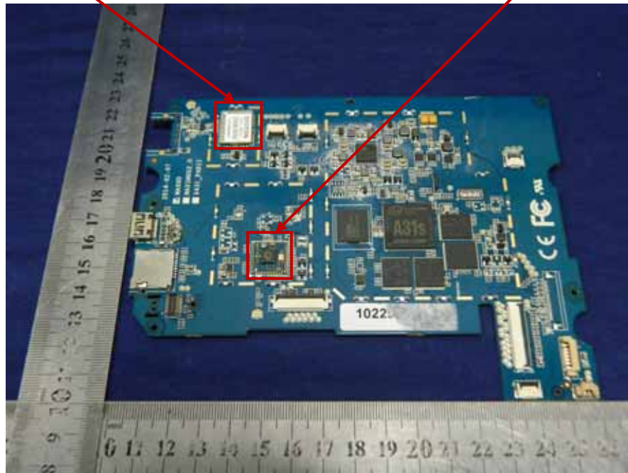
GPS Module
