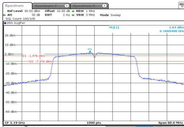
n40_5190MHz_Chain 0
