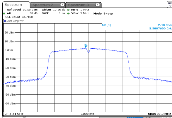
n40_5510MHz_Chain 0
