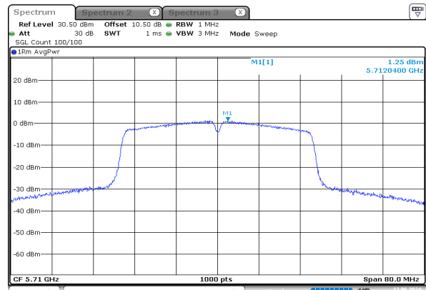
n40_5710MHz_Chain 0
