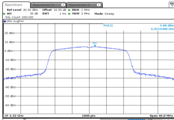
n20_5320MHz_Chain 0
