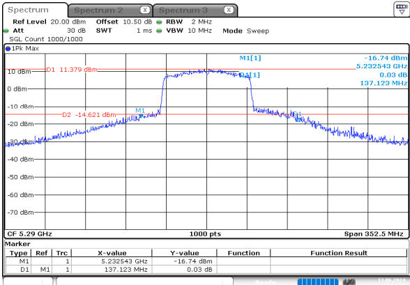
ac80_5290MHz_Chain 0
