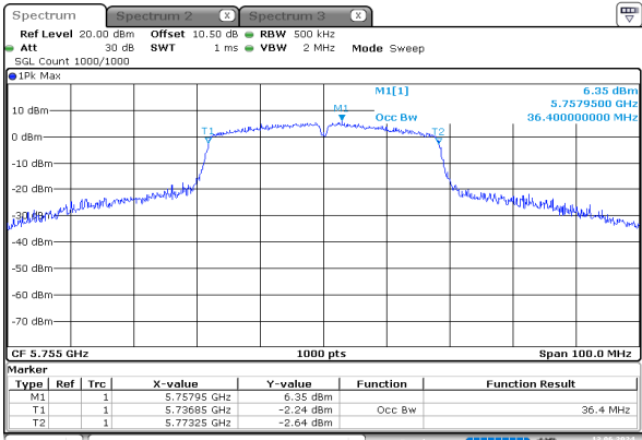
n40_5755MHz_Chain 0
