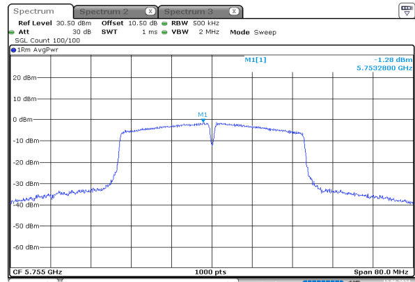
n40_5755MHz_Chain 0
