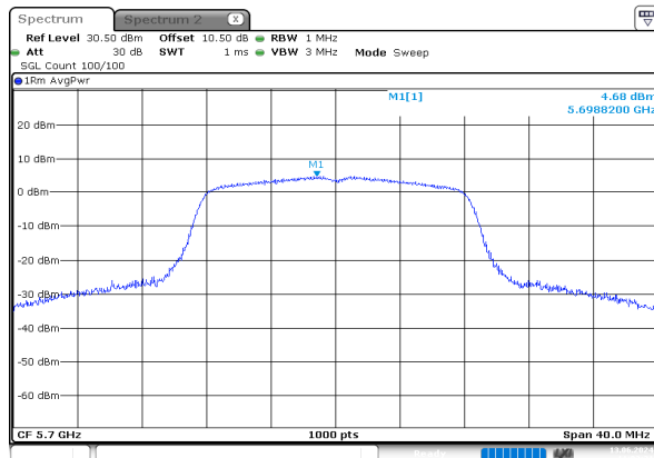
a_5700MHz_Chain 0
