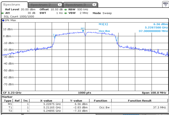
n40_5230MHz_Chain 0
