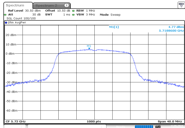
a_5720MHz_Chain 0
