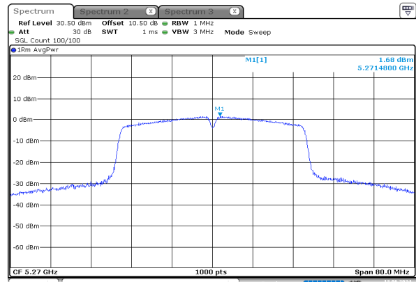
n40_5270MHz_Chain 0
