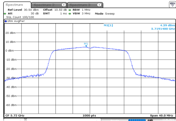
n20_5720MHz_Chain 0
