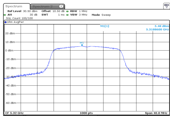
a_5320MHz_Chain 0
