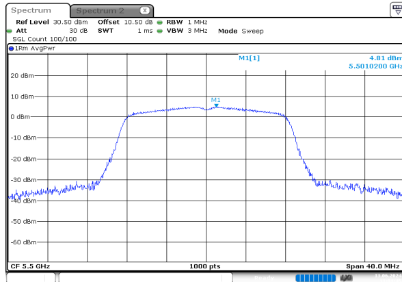
a_5500MHz_Chain 0
