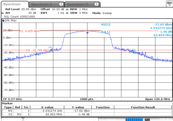
n40_5270MHz_Chain 0
