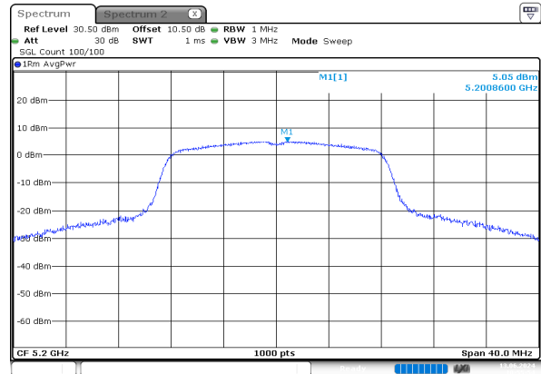
a_5200MHz_Chain 0
