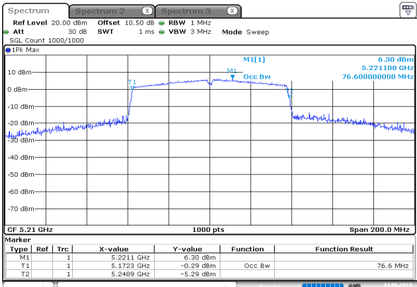
ac80_5210MHz_Chain 0
