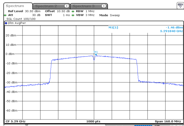
ac80_5290MHz_Chain 0
