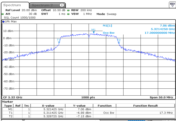
a_5320MHz_Chain 0
