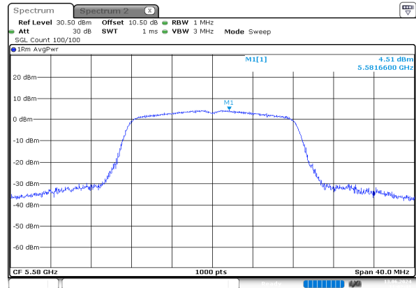
a_5580MHz_Chain 0
