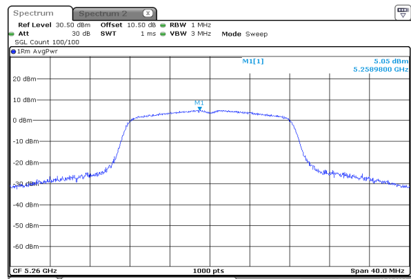
a_5260MHz_Chain 0
