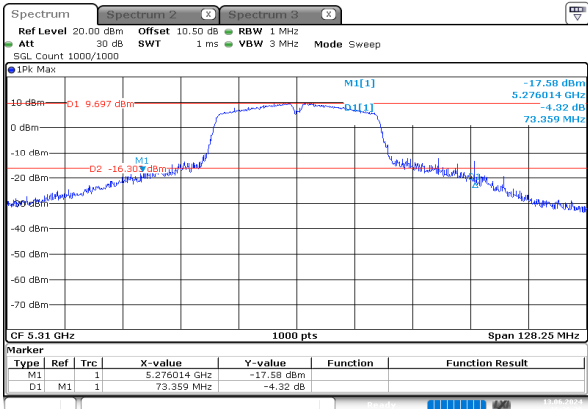
n40_5310MHz_Chain 0
