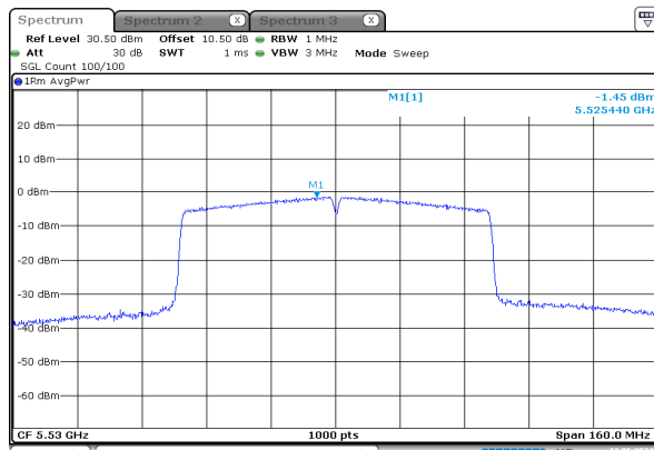
ac80_5530MHz_Chain 0
