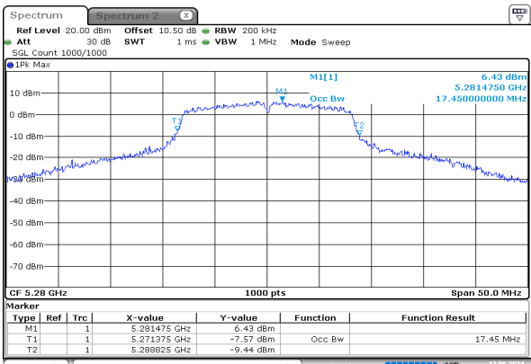
a_5280MHz_Chain 0
