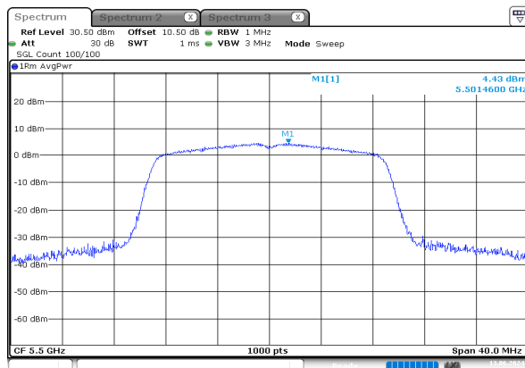
n20_5500MHz_Chain 0
