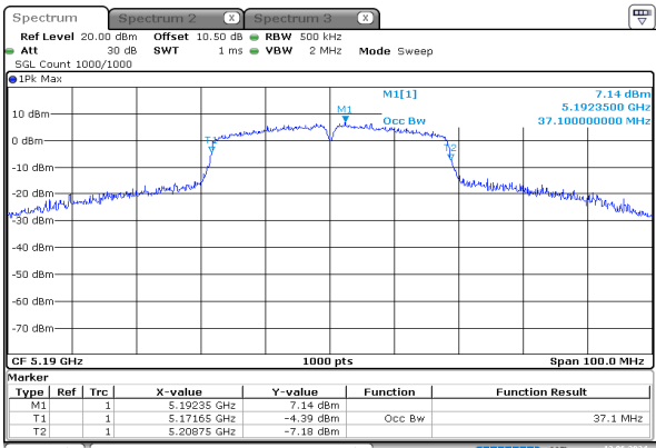
n40_5190MHz_Chain 0
