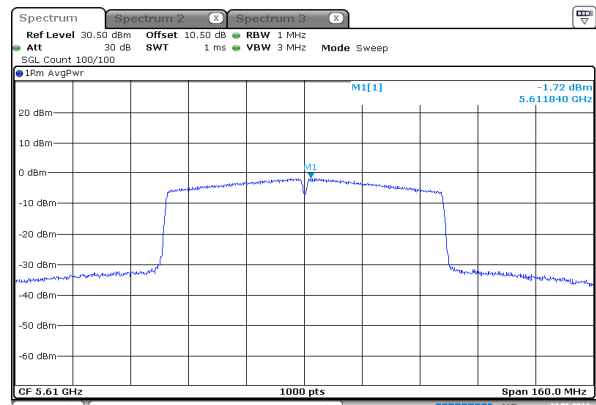
ac80_5610MHz_Chain 0
