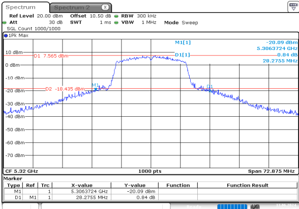
n20_5320MHz_Chain 0
