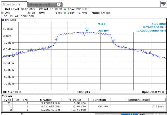
a_5260MHz_Chain 0
