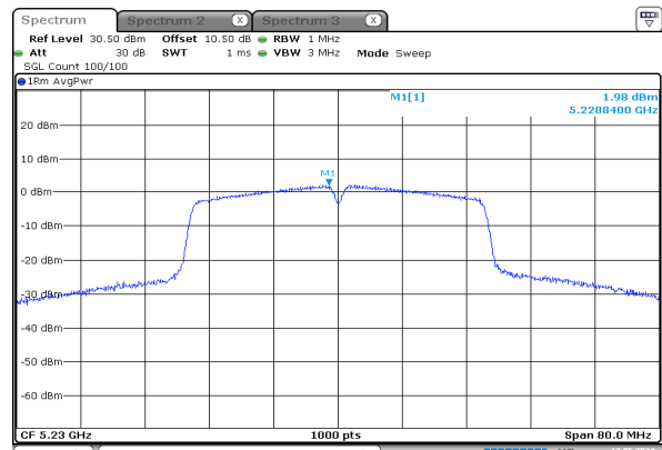
n40_5230MHz_Chain 0
