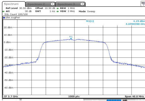
n20_5700MHz_Chain 0
