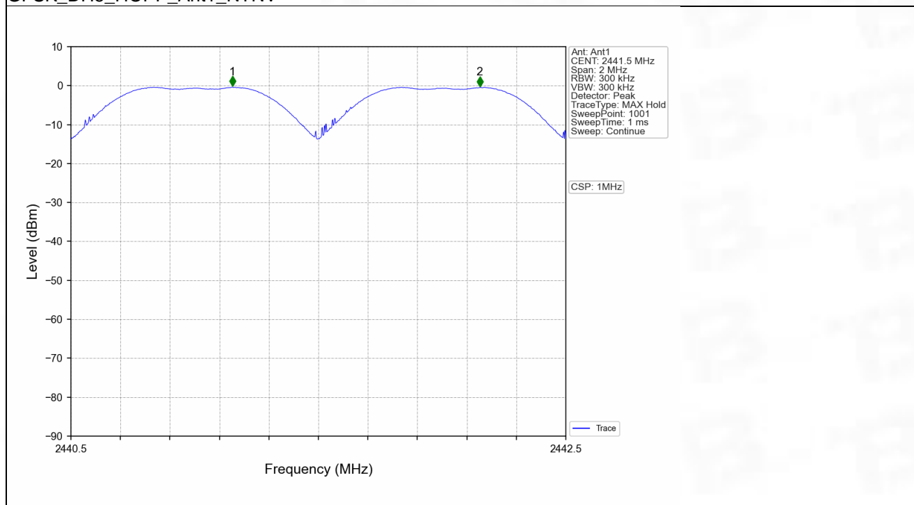
Pi/4DQPSK_2DH5_HOPP_Ant1_NTNV
