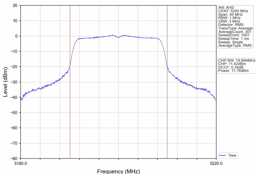
802.11n(HT20)_MCH_5200MHz_Ant2_NTNV
