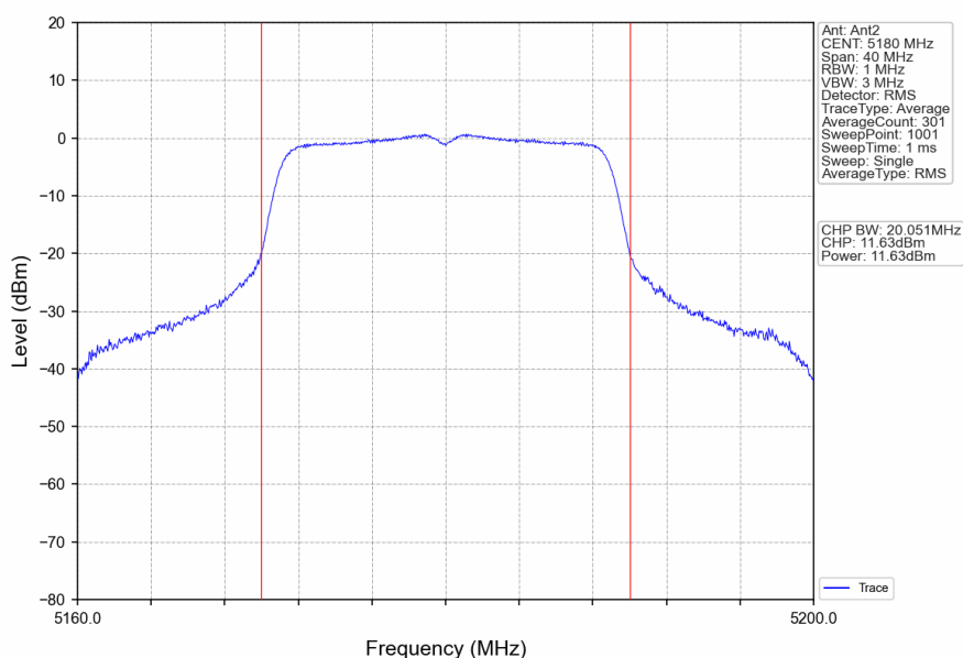
802.11n(HT20)_LCH_5180MHz_Ant2_NTNV
