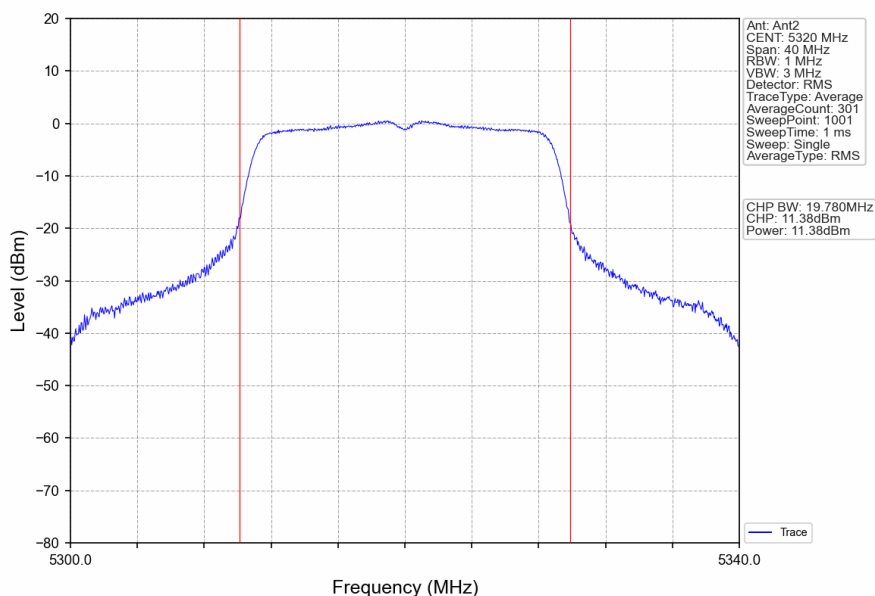
802.11n(HT20)_HCH_5320MHz_Ant2_NTNV
