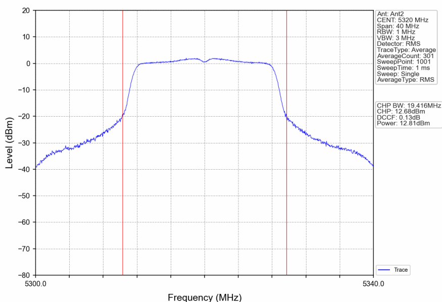
802.11a_HCH_5320MHz_Ant2_NTNV
