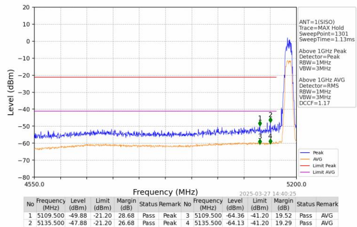
802.11a LCH 5180MHz Ant1 NTN
