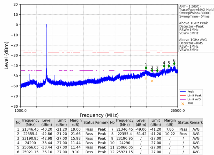
802.11a LCH 5180MHz Ant1 NTN
