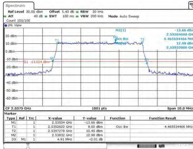
Band41_5MHz_QPSK_40065_25RB#0
