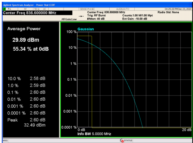
GSM 850
