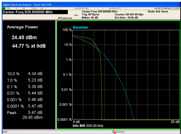
EGPRS 850
