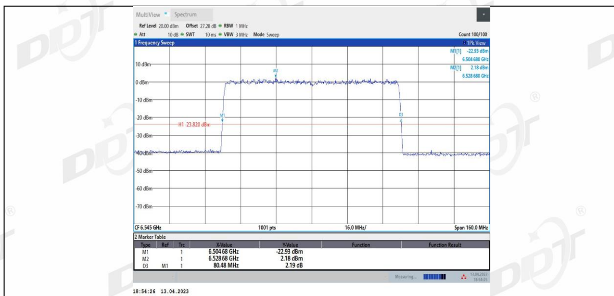
11AX80MIMO_Ant4_6545
