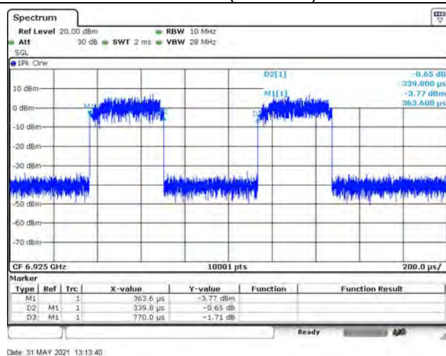
802.11ax (160MHz)
