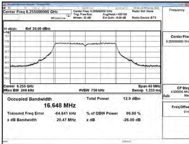
802.11a / Ant. 3 / 6255 MHz (U-NII-5)
