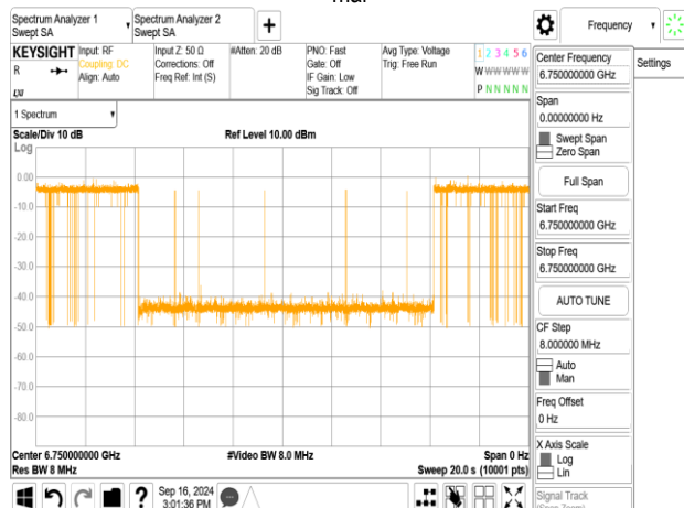
802.11be_320MHz_CF 6905MHz_Interference_6750MHz_-80.69dBm_ON
