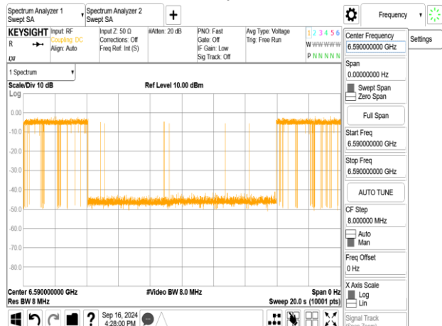
802.11be_320MHz_CF 6745MHz_Interference_6590MHz_-80.05dBm_ON
