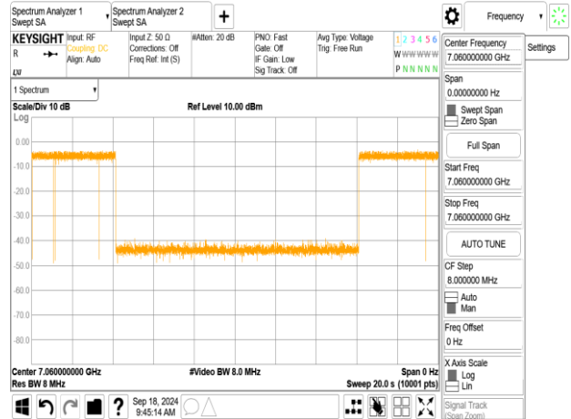
802.11be_320MHz_CF 6905MHz_Interference_7060MHz_-79.55dBm_Minimal
