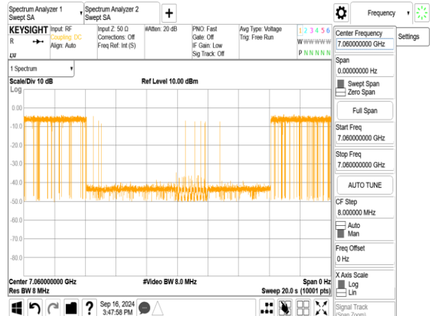
802.11be_320MHz_CF 6905MHz_Interference_7060MHz_-81.55dBm_ON
