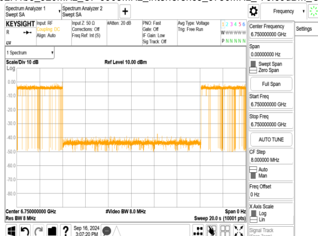
802.11be_320MHz_CF 6905MHz_Interference_6750MHz_-77.69dBm_Minimal
