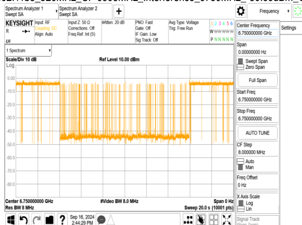
802.11be_320MHz_CF 6905MHz_Interference_6750MHz_-80.69dBm_ON
